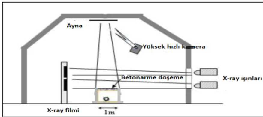
Şekil 1.2. Deney düzeneği
