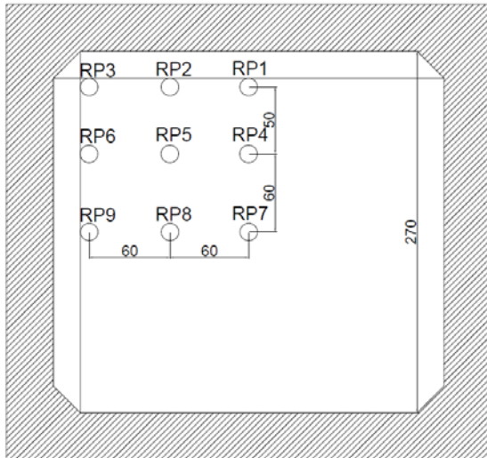
Şekil 1.5. Basınç ölçüm cihazlarının yerleşimi, yükseklik kesiti
