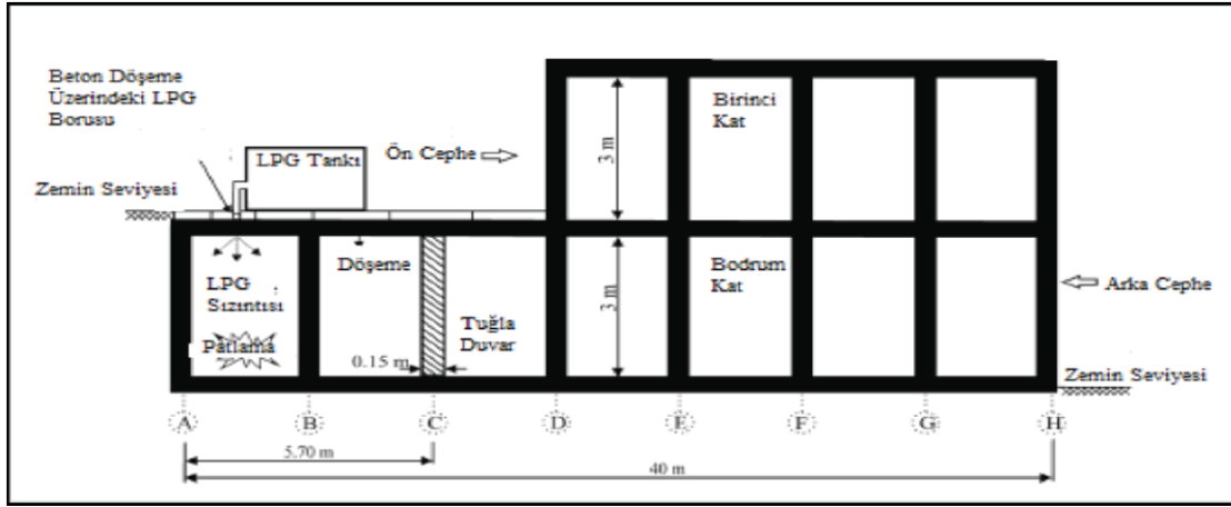
Şekil 1.10. Yapının kesiti
