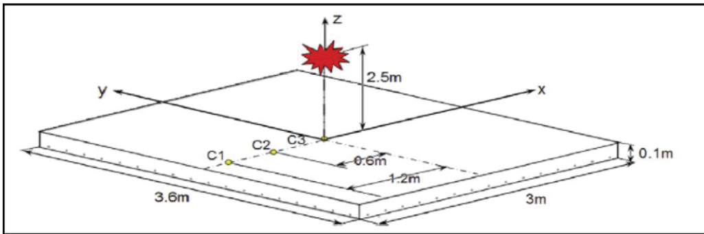
Şekil 1.7. Betonarme döşemenin geometrik biçimi
