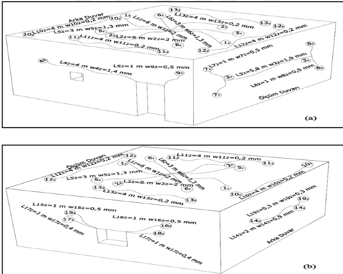
Şekil 3.6. Betonarme odadaki çatlak kroki (İkinci patlama) (a) Ön görünüş (b) Arka görünüş
