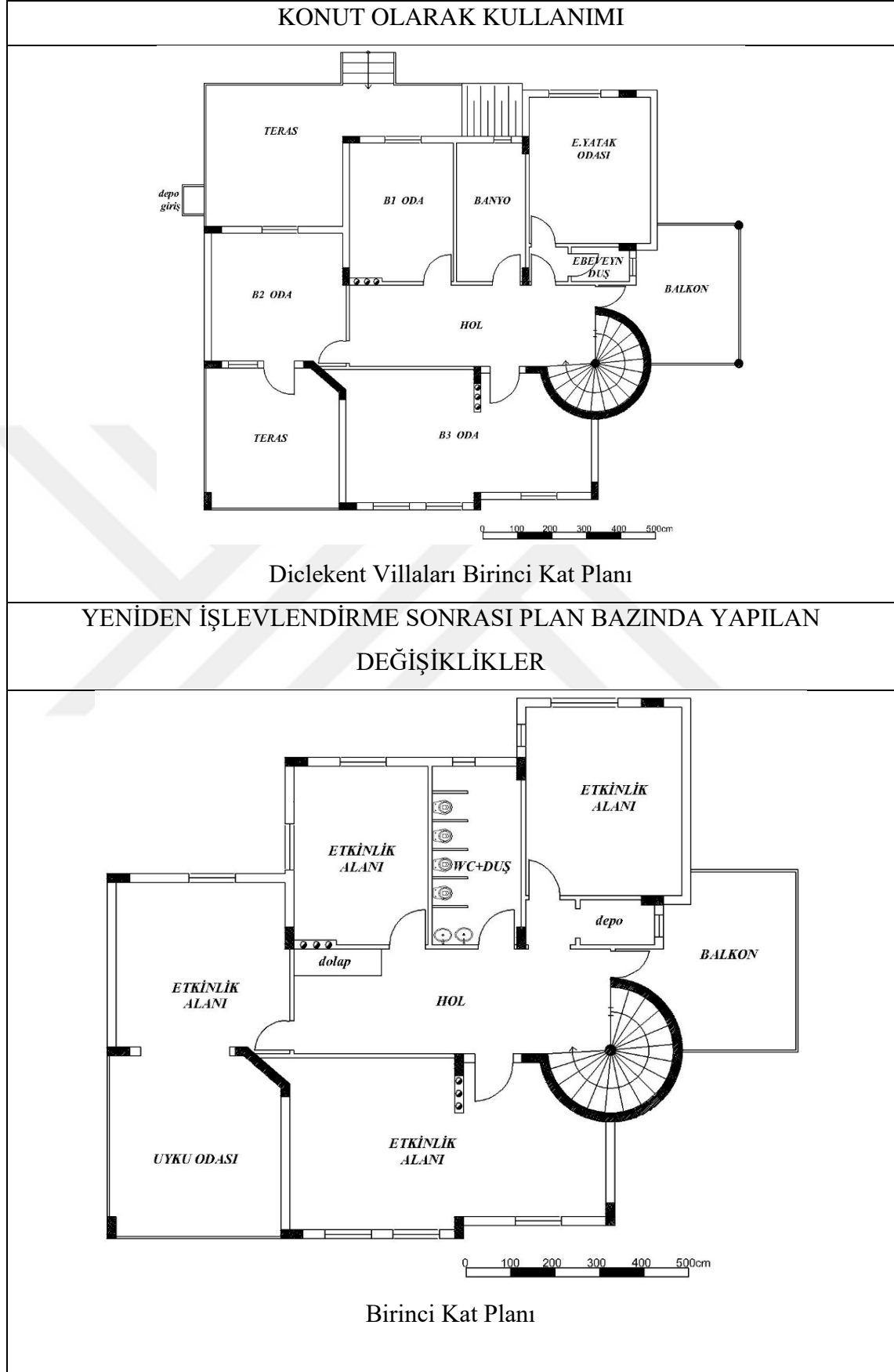
Çizelge 4.25. 2093 ada 6 parselde yer alan yapının birinci kat planındaki değişimler
