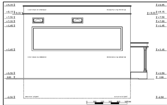
Şekil 4.55. Gönül Kahvesinin sol yan görünüşü
