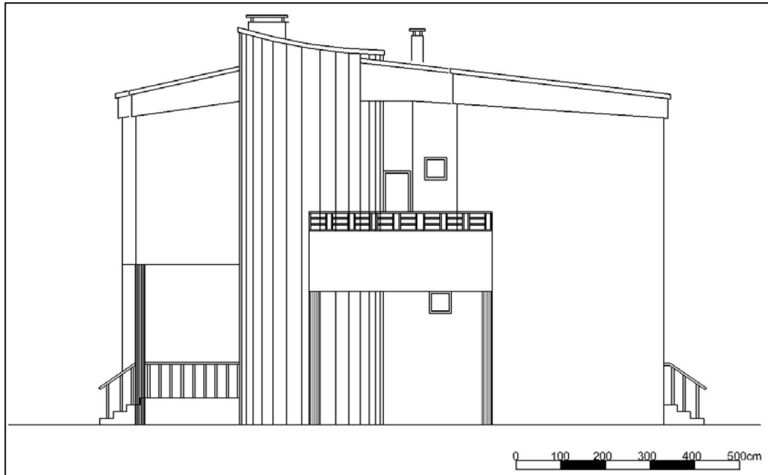
Şekil 4.7. Villa sağ yan cephe
