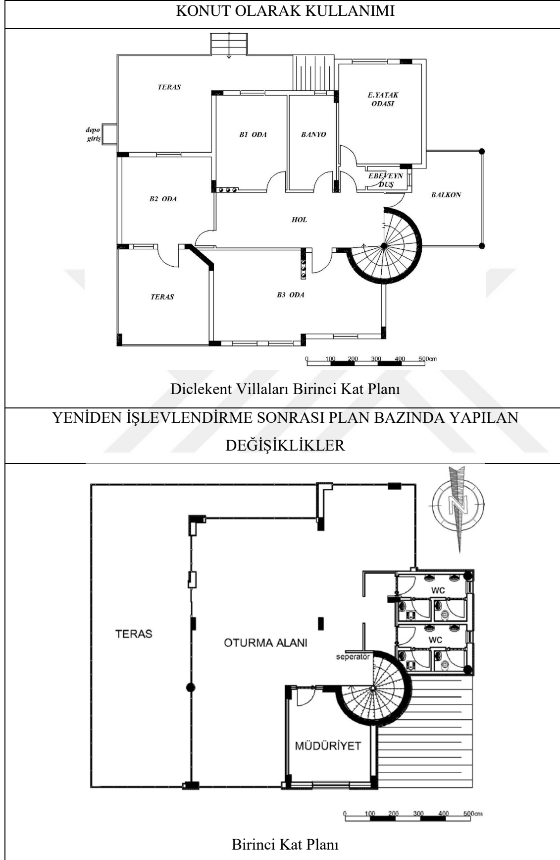
Çizelge 4.7. 2097 ada 1 parselde yer alan yapının birinci kat planındaki değişimler
