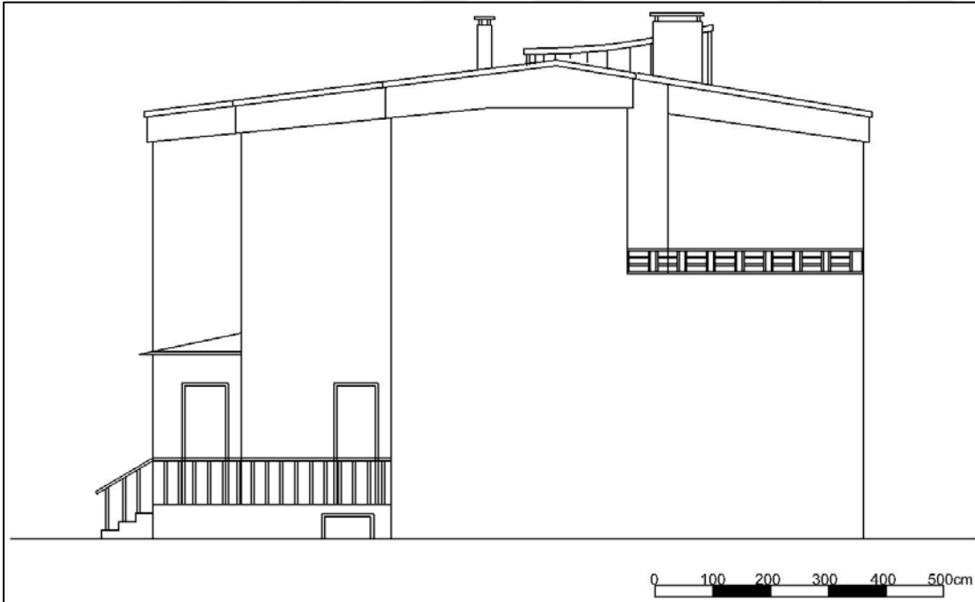
Şekil 4.9. Villa sol yan cephe
