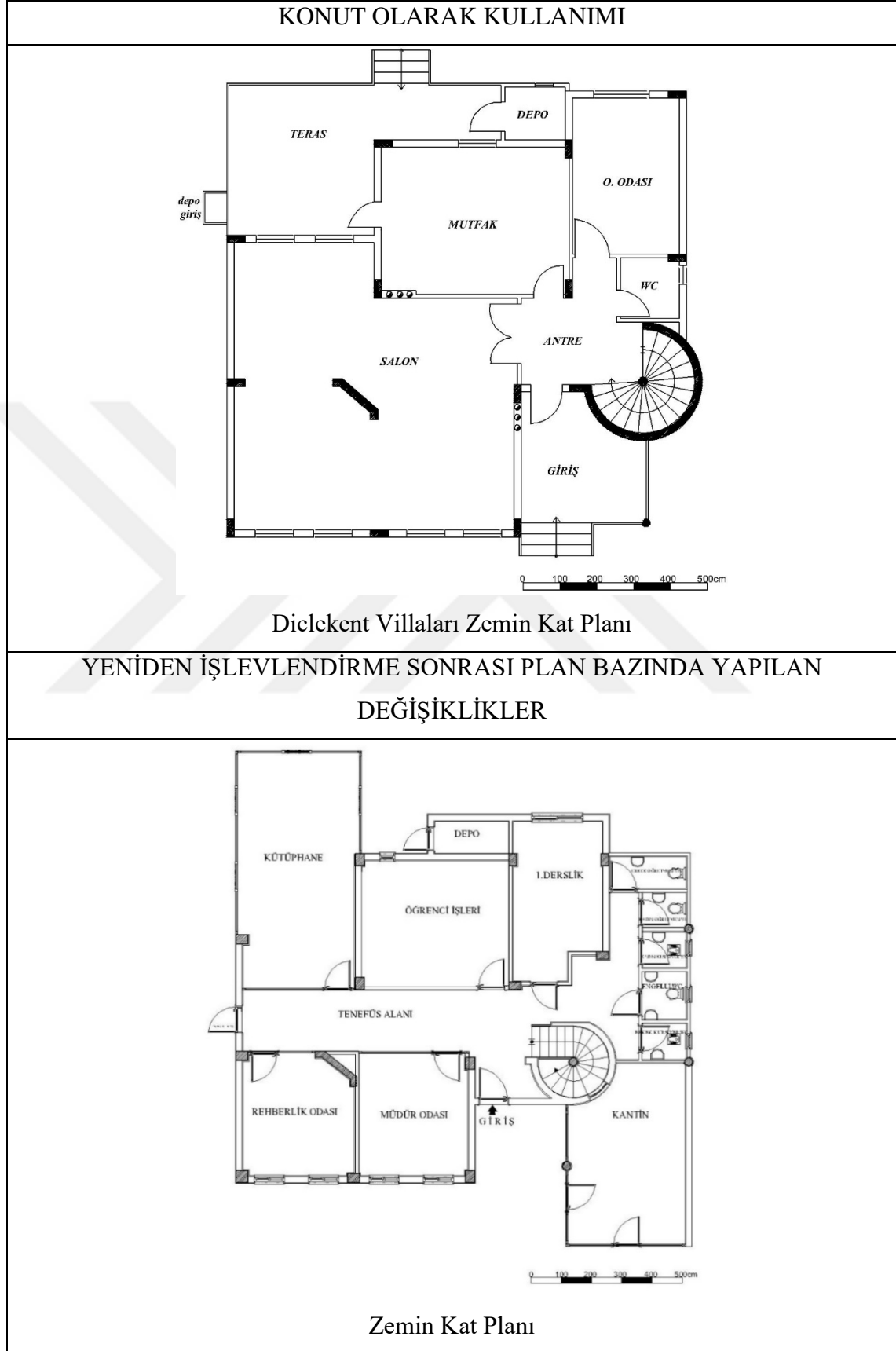
Çizelge 4.21. 2104 ada 5 parselde yer alan yapının zemin kat planındaki değişimler
