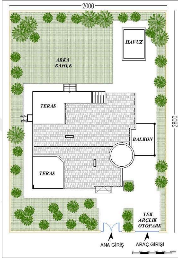
Şekil 4.5. Diclekent Villaları vaziyet planı
