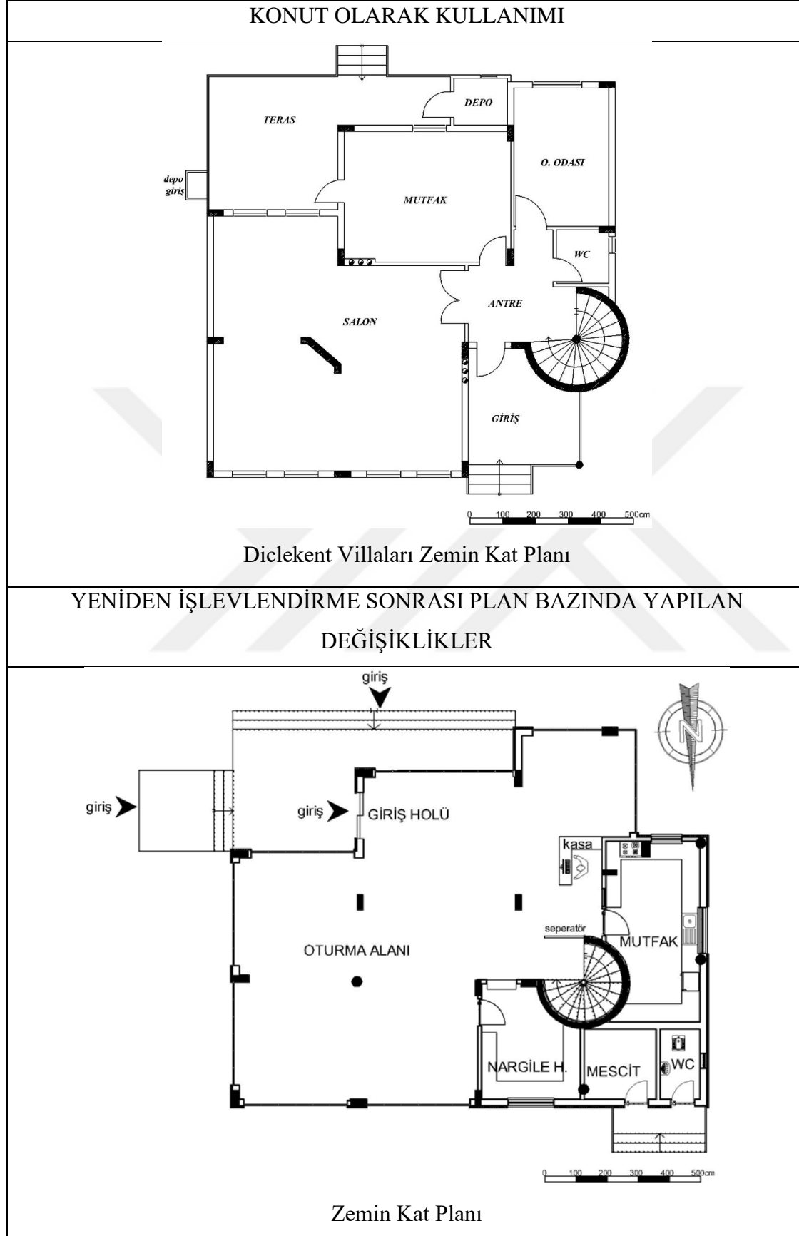
Çizelge 4.6. 2097 ada 1 parselde yer alan yapının zemin kat planındaki değişimler
