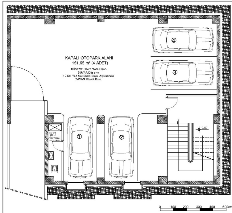
Şekil 4.48. Gönül Kahvesi bodrum kat planı
