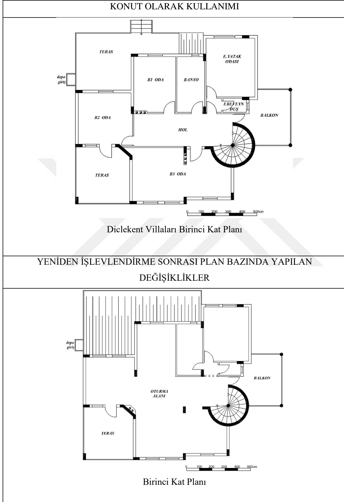
Çizelge 4.10. 418 ada 9 parselde yer alan yapının birinci kat planındaki değişimler
