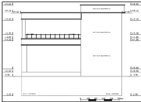
Şekil 4.54. Gönül Kahvesinin arka görünüşü
