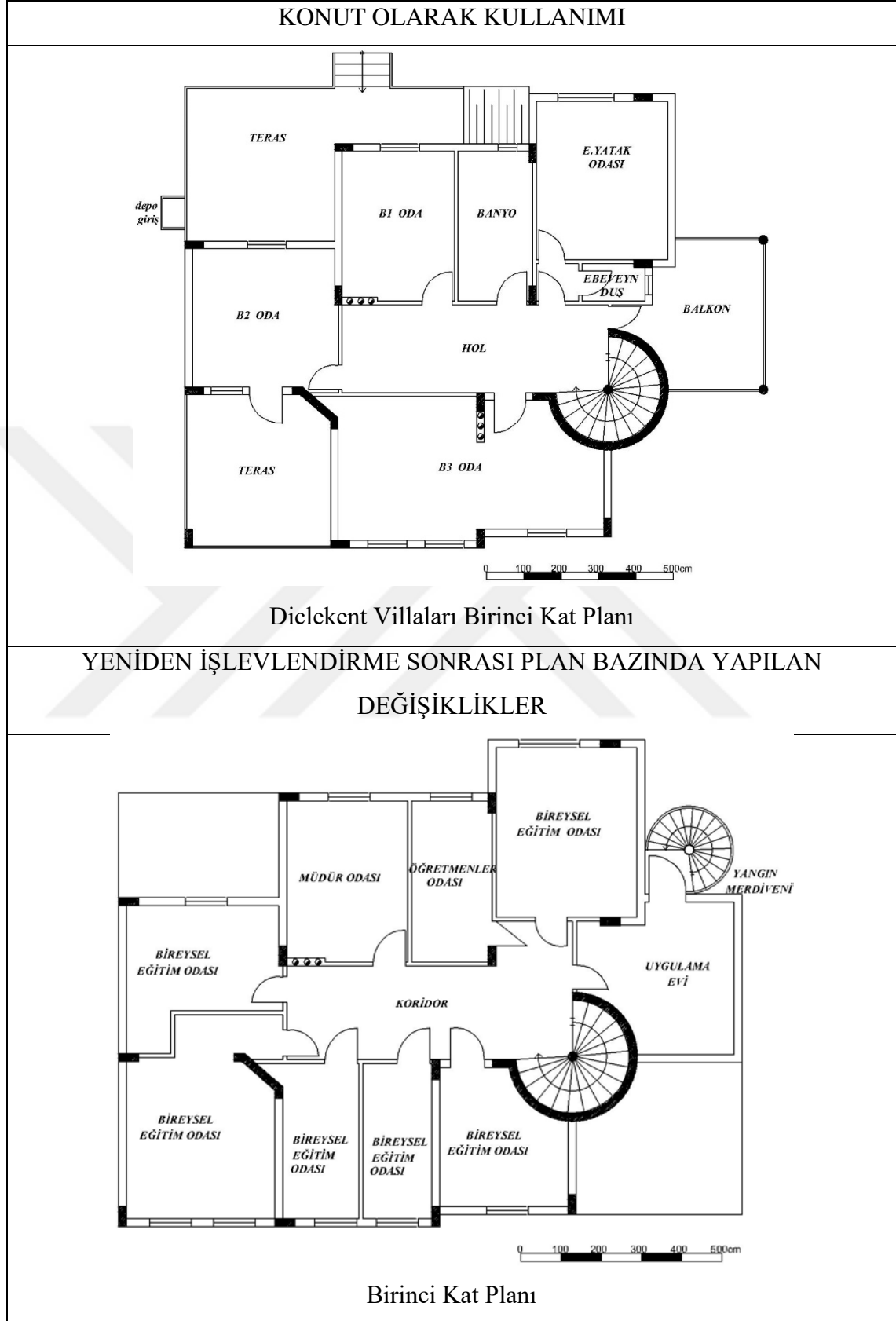
Çizelge 4.19. 2099 ada 3 parselde yer alan yapının birinci kat planındaki değişimler
