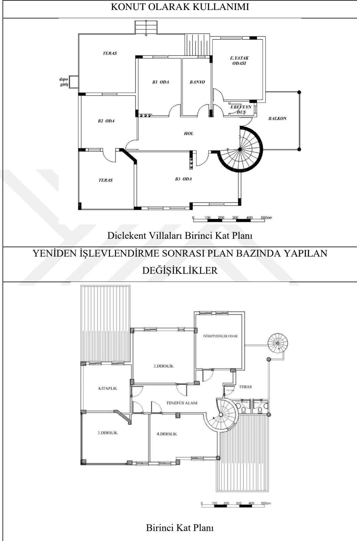
Çizelge 4.22. 2104 ada 5 parselde yer alan yapının birinci kat planındaki değişimler
