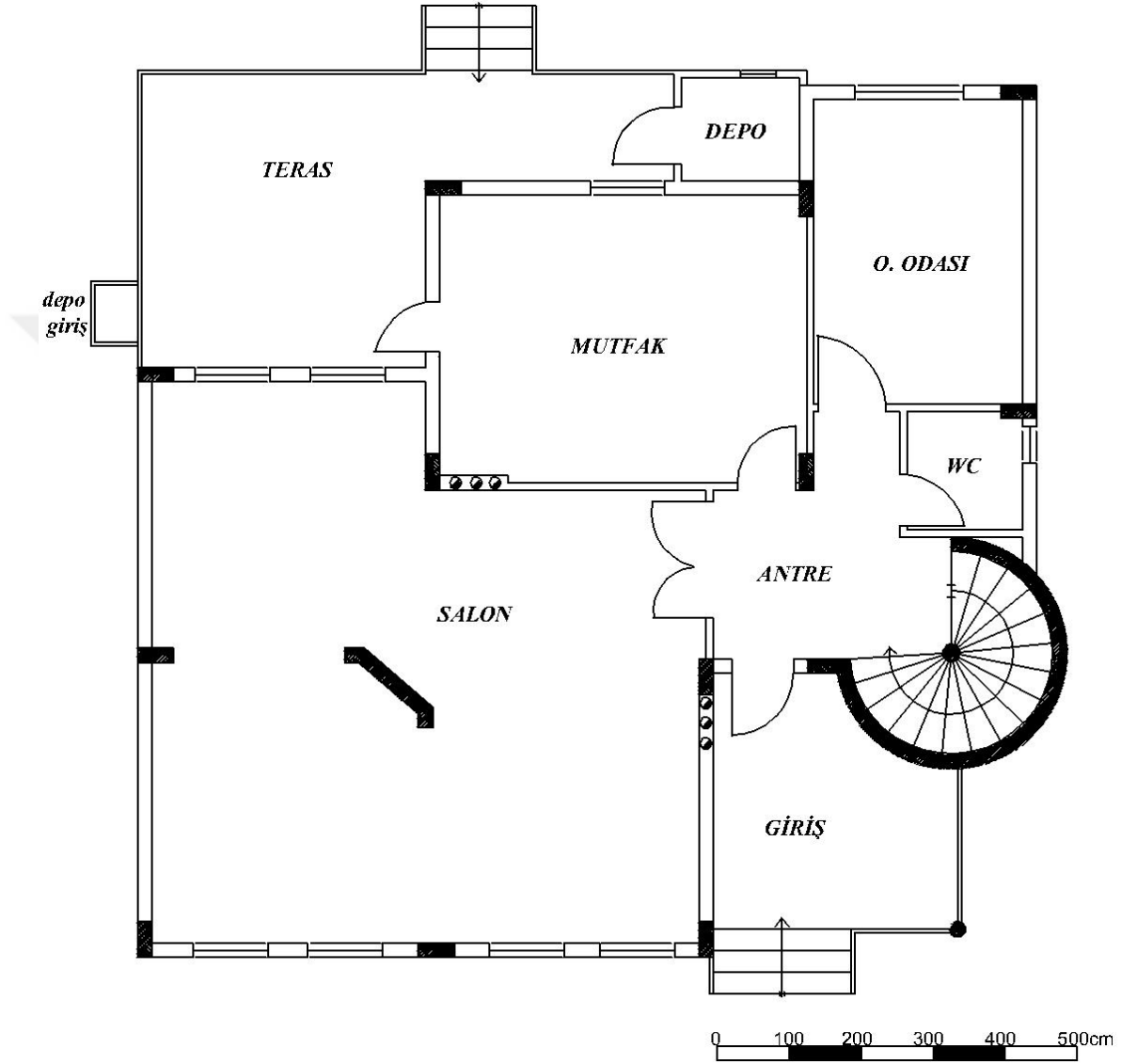
Şekil 4.10. Diclekent Villaları zemin kat planı
