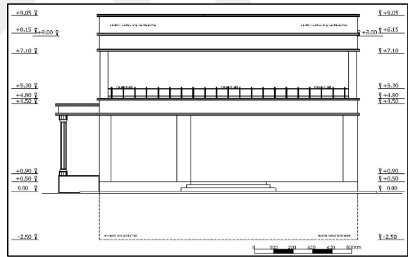
Şekil 4.53. Gönül Kahvesinin sağ yan görünüşü
