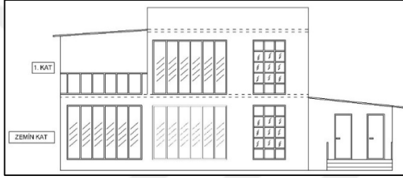
Şekil 4.38. Kafenin arka görünüşü
