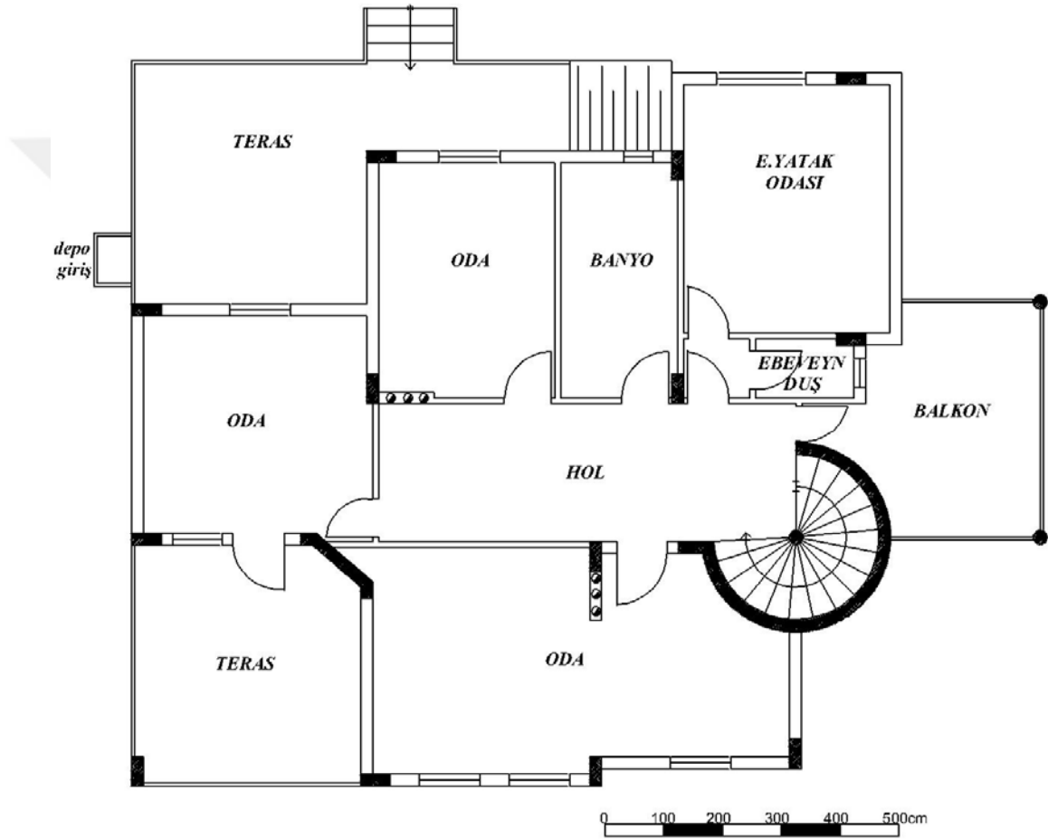
Şekil 4.13. Diclekent Villaları birinci kat planı
