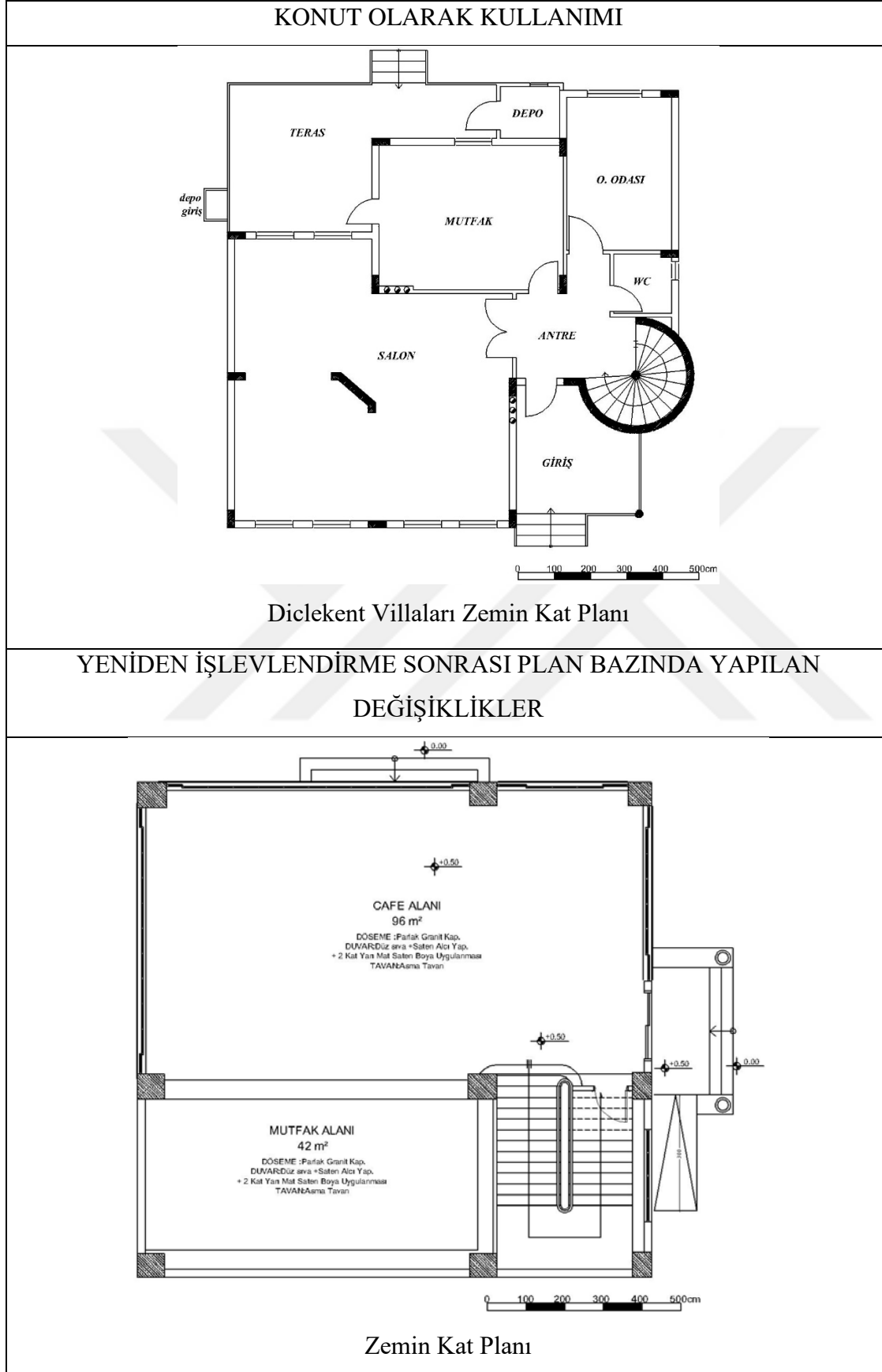
Çizelge 4.12. 2108 ada 5 parselde yer alan yapının zemin kat planındaki değişimler
