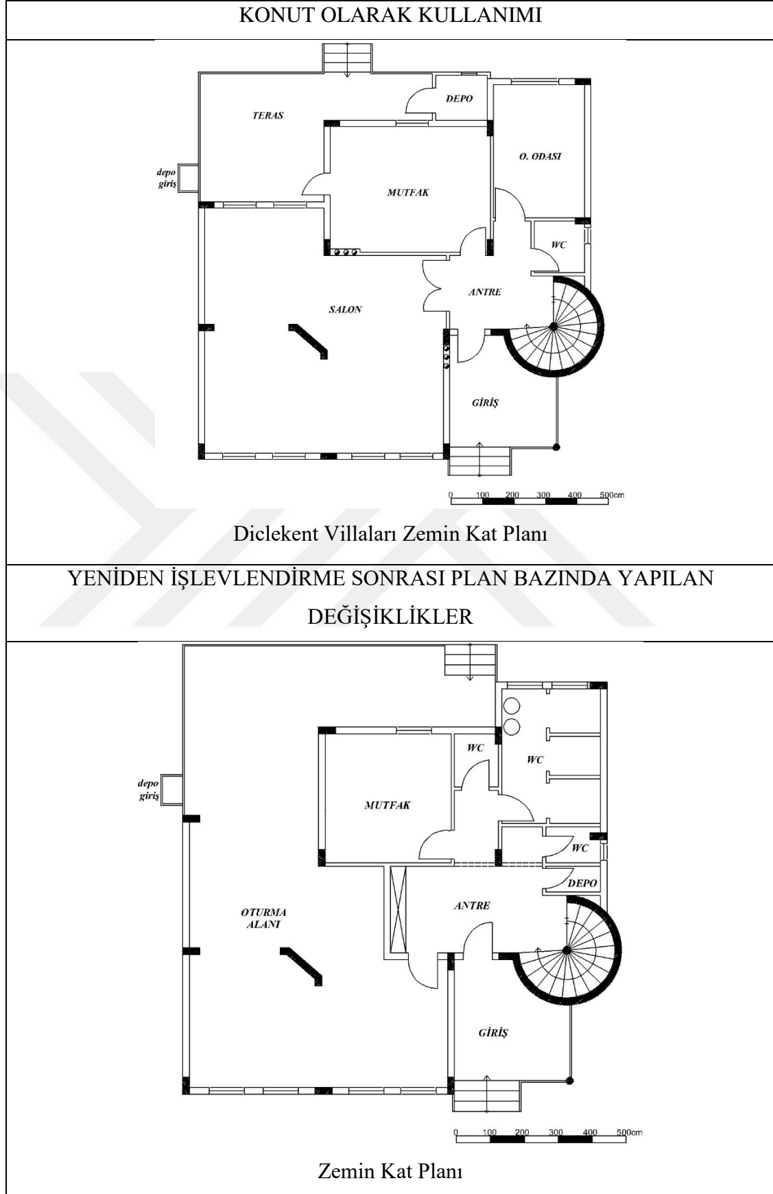
Çizelge 4.9. 418 ada 9 parselde yer alan yapının zemin kat planındaki değişimler
