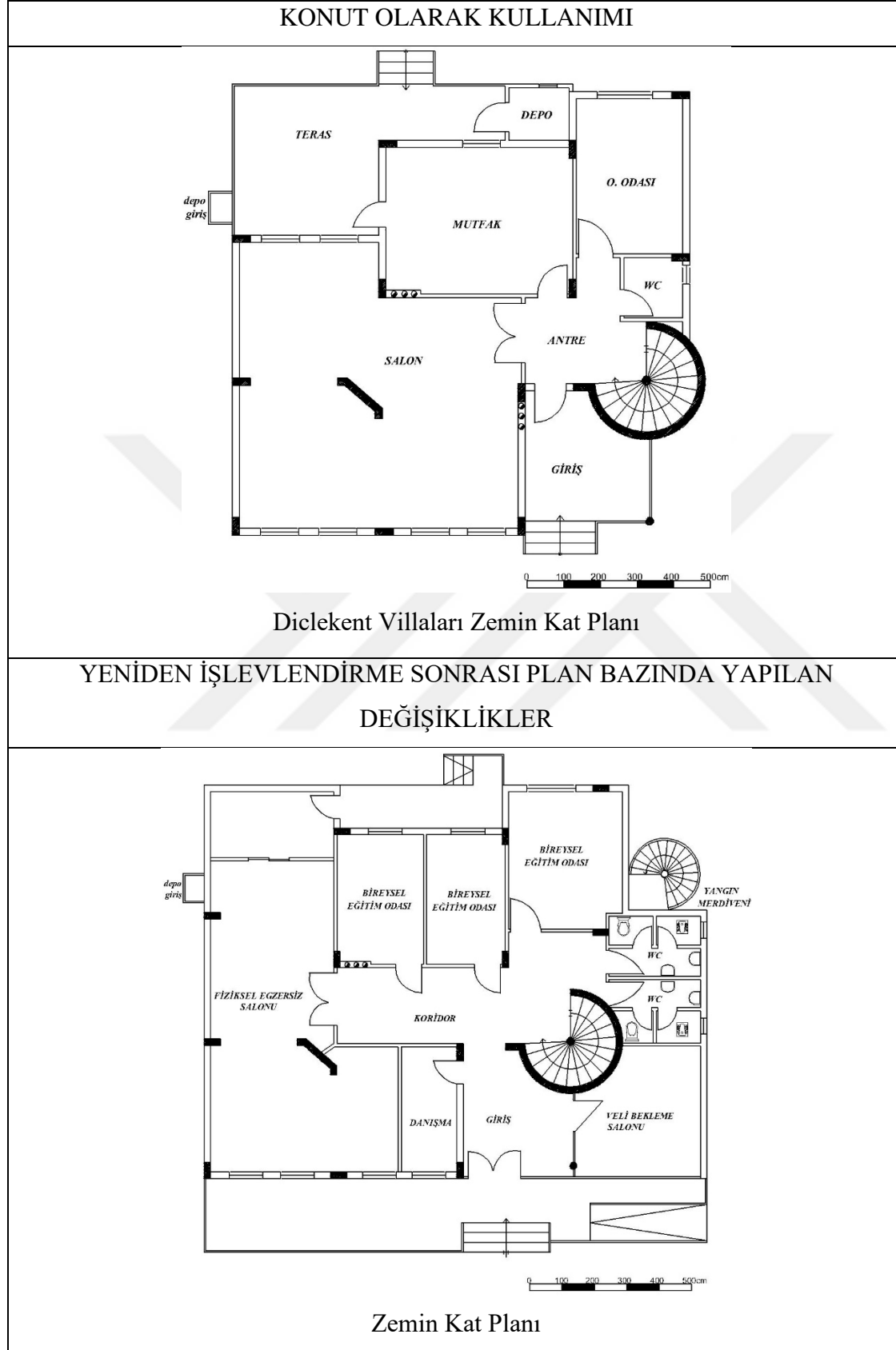
Çizelge 4.18. 2099 ada 3 parselde yer alan yapının zemin kat planındaki değişimler
