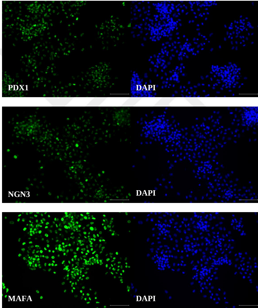
Şekil.1A. Ad-NPM virüsünün sırasıyla Anti-Pdx1, Anti-Ngn3, Anti-MafA (yeşil) ve DAPI (mavi) immünoboyama sonuçları. Cetvel 100µm'dir.
