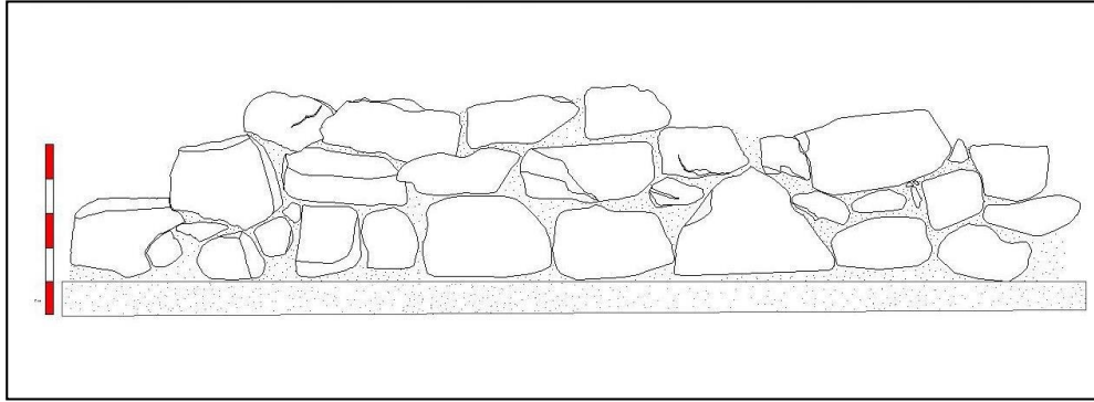
Çizim 2. Mekan 13' ün Dış Kısımının Bir Bölümünün Görünümü.
