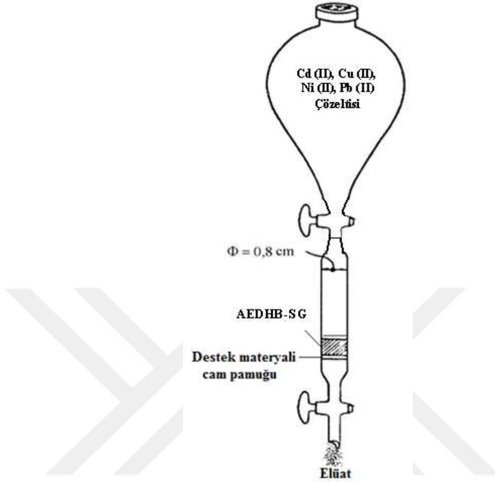
Şekil 3.3. Zenginleştirme çalışmaları için kullanılan kolon düzeneği
