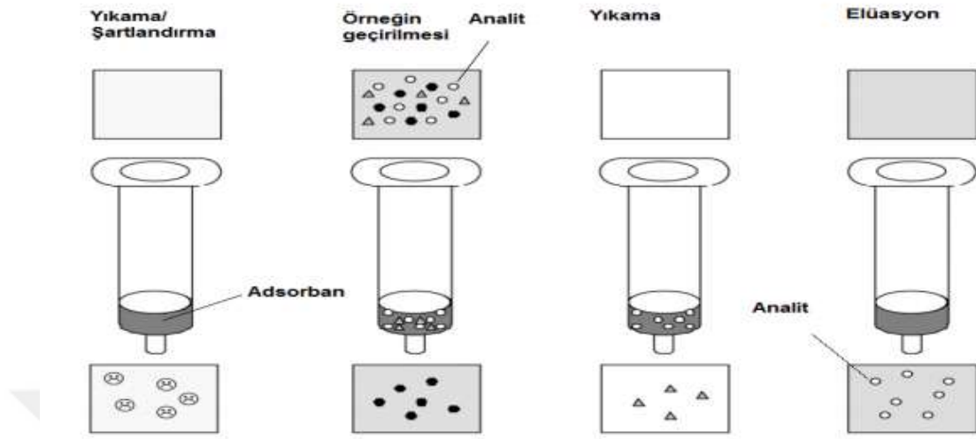
Şekil 2.1. Katı faz ekstraksiyonu metodunun basamakları [42].
