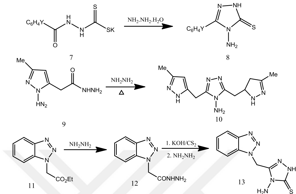
Şekil 2.2. Hidrazin türevlerini kullanarak sentezi [2]
