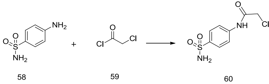
Şekil 3.8. 4-amino benzenesülfonilamit açılması [19]
