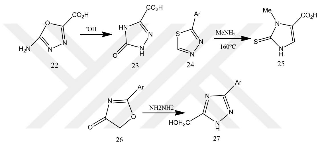
Şekil 2.5. Diğer heterosiklik sistemlerin dönüşümü yoluyla triazollerin sentezi [5]
