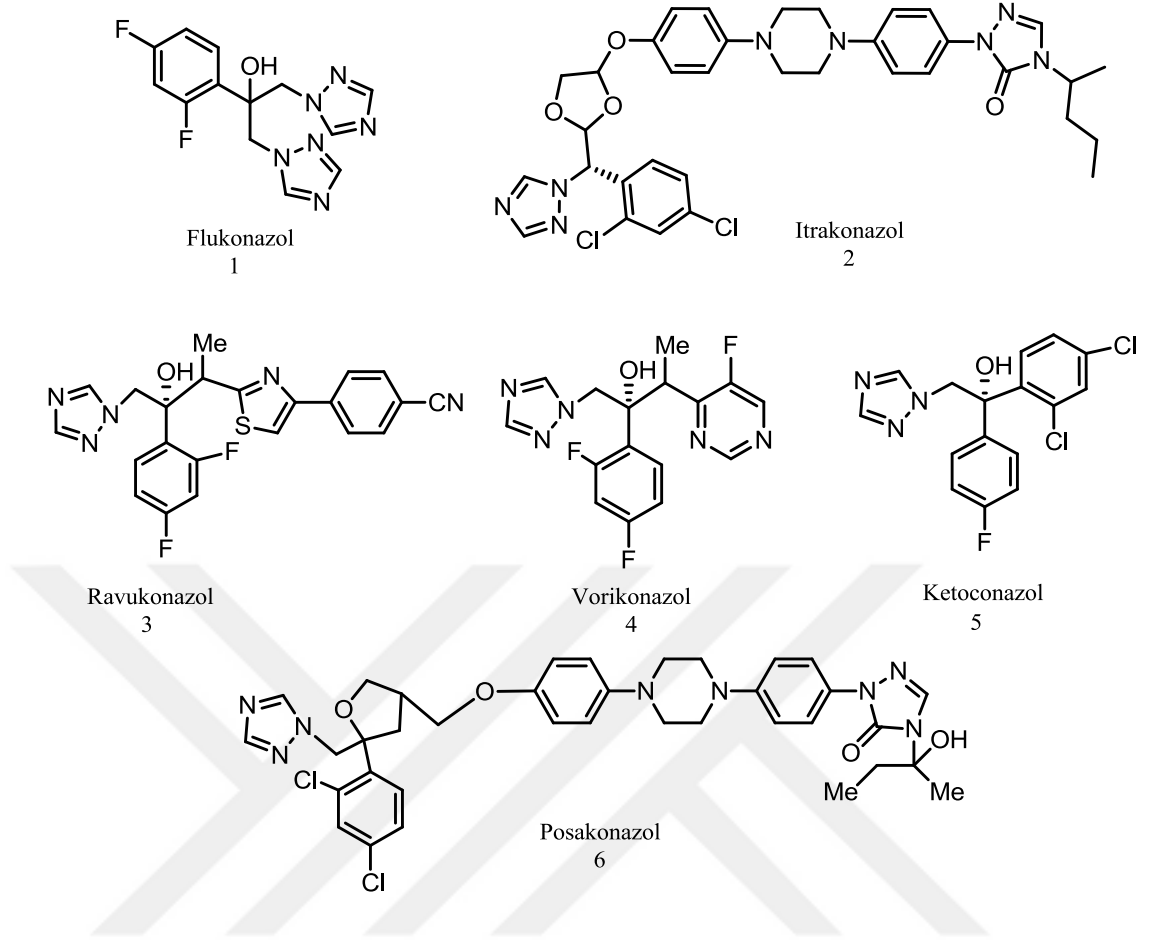
Şekil 2.1. Triazol Yapısı [1]
