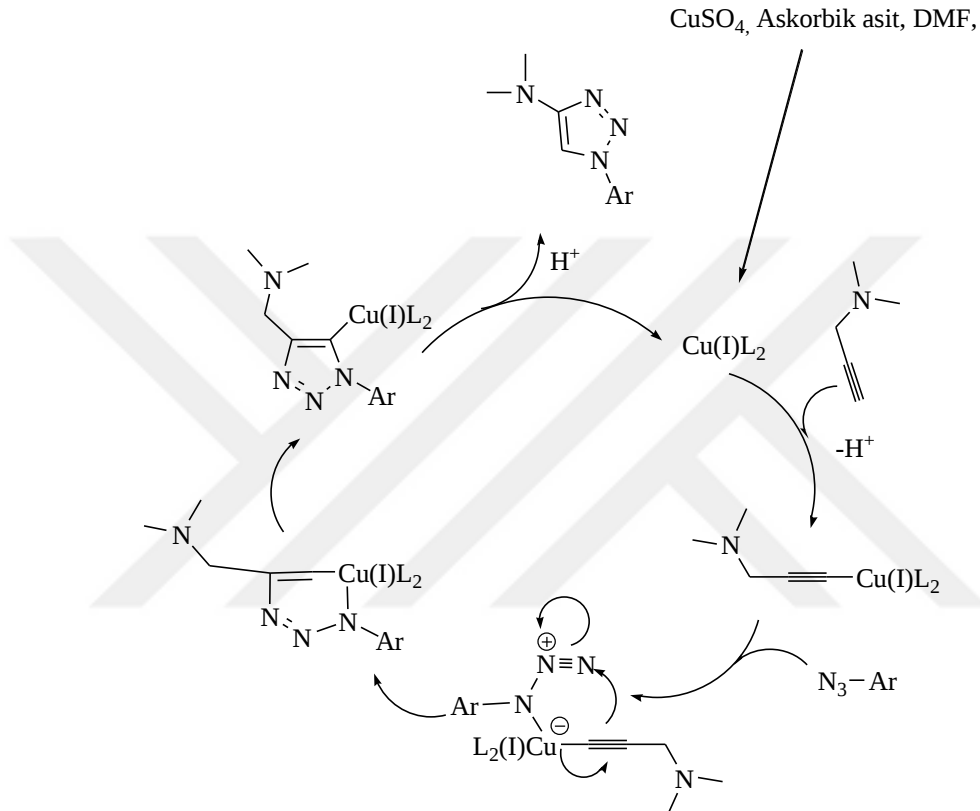
Şekil 6.1. 1,3-dipolar siklo katılma sonucu oluşan D1 molekülü için önerilen mekanizma [27].
