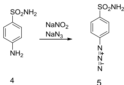
Şekil 4.1. Azidosülfonamit sentezi [28]
