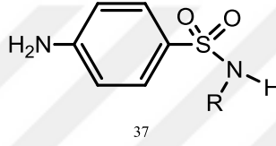
Şekil 3.1. Sülfonilamitlerin genel yapısı [12]
