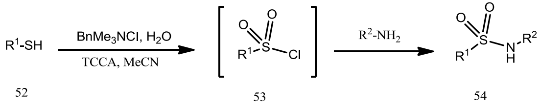
Şekil 3.6. Bonk sülfonilamit sentezi[17]
