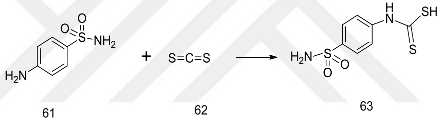
Şekil 3.9. 4-amino benzenesülfonilamit'in karbondisülfür reaksiyonu [20]
