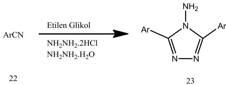
Şekil 2.6. Mikrodalga ışınlaması altında 1,2,4-triazollerin sentezi [6]
