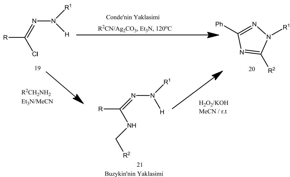
Şekil 2.4. Nitril iminler ve triazinler kullanarak sentezi [4]
