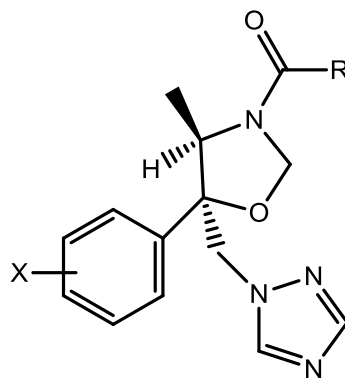
Şekil 2.8 4 (R), 5 (R) içeren triazol [8]
