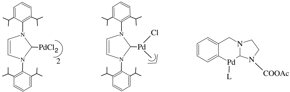
Şekil 2.8. Suzuki-Miyaura çapraz eşleşme reaksiyonlarında kullanılan paladosiklikler
