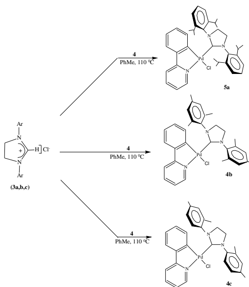
Şekil 4.3. Sentezlenen paladosiklik kompleksler
