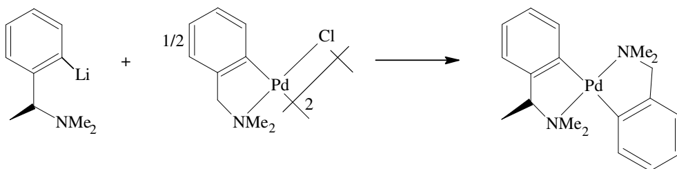
Şekil 2.30. Transmetalasyon reaksiyonu ile bis-siklopaladat bileşiklerinin sentezi
