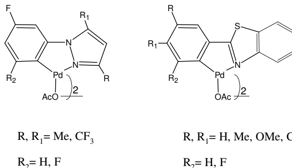
Şekil 2.20. 1-Arilpirazol veya 2-arilbenzotiyazollerden türeyen paladosiklikler
