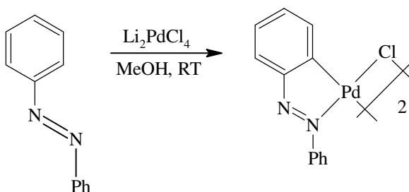
Şekil 1.1. Azobenzenin siklopaladasyonu
