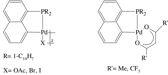
Şekil 2.11. tri- \alpha -naftalilfosfine dayanan farklı yapılardaki fosfin yapılı paladosiklikler
