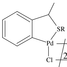
Şekil 2.21. SC-Paladosiklik kompleks
