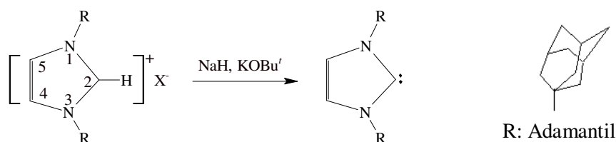
Şekil 2.1. İlk serbest kararlı NHC sentezi
