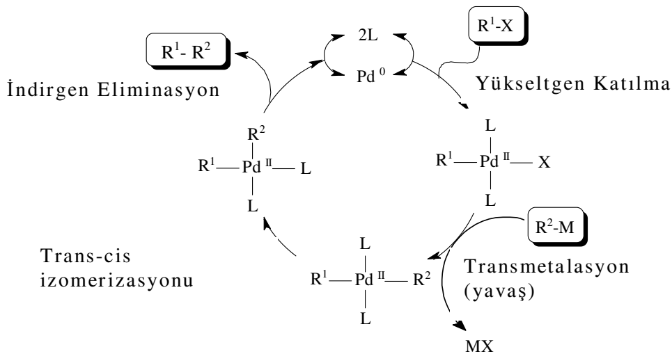
řekil 2.34. Suzuki-Miyaura apraz eřleřme reaksiyonunun genel mekanizması
