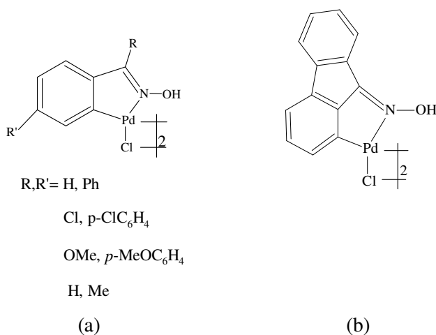
Şekil 2.17. Oksim türevli paladosiklikler
