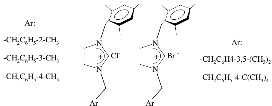
Şekil 1.6. 1,3-dialkilimidazolyum tuzları
