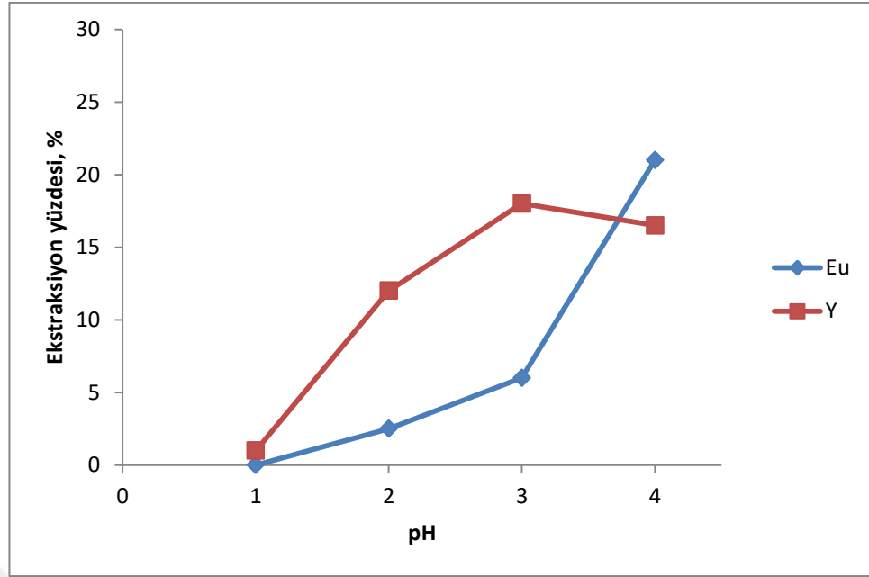
Şekil 9.7. Farklı pH'larda hazırlanan kırmızı fosfor besleme çözeltilerinin 0,02 M [MAL][NTf 2 ] ile ekstraksiyonu sonucunda elde edilen ekstraksiyon yüzdesleri.
