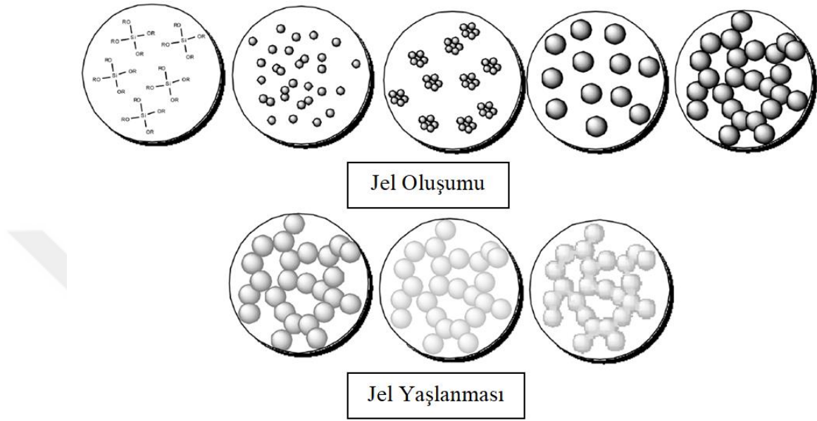
Şekil 6.1. Sol-jel prosesi (silikon alkoksit öncü ile), jel oluşumu ve yaşlanması (Marr ve Marr, 2016).
