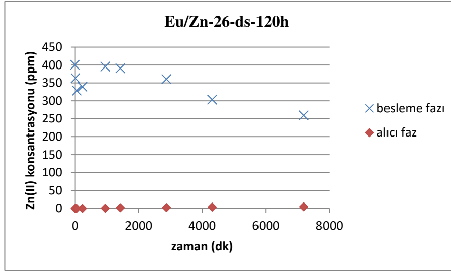
Şekil 9.28. Alıcı faz distile su olduğu durumda Eu/Zn karışımının membran sistem boyunca geçişinde fazların zamana bağlı (a) Eu(III) ve (b) Zn(II) konsantrasyonu değişimi.
