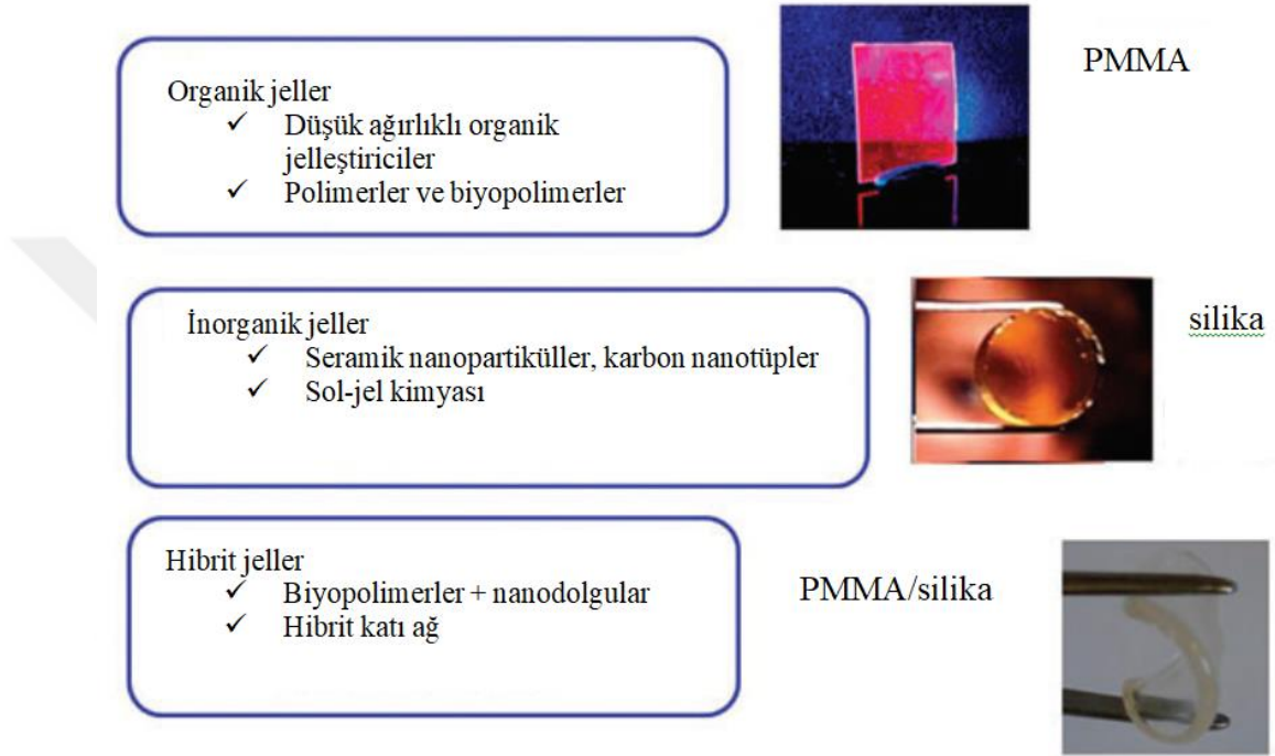
Şekil 6.5. Farklı türlerde iyonojeller (Le Bideau, vd., 2011).
