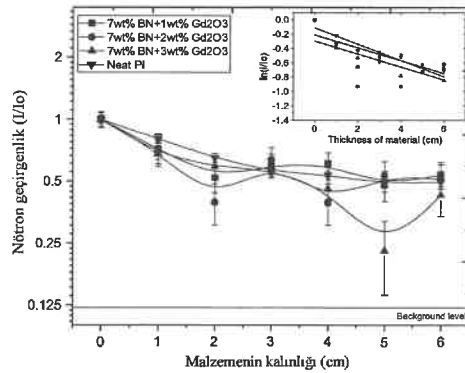
Şekil 4.51. %7 BN katkılı örneklerin katkılanan Gd_2O_3 miktarına bağlı nötron soğurma eğrileri
