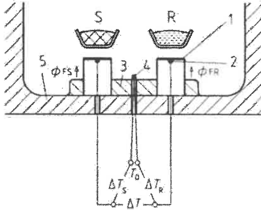
Şekil 3.7. DSC hücresinin kesit alanı; 1- Örnek ve referans örnek için yükseltilmiş platform; 2- Kromel ısı eleman (thermocouple); 3- Bakır ve nikel alaşımından (konstantan) oluşan gövde, 4- Kromel-konstantan ısı eleman; 5-Gümüş fırın
