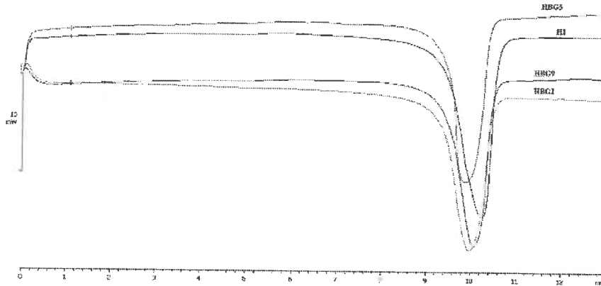
Şekil 4.30. Saf YYPE ve seçilmiş kompozitlerin DSC termogramları
