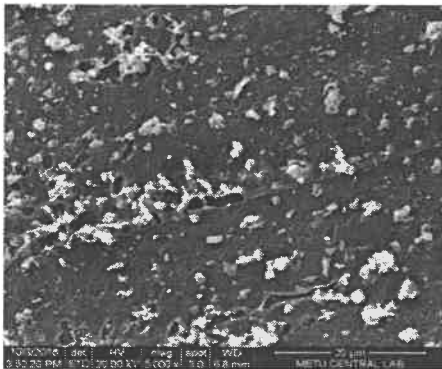
Şekil 4.15. %11 B_4C /%3 Gd_2O_3 /%86 PI kompozitlerinin SEM fotoğrafları
