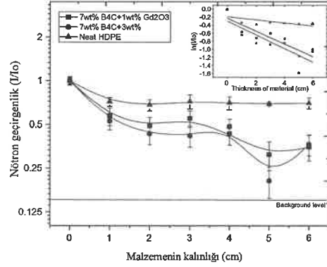
Şekil 4.44. %7 B 4 C katkılı örneklerin katkılanan Gd 2 O 3 miktarına bağlı nötron soğurma eğrileri
