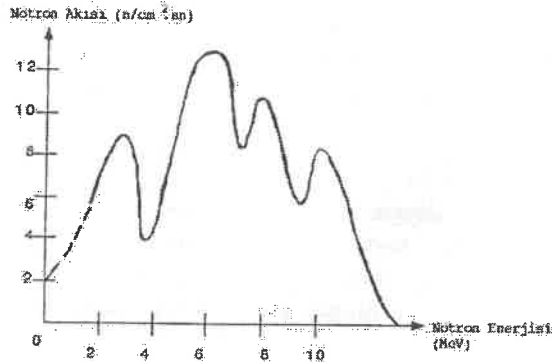
Şekil 3.10 . Nötron Howitzer-3 kaynağının nötron enerjisi-nötron akısı dağılımı (Yiğit 1996).
