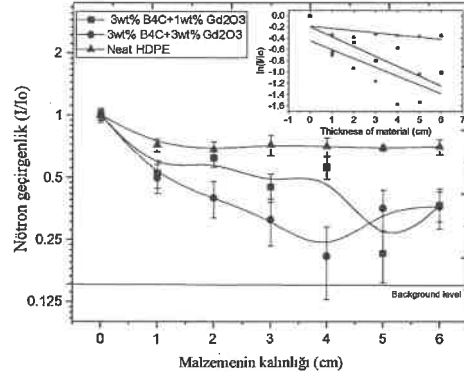
Şekil 4.43. %3 B 4 C katkılı örneklerin katkılanan Gd 2 O 3 miktarına bağlı nötron soğurma eğrileri
