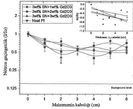
Şekil 4.50. %3 BN katkılı örneklerin katkılanan Gd_2O_3 miktarına bağlı nötron soğurma eğrileri
