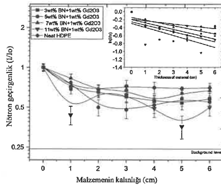
Şekil 4.33. (%3-11 h-BN/%1 Gd 2 O 3 )/YYPE nano kompozitlerin nötron soğurma grafiği
