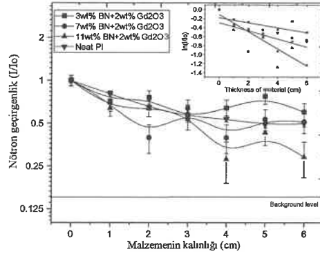
Şekil 4.48. (%3-%7-%11BN+%2 Gd_2O_3 )/PI nano kompozitlerin nötron geçirgenlik eğrileri
