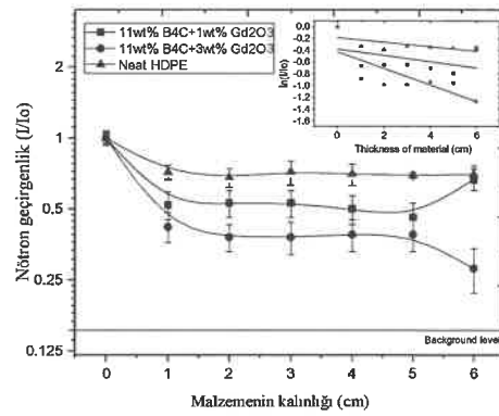
Şekil 4.45. %11 B 4 C katkılı örneklerin katkılanan Gd 2 O 3 miktarına bağlı nötron soğurma eğrileri
