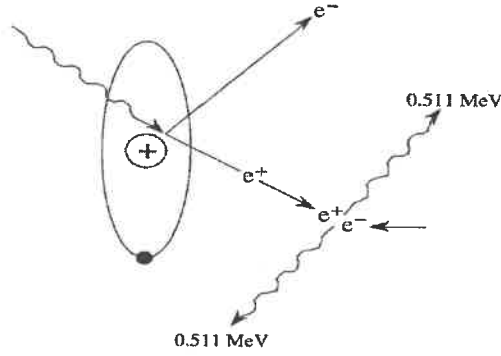
Şekil 2.4. Çift oluşum (Martin 2013)
