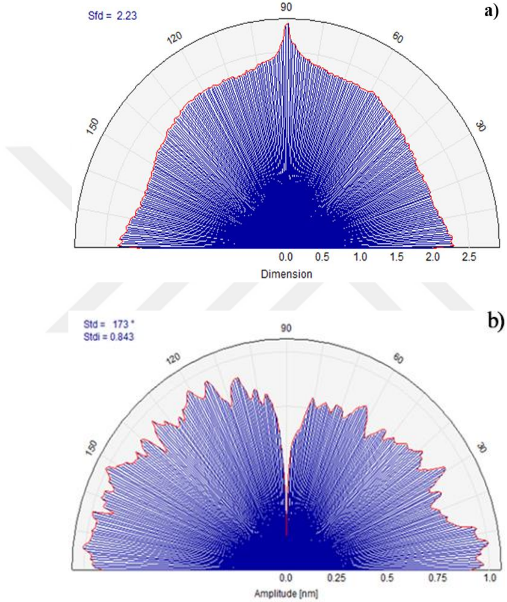
Şekil 4.8. VN4-13-Si2.000 isimli numunenin SPIP görüntüleri: a) Sfd (alt ekseninde boyut), b) StdI (alt ekseninde genlik)
