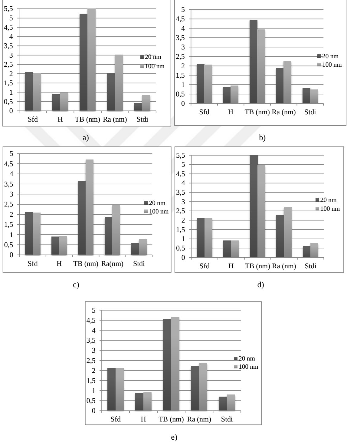
Şekil 5.8. Si/SiO 2 /Si 3 N 4 alttaşı üzerine büyütülmüş 20 nm ve 100 nm kalınlıklı filmlerin aynı gaz oranlarında karşılaştırılması: a) %5 gaz oranı, b) %10 gaz oranı, c) %15 gaz oranı, d) %20 gaz oranı, e) %30 gaz oranı
