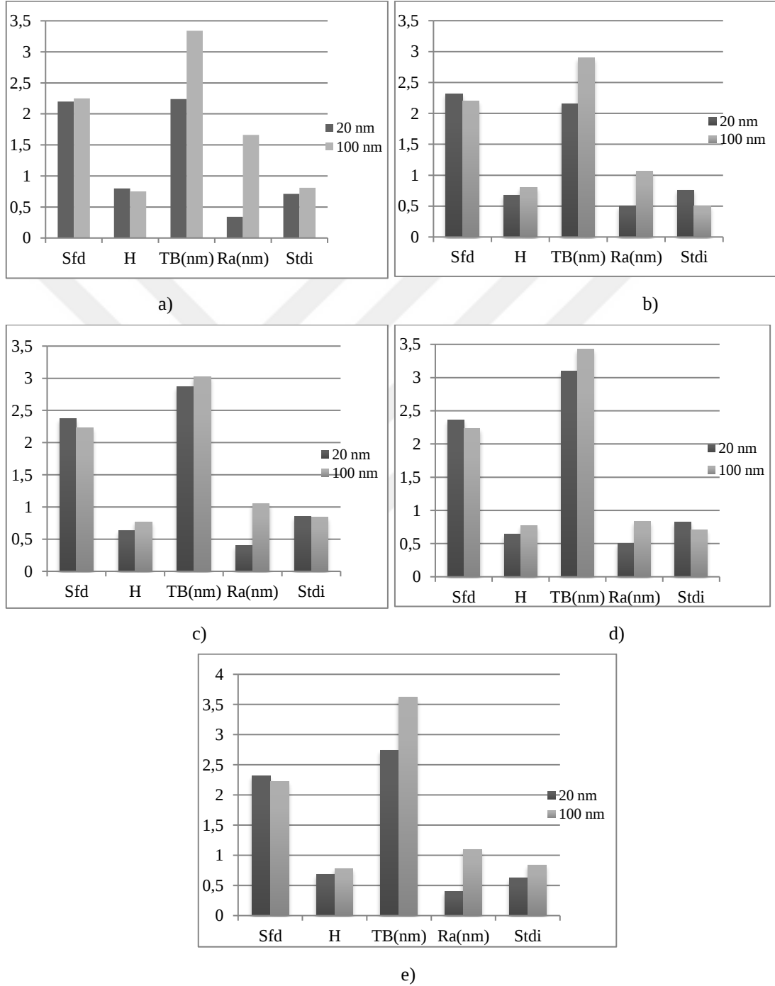
řekil 5.7. Si/SiO 2 alttař üzerine büyütmüş 20 nm ve 100 nm kalınlıklı filmlerin aynı gaz oranlarında karřılařtırılması: a) %5 gaz oranı, b) %10 gaz oranı, c) %15 gaz oranı, d) %20 gaz oranı, e) %30 gaz oranı
