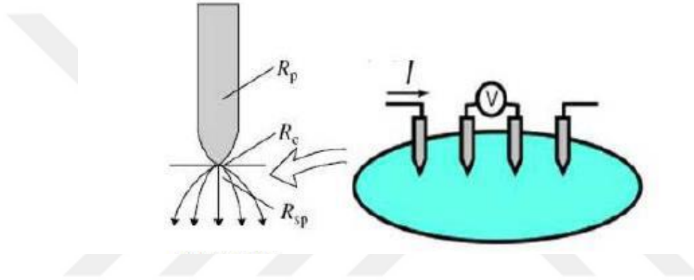
Şekil 3.1. FPP tekniğinin şematik gösterimi [36]
