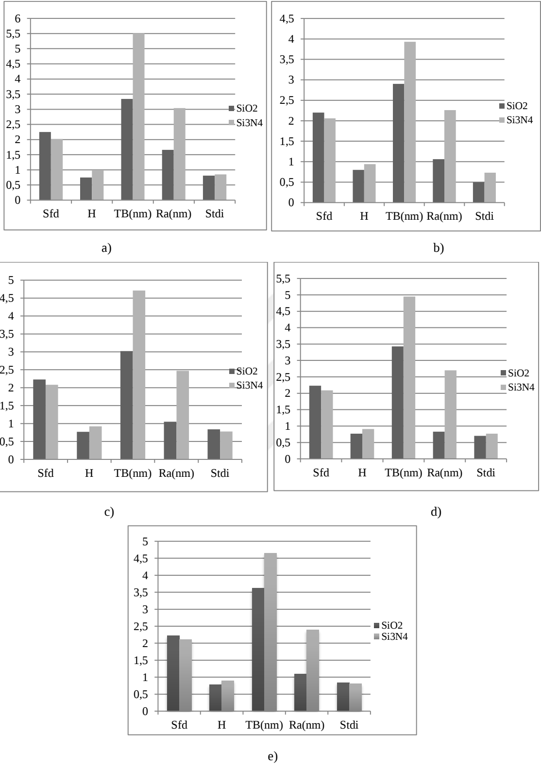
Şekil 5.6. Si/SiO 2 ve Si/SiO 2 /Si 3 N 4 alttaş üzerine büyütülmüş 100 nm kalınlıklı filmlerin aynı gaz oranlarının karşılaştırılması: a) %5 gaz oranı, b) %10 gaz oranı, c) %15 gaz oranı, d) %20 gaz oranı, e) %30 gaz oranı
