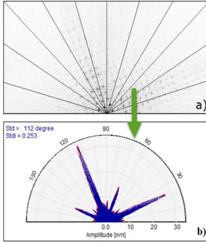
Şekil 3.2. Fourier spektrumu ve açısal spektrum. Şekil b)'de gösterilen açının hesaplanması için kullanılan eşit hatlar Şekil a)'da verilmiştir [44]
