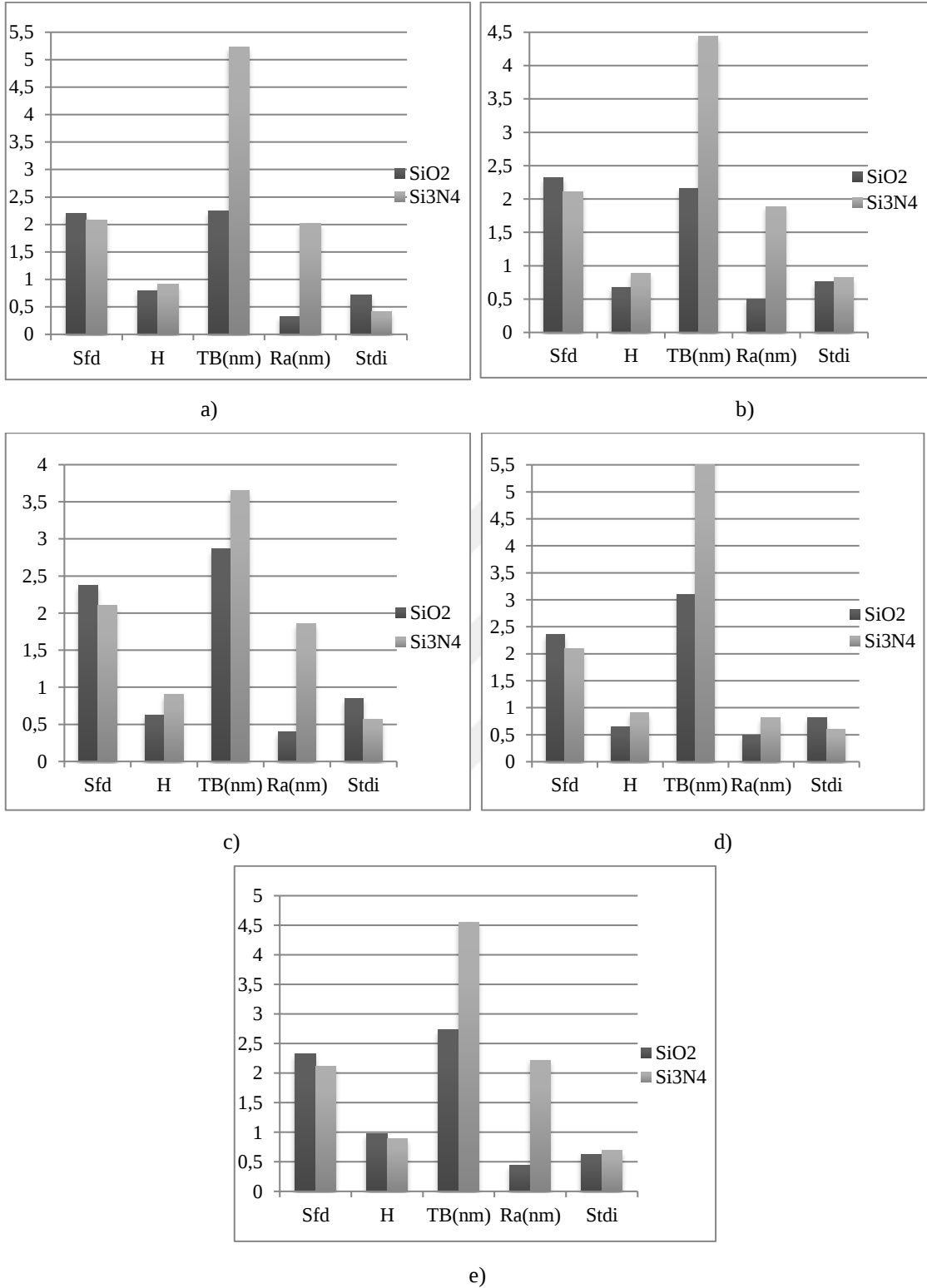
Şekil 5.5. Si/SiO 2 ve Si/SiO 2 /Si 3 N 4 alttaş üzerine büyütülmüş 20 nm kalınlıklı filmlerin aynı gaz oranlarının karşılaştırılması: a) %5 gaz oranı, b) %10 gaz oranı, c) %15 gaz oranı, d) %20 gaz oranı, e) %30 gaz oranı
