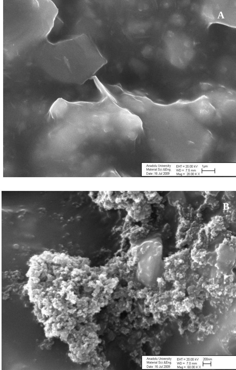
Şekil 5.21. Referans boya (a), ağırlıkça %5 T-Boya (b)
