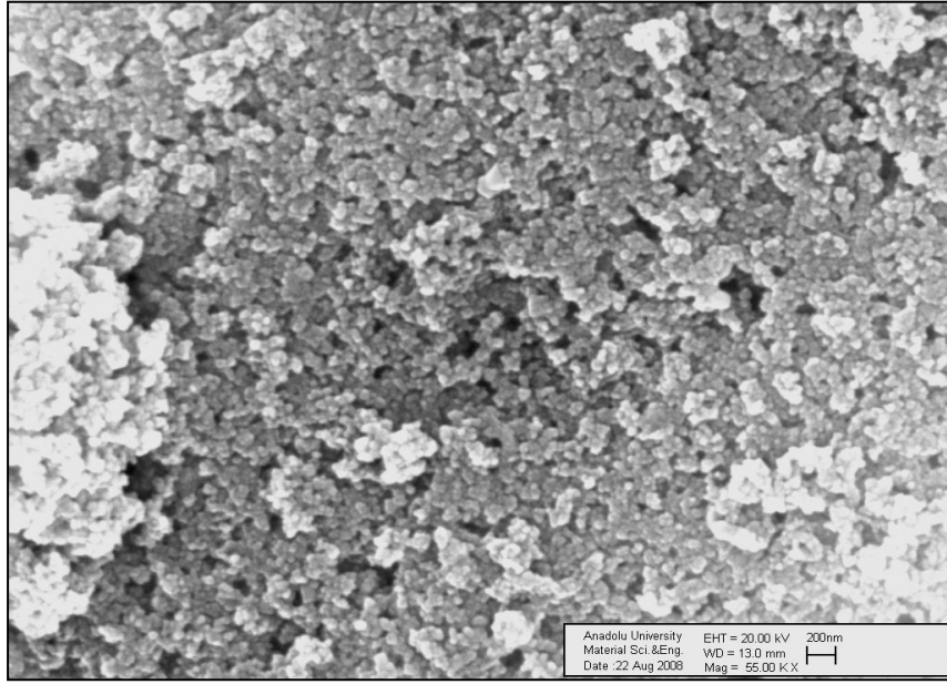
Şekil 5.9. Isıl işlem görmüş tozun SEM görüntüsü T-toz (a) TS- toz (b)
