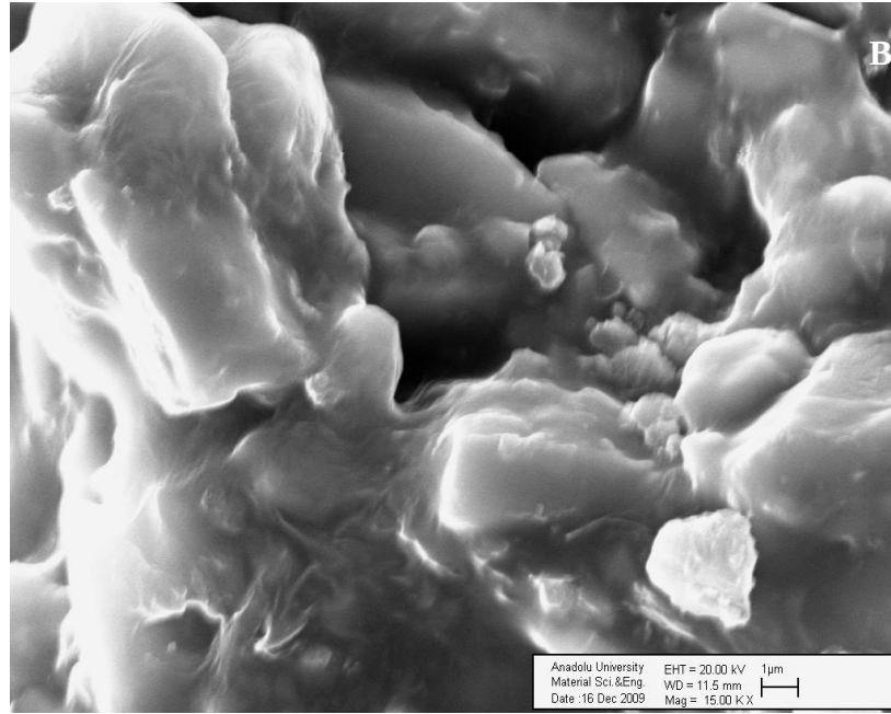
Şekil 5.22. Ağırlıkça %1,6 TS-boya (a), Ağırlıkça %3 TS-boya (b)
