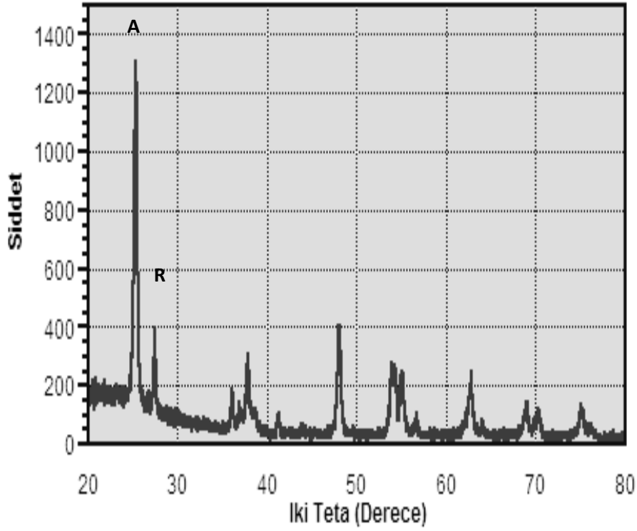
Şekil 5.7. TS tozun 950°C ısıt işlemler sonrası XRD analizi
