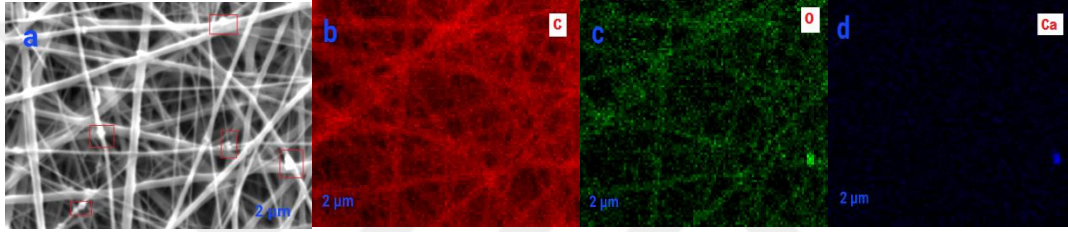
Şekil 4. 9. %2,5 karpit katkı PVP nanofiberin a) SEM görüntüsü, (b) karbon element haritası, (c) oksijen element haritası
