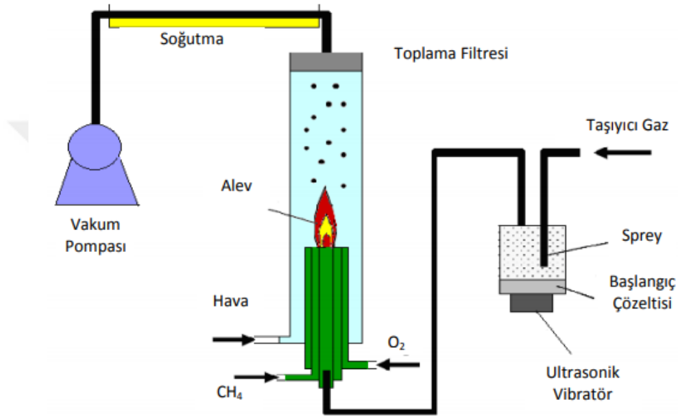
Şekil 2.3. Alev sentezinin aşamalarının gösterimi (Kamacı 2019)
