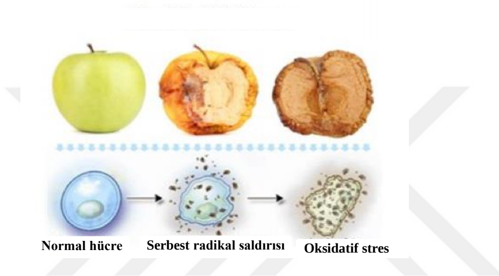
Şekil 4.2. Oksidatif stresin hücrede yarattığı etki (Anonim1)
