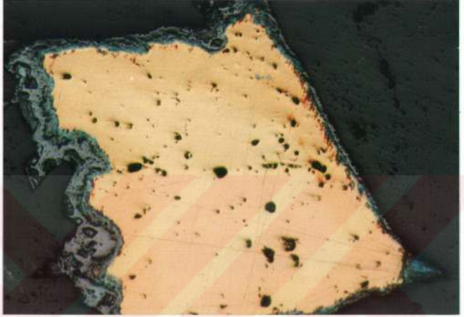
Şekil 3.2: Yarı özşekilli kalkopirit (sarı renkli) ve etrafında, kenarları boyunca gelişmiş kovelin ve kalkozin. ND-1 damarı, yüzeyden (ÇN X 100).
