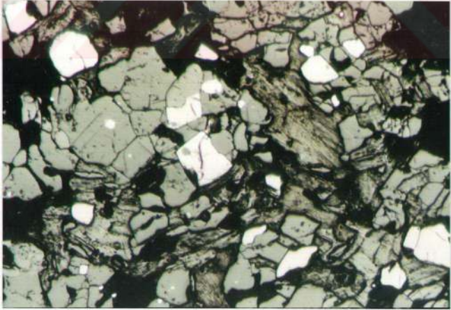
Şekil 3.4: Kayaç içerisinde saçınımlı, özşekli yarı özşekilli pirit (beyaz) taneleri NS-1 sondajı, metraj: 187,40 m. (ÇN X 100).
