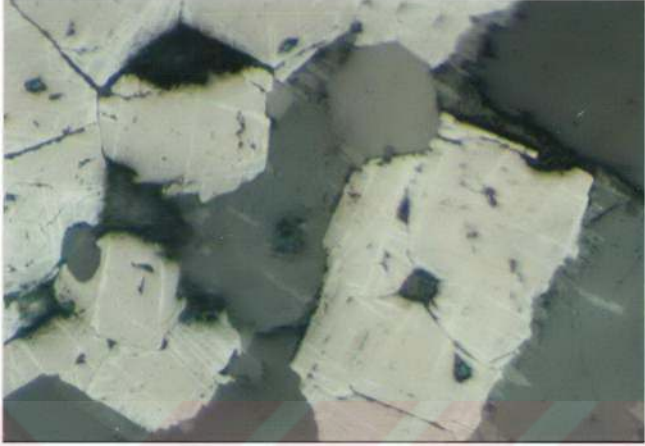
Şekil 3.6: Manyetitlerde (açık gri, kirli beyaz) görülen martitileşmeler (ince çubuğumsu, açık renkli çizgiler). NS-1 sondajı, metraj: 146.00 m (ÇN X 200).
