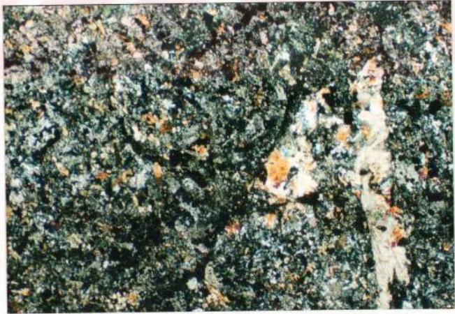
Şekil 2.4: Baskil Granitoidini kesen bazik damar kayaçlarının (diyabaz) polarizan mikroskopta görünümü. NS-2 sondajı, metraj: 7.10 m. (ÇN X 32).
