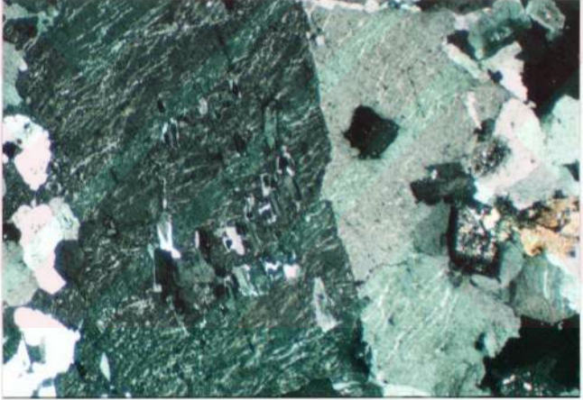
Şekil 2.3: Alkali feldspatlarda albit ayrılımlarından kaynaklanan ipliğimsi pertitler. Kizırüşağı Mahallesi 100 m. güneyi (ÇN X 32).
