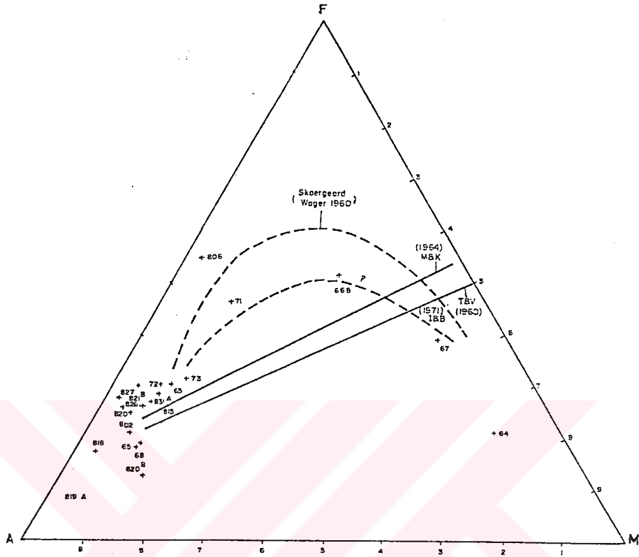
Şekil 2.9: Baskil Mağmatik kayaçlarının AFM diyagramında dağılımı (Asutay, 1985).
