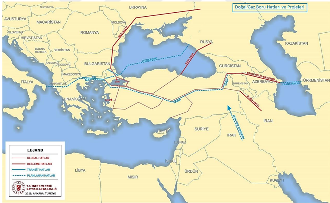
Şekil 13: Trans-Balkan Boru Hattı-Batı Boru Hattı
