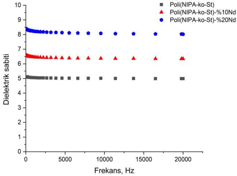
Şekil 3.9. Poli(NIPA-ko-St) kopolimeri, poli(NIPA-ko-St)-%10Nd kompoziti ve poli(NIPA-ko-St)-%20Nd kompozitinin dielektrik sabitinin frekansa bağımlılığı
