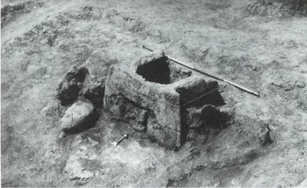
Resim 14: Höyücek TD'nin 1. Yapısı İçindeki Fırın
