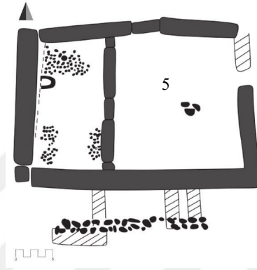
Şekil 14 :Höyücek Tapınak Dönemi 5 Nolu Yapı
