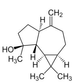
Spatulenol
