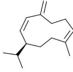
Germakren D
