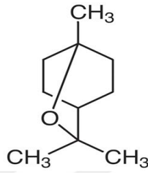
1,8-Sineol
