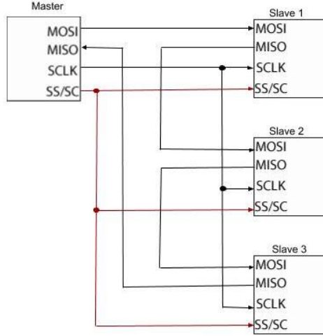
Şekil 3.16 Master düğümün bir SS/SC hattı bulundurması durumunda kullanılabilecek SPI konfigürasyon örneği.
