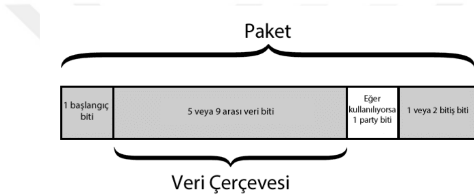
Şekil 3.18 UART paket yapısı
