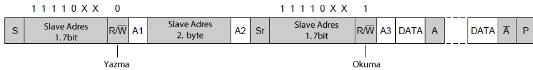
Şekil 3.14 Bir master düğümünden, 10 bit adresli bir slave düğüme yönelik veri iletimi
