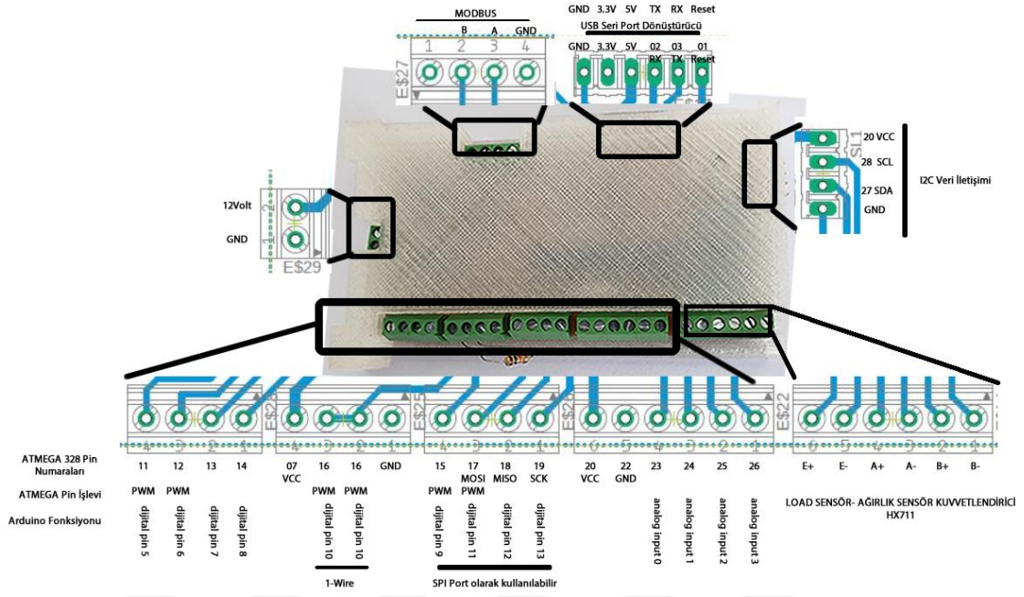
Şekil 3.33 Ek modül bağlantı yuvaları
