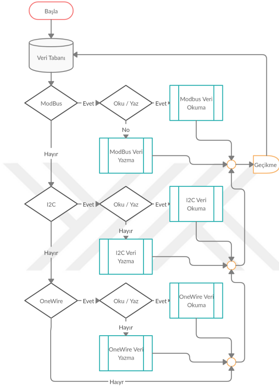
Şekil 3.42 Kullanılan python kodları akış diyagramı
