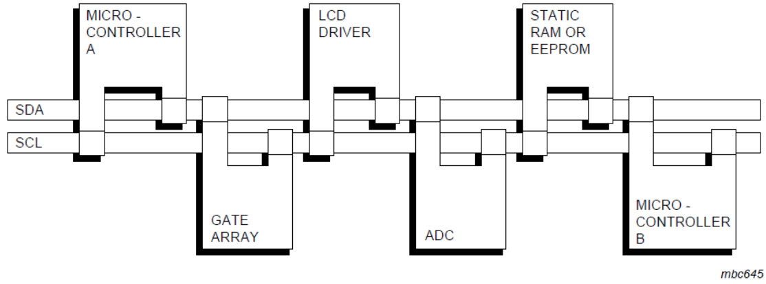
Şekil 3.10 İki mikrodnetleyici kullanan bir I 2 C hat konfigürasyonu örneği
