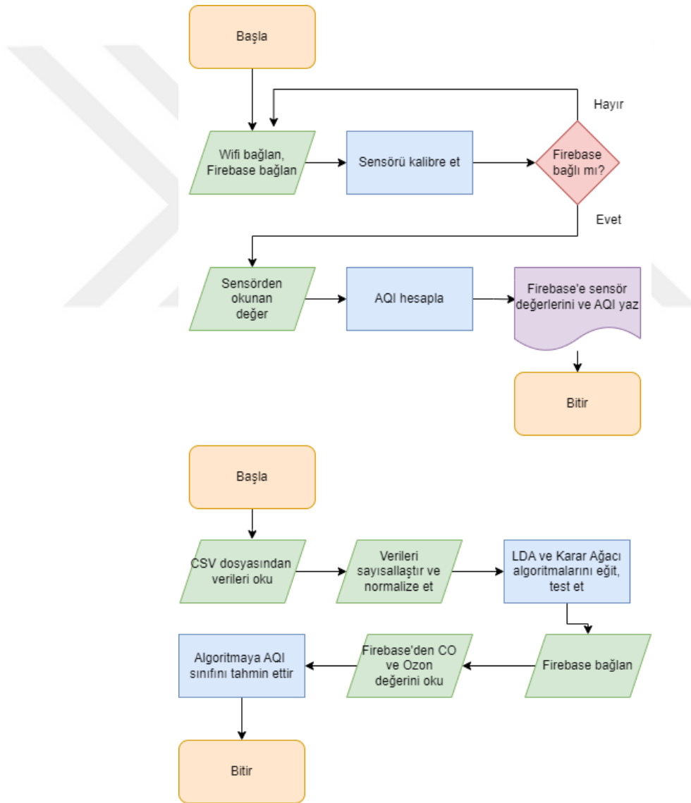
Şekil 4.1. Gerçekleştirilen sistemin akış diyagramı.
