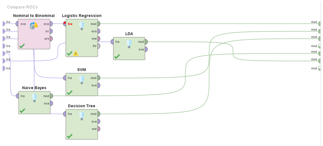
Şekil 3.8. ROC analizi.
