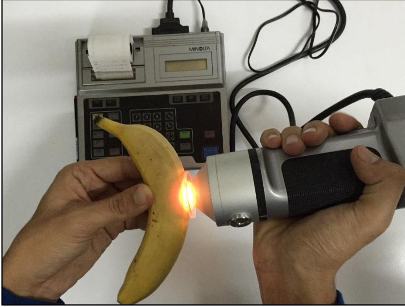
Şekil 3.8. Renk ölçümünün yapıldığı MİNOLTA CR-200 kromametrosi
