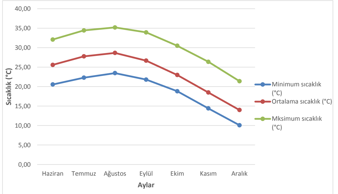
Şekil 4.3. Net örtü sistemi altında, aylar bazında kaydedilen minimum, ortalama ve maksimum sıcaklık değeri (°C)
