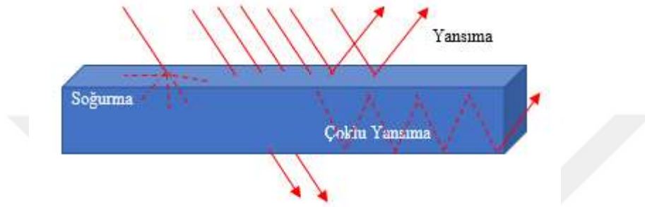
Şekil 2.2. Elektromanyetik Ekranlama Mekanizmasını Gösteren Şematik Gösterimi [39].
