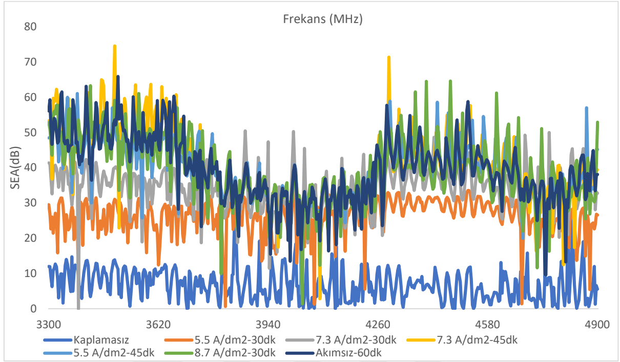
Şekil Ek.4. Numune a. A b. B c. C d. D e. E f.F ve g. Kaplamasız Numuneler için 3300-4900 MHz Frekans Aralığında SEA Değerleri
