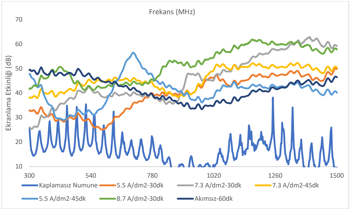
Şekil 4.4. Numune a. A b. B c. C d. D e. E f.F ve g. Kaplamasız Numuneler için 300-1500 MHz Frekans Aralığında Ekranslama Etkinliği Değerleri
