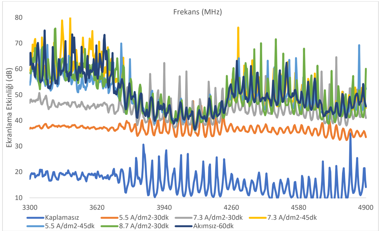
Şekil 4.8. Numune a. A b. B c. C d. D e. E f.F ve g. Kaplamasız Numuneler için 3300-4900 MHz Frekans Aralığında Ekranlama Etkinliği Değerleri
