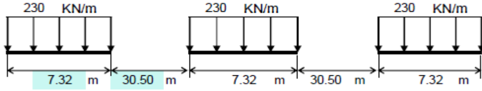
Şekil 4.6. Köprüye uygulanan yükleme modeli
