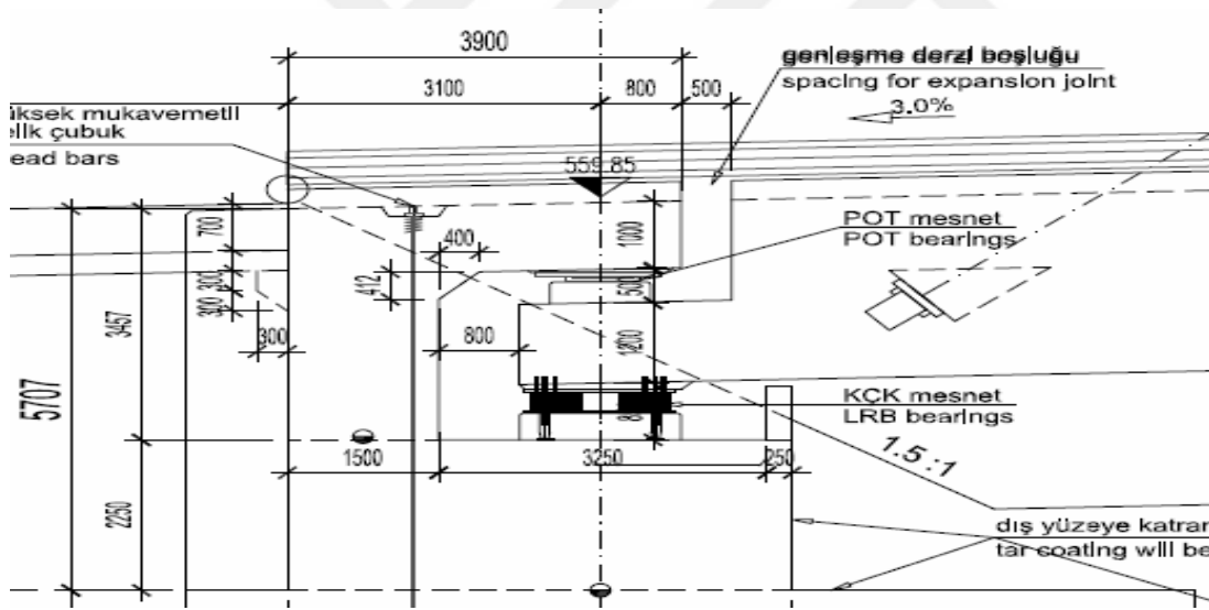
Şekil 3.24. Kurşun Çekirdekli Kauçuk ve Pot Mesnet Kesiti
