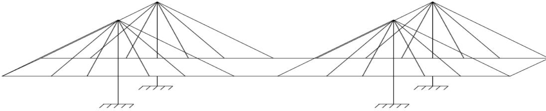
Şekil 2.17. Kablonun İki Düzlemde Yerleştirilmesi
