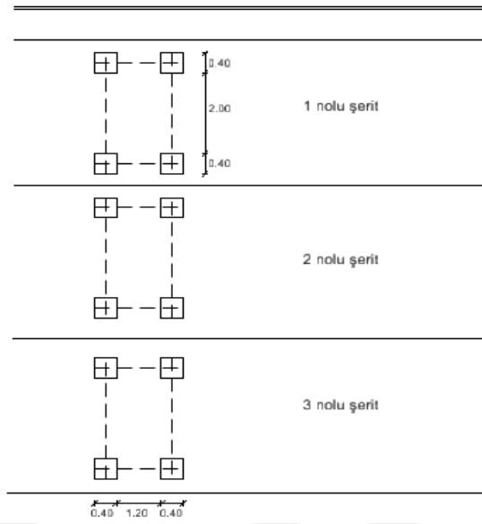
Şekil 4.3. Köprüye uygulanan yükleme modeli
