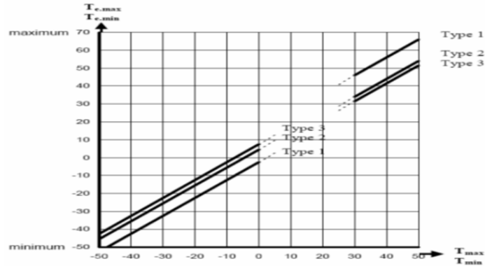
Çizelge 4.6. Köprüdeki Betonarme, Çelik ve Kompozitin Maksimum, Minimum Sıcaklık Değeri
