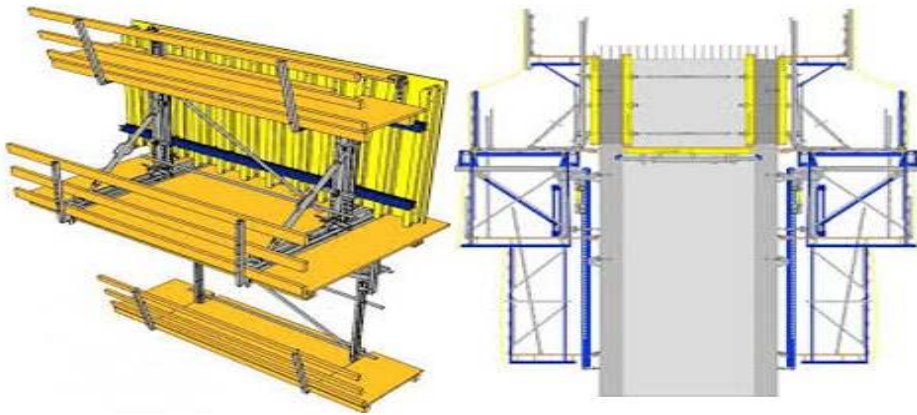
Şekil 4.41. Pilon İmalatında Kullanılan Kalıp Sistemi
