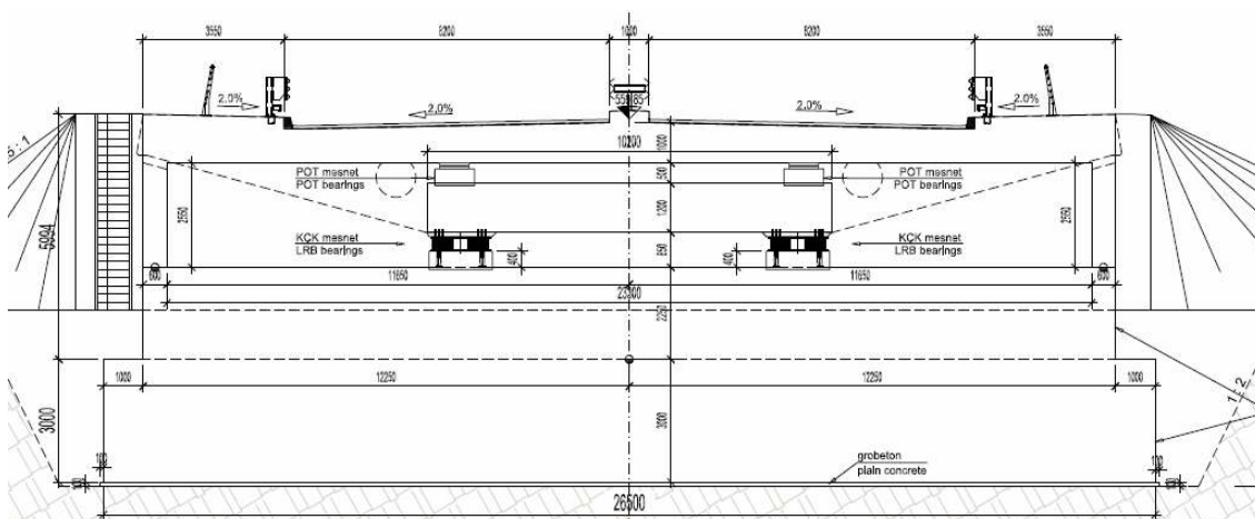
Şekil 3.20. Kenar Açıklıktaki Kenar ayak Kesiti
