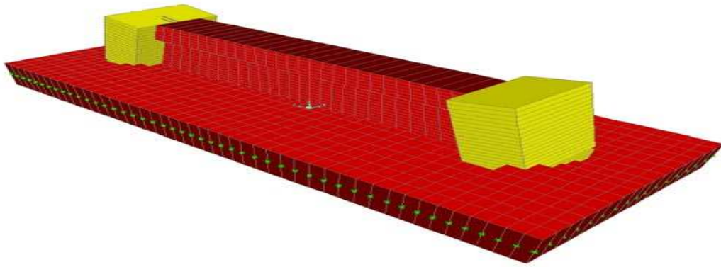
Şekil 3.15. Pilon Temelinin Sistem Modeli
