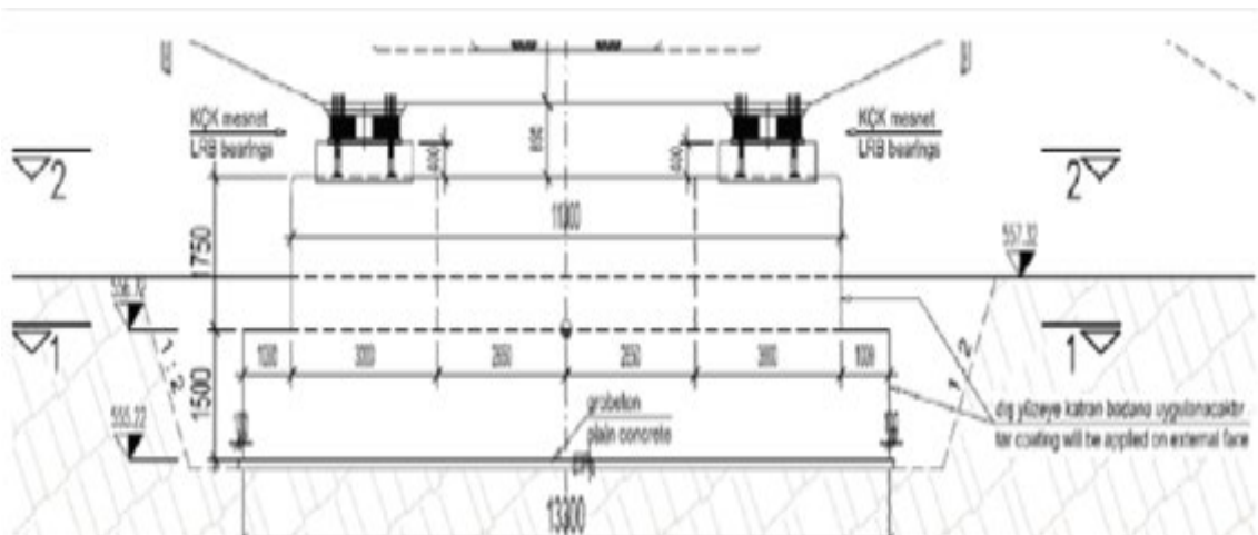
Şekil 3.17. Kenar Açıklıktaki Orta ayak Planı
