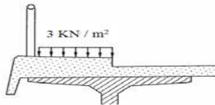
Şekil 4.10. Köprüye etki eden yaya yükü
