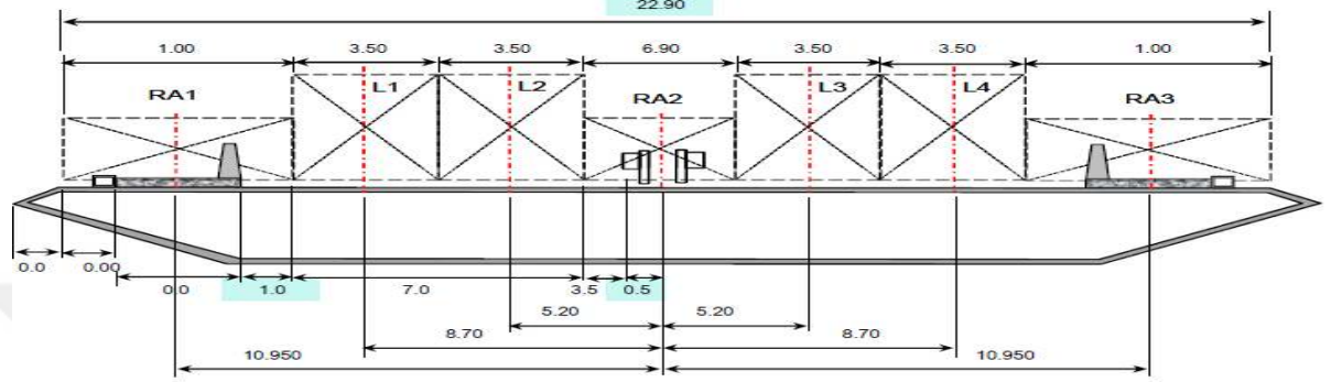
Şekil 4.1. Köprü kesiti
