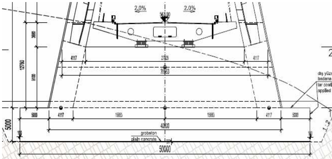
Şekil 3.14. Pylon Temelinin Enkesiti
