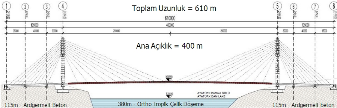
Şekil 3.2. Nissibi eğik kablo askılı köprünün boy kesiti
