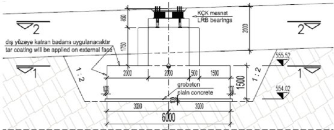
Şekil 3.16. Kenar Açıklıktaki Orta ayak Kesiti
