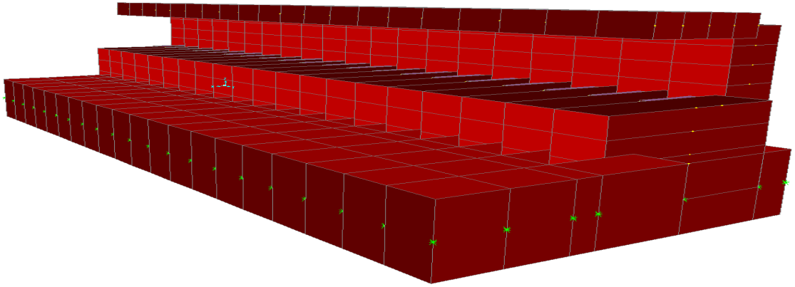
Şekil 3.21. Kenar Açıklıktaki Kenar ayak Sistem Modeli
