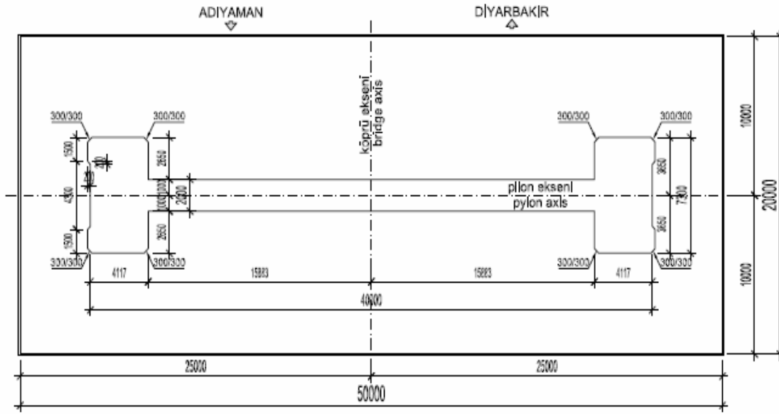
Şekil 3.13. Pylon Temel Boyutu
