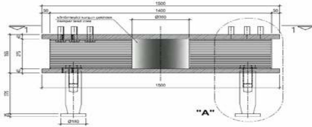
Şekil 3.23. Kurşun Çekirdekli Kaucuk Mesnet Kesiti
