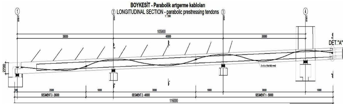
Şekil 4.31. Kenar Açıklık Parabolik Ard germe Kablosunun Boy Kesiti
