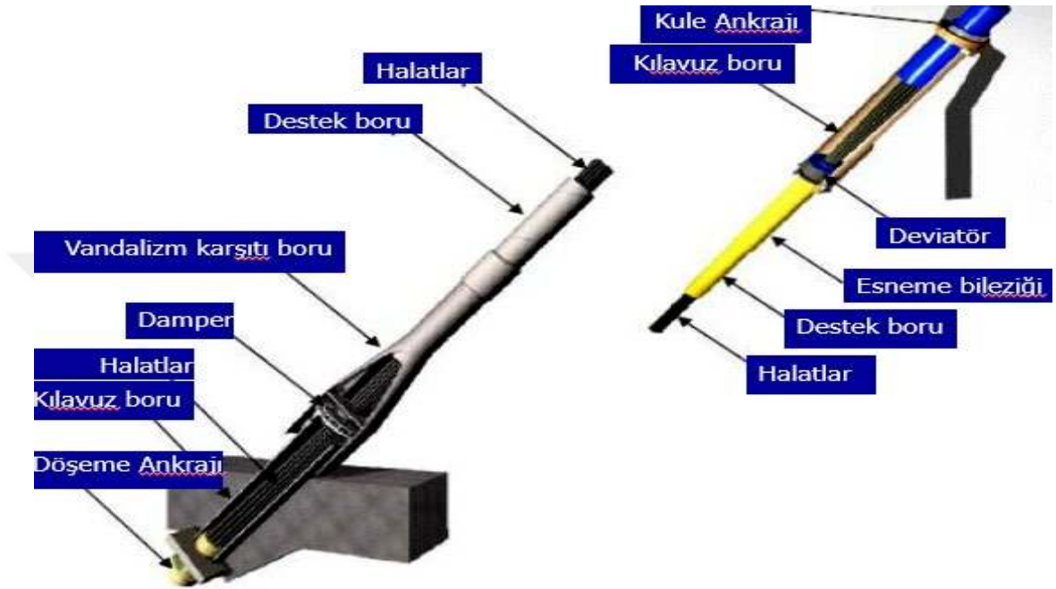
Şekil 4.62. Kablo Kesitinde Bulunan Malzemeler
