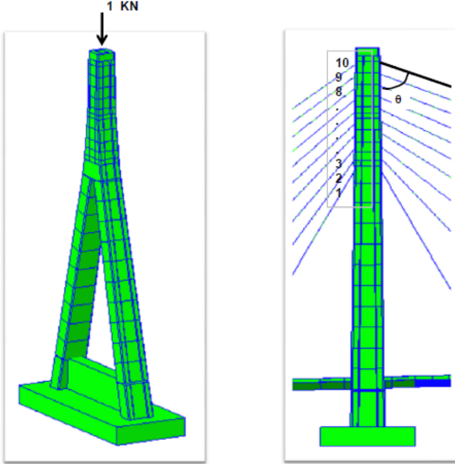
Şekil 4.11. kN ’luk yükün pilona uygulanması
