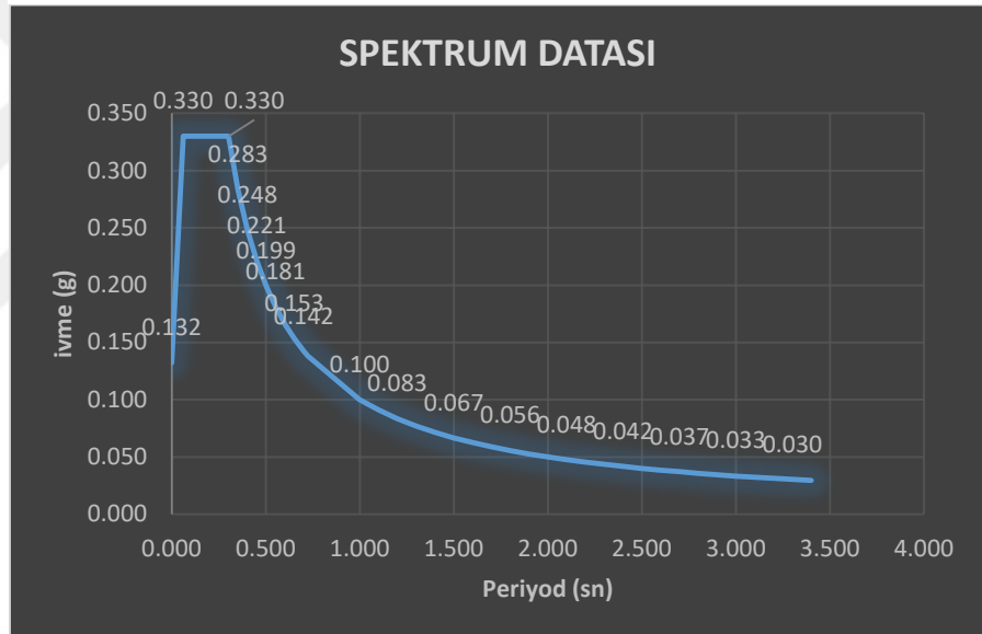
Çizelge 4.9. D1 Deprem Spektral İvme Grafiği
