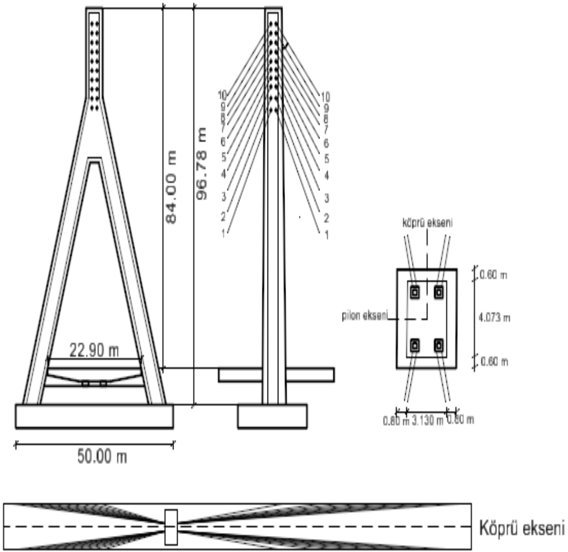
Şekil 3.6. Pilonun Boy-En Kesiti ve Üsten Görünümü
