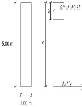
Şekil 4.12. Temel betonarme kesiti
