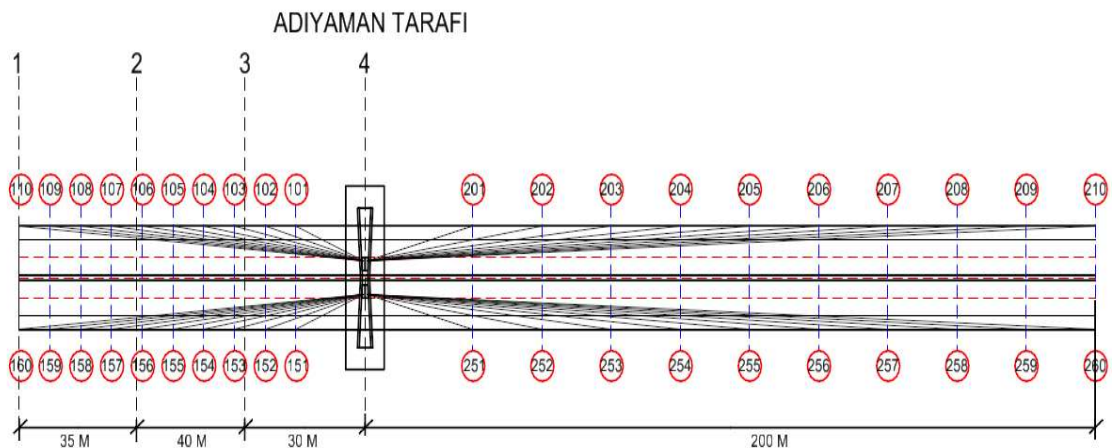
Şekil 3.11. Köprünün Adıyaman tarafındaki kısmının kablolarının yerleşmiş halindeki planın üstten görünümü
