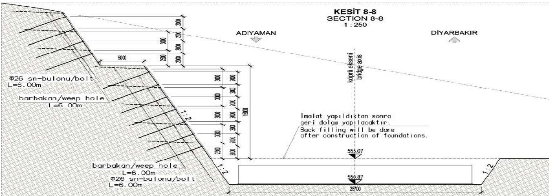
Şekil 4.18. Şev Destekleme Sisteminin Kesiti
