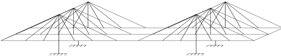
Şekil 2.18. Kablonun Üç Düzlemde Yerleştirilmesi
