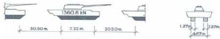
Şekil 4.5. Modelde uygulanan tank tipi
