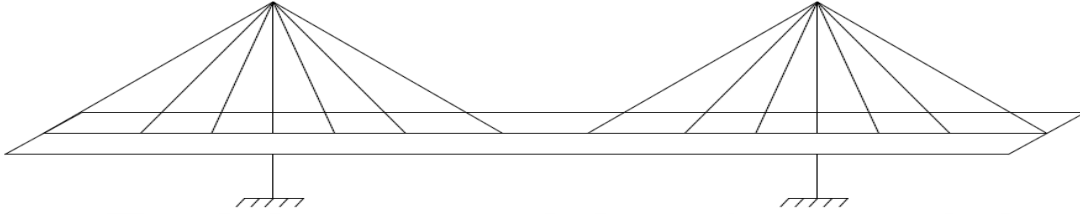
Şekil 2.16. Kablonun Tek Düzlemde Yerleştirilmesi
