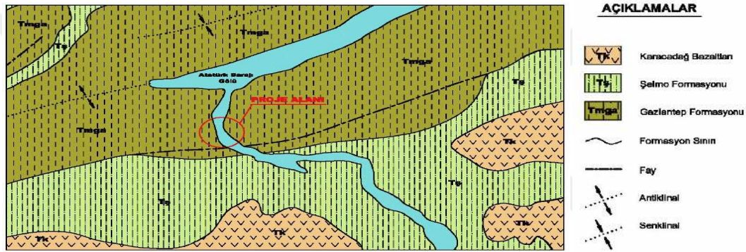
Şekil 3.3 Proje Bölgesinin Jeolojik haritası
