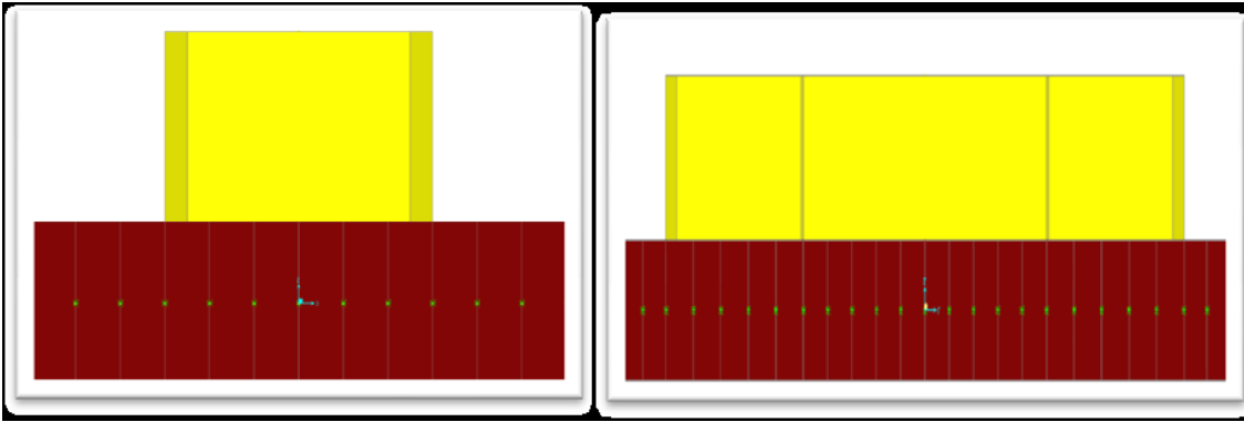
Şekil 3.18. Kenar Açıklığıtaki Orta ayak Sistem Modeli
