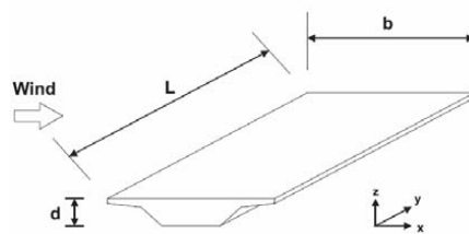
Şekil 4.8. Tabliye Kesiti
