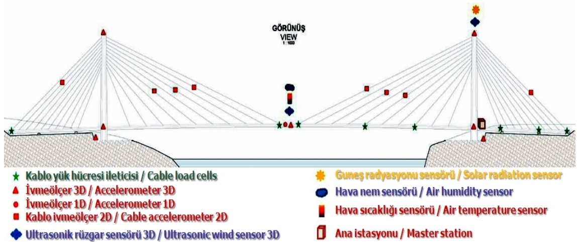
Şekil 4.74. Köprü İzleme Sisteminin Kurulması
