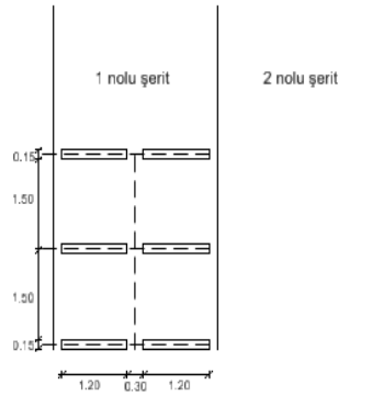
Şekil 4.7. Köprüye uygulanan yükleme modeli
