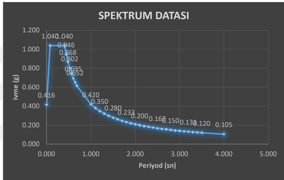
Çizelge 4.11. D3 Deprem Spektral İvme Grafiği
