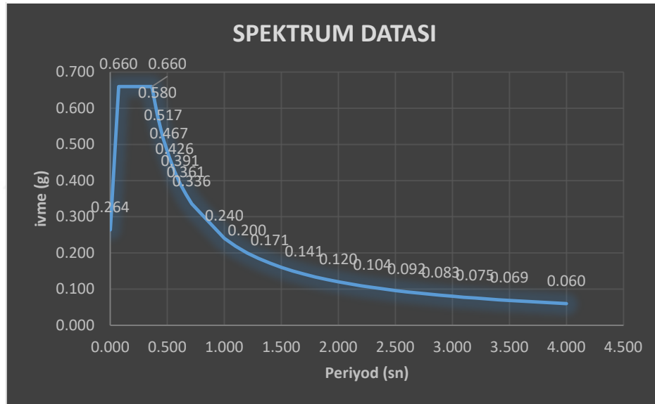
Çizelge 4.10. D2 Deprem Spektral İvme Grafiği
