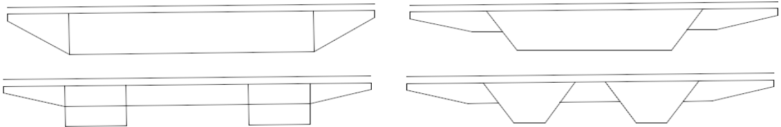
Şekil 2.20. Kutu Kesitli Tabliye Tipleri
