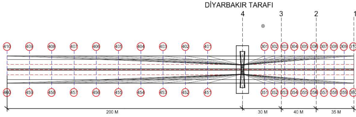
Şekil 3.12. Köprünün Diyarbakır tarafındaki kısmın kablolarının yerleşmiş halindeki planın üstten görünümü
