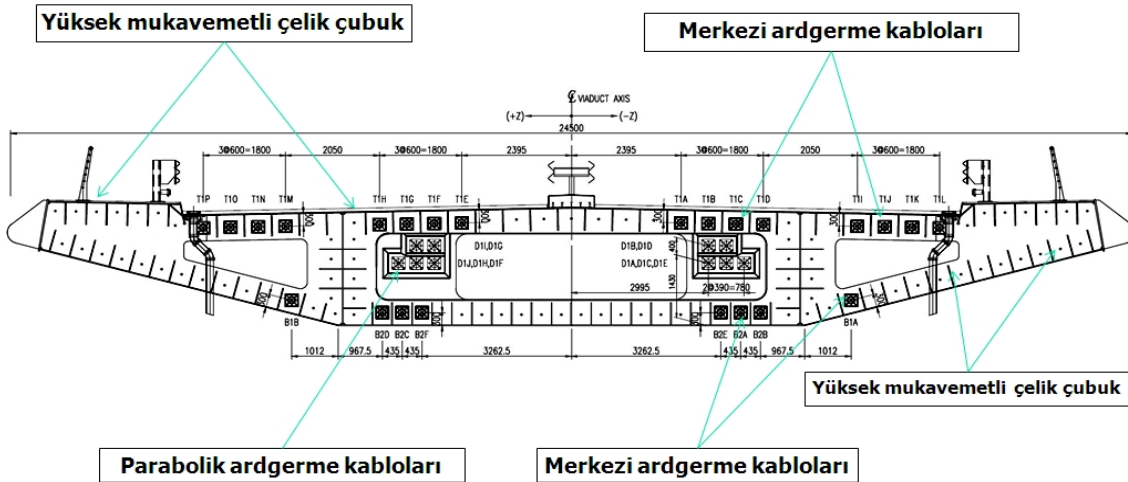
Şekil 4.45. İlk Çelik Segmentin Kesiti
