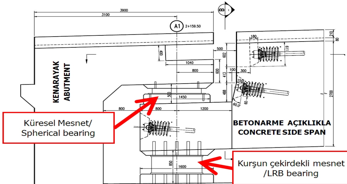
Şekil 4.26. Kenar ayak Temelinin Mesnet Bandı Kotuna Getirilmesi
