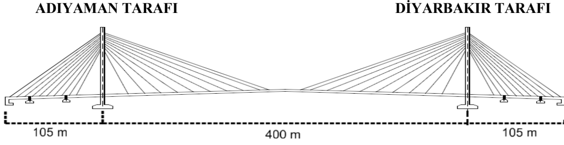
Şekil 3.25. Köprünün Geometrisi
