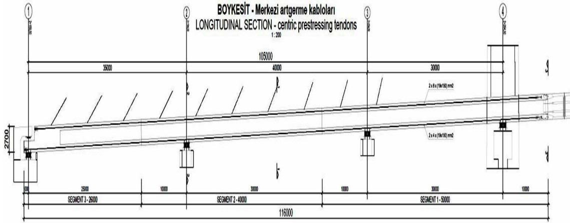
Şekil 4.32. Kenar Açıklık Merkezi Ard germe Kablosunun Boy Kesiti
