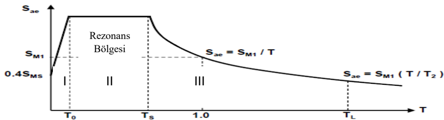
Çizelge 4.8. Spektral İvme Grafiği
