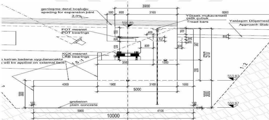
Şekil 3.19. Kenar Açıklıktaki Kenar ayak Temel Boyutu
