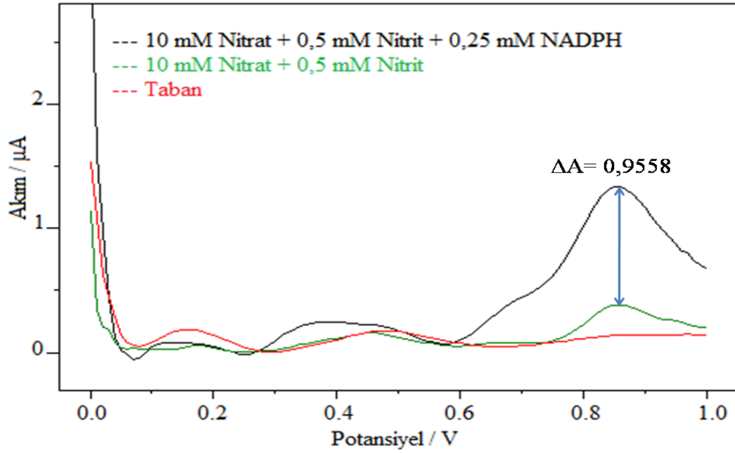
Şekil 4.124. PU-L-%1 polimeri ile hazırlanan biyosensörle 10 mM nitrat tayini için DPV eğrileri [0,5 U NR; 2 \mu\text{L} PU-L-%1; 100 mM, pH 7,5 fosfat tamponu; 25 \pm 2 °C].
