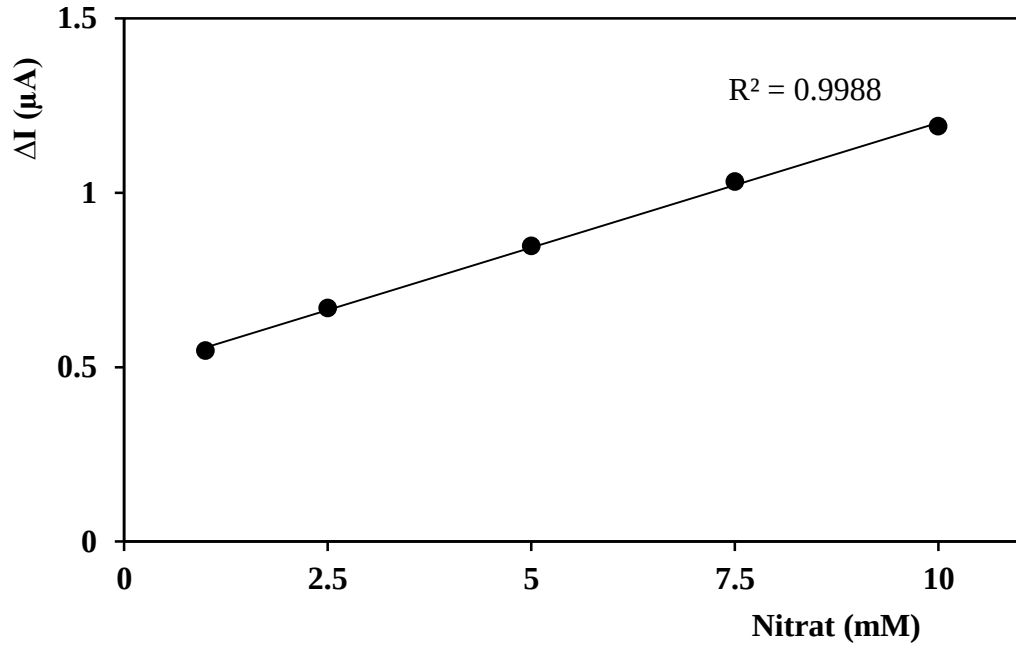
Şekil 4.167. PU-Maltoz-%1 polimeri ile hazırlanan biyosensörle nitrat tayinine yönelik doğrusal tayin aralığı [0,5 U NR; 2 \mu L PU-Maltoz-%1; 100 mM, pH 7,5 fosfat tamponu; 25 \pm 2 ^{\circ} C; 0,87 V; DPV].
