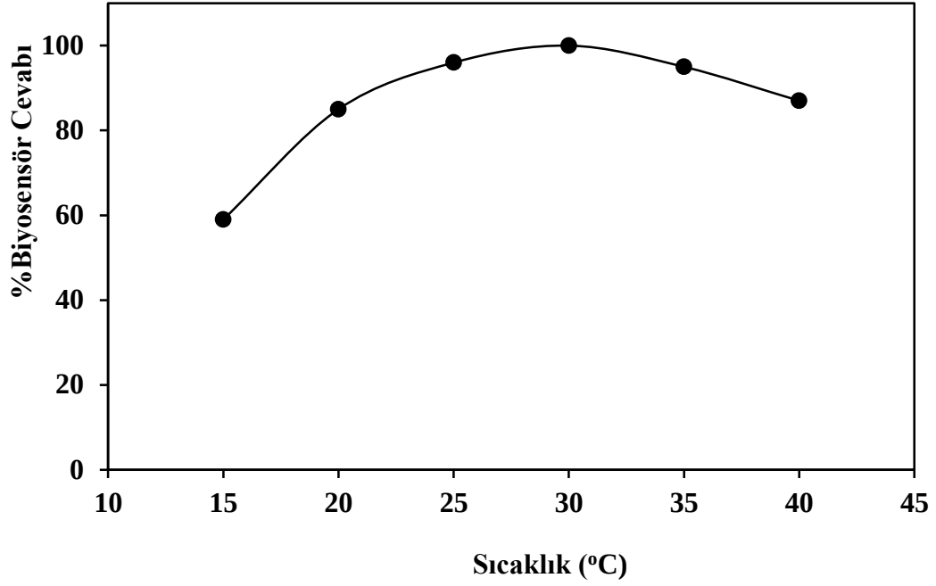
Şekil 4.155. PU-Maltoz-%1 polimeri ile hazırlanan biyosensörün optimum sıcaklık grafiği [0,5 U NR; 2 µL PU-Maltoz-%1; 0,25 mM NADPH; 100 mM, pH 7,5 fosfat tamponu; +0,87 V; DPV].
