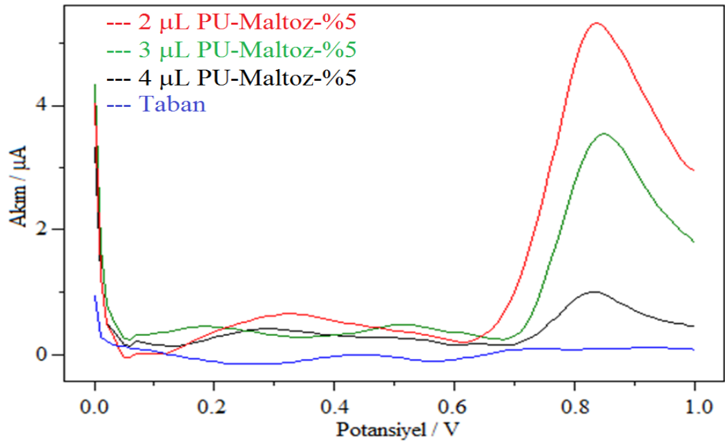
Şekil 4.65. Platin elektrodun PU-Maltoz-%5 polimeri ile kaplanması ve nitrit ölçümü [100 mM, pH 7,5 fosfat tamponu; 25\pm 2 °C; DPV].
