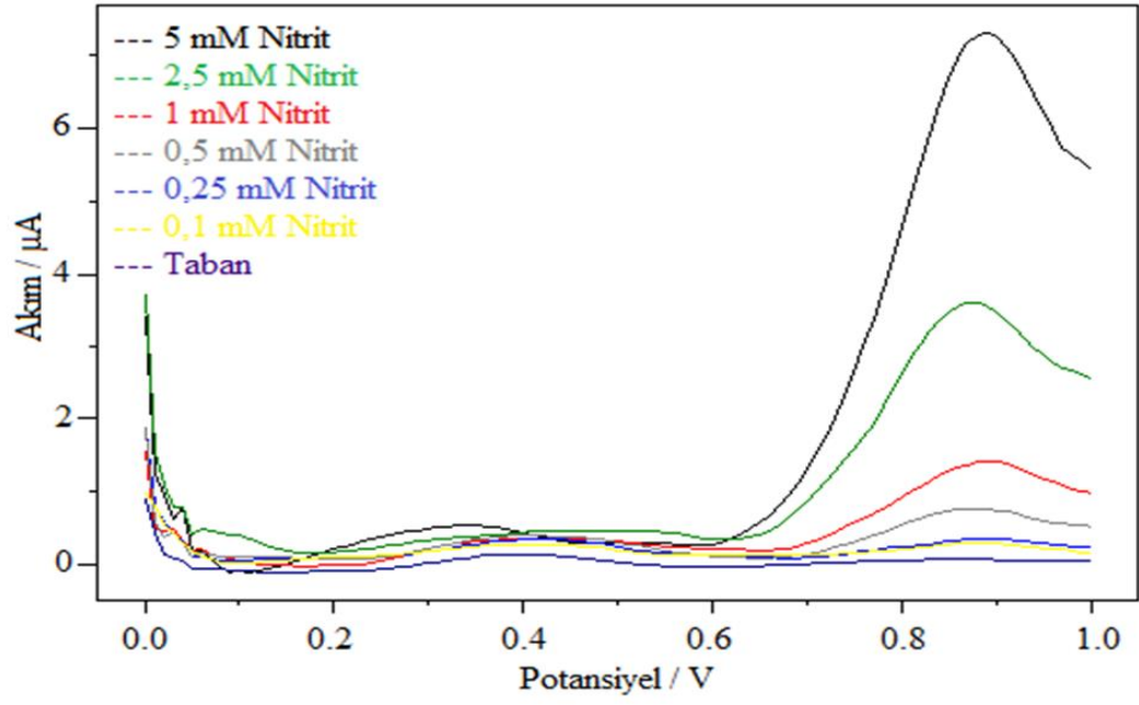
Şekil 4.36. Çıplak platin elektrotla 0,1 mM – 5 mM aralığındaki nitrit derişimleri için alınan DPV eğrileri [100 mM, pH 7,5 fosfat tamponu; 25 \pm 2 °C].
