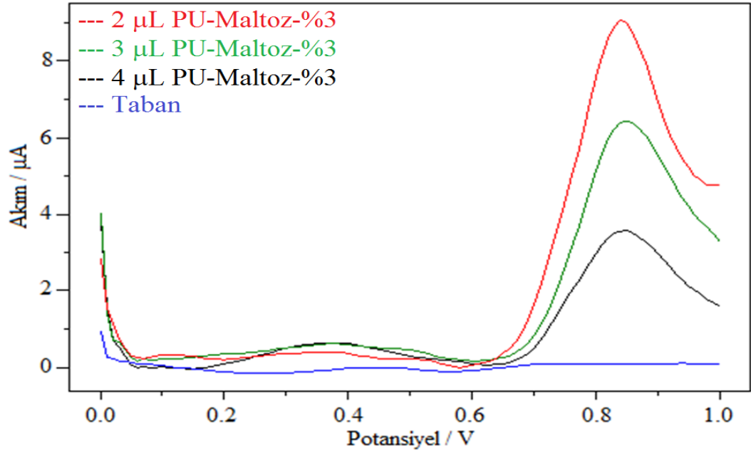
Şekil 4.64. Platin elektrodun PU-Maltoz-%3 polimeri ile kaplanması ve nitrit ölçümü [100 mM, pH 7,5 fosfat tamponu; 25\pm 2 °C; DPV].
