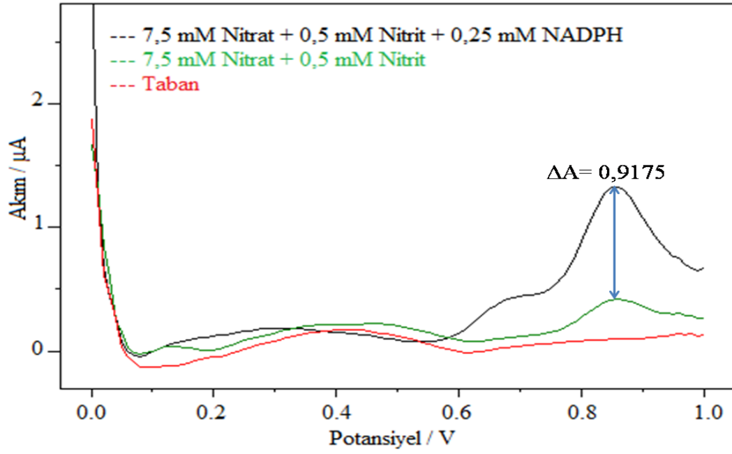
Şekil 4.83. PU-F-%1 polimeri ile hazırlanan biyosensörle 7,5 mM nitrat tayini için DPV eğrileri [0,5 U NR; 2 µL PU-F-%1; 100 mM, pH 7,5 fosfat tamponu; 25±2 °C].
