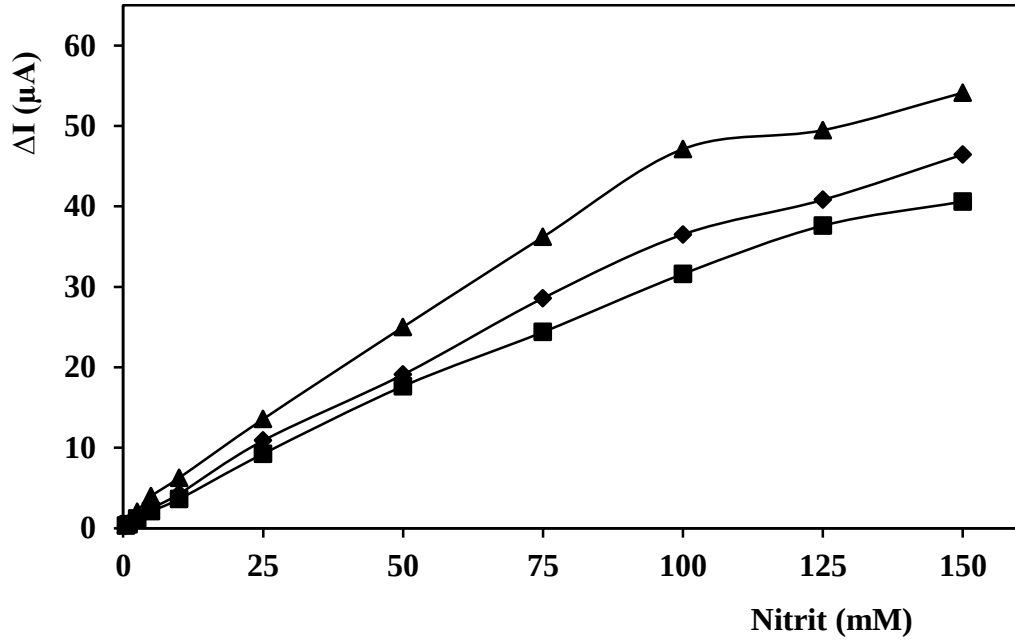
Şekil 4.71. Nitrit ölçümü için enzim miktarının PU-F-%1 polimeri ile hazırlanan biyosensör cevabına etkisi [2 µL PU-F-%1; 0,25 mM NADPH; 100 mM, pH 7,5 fosfat tamponu; 25±2 °C; +0,87 V; DPV; ▲ 0,25 U; ♦ 0,5 U; ■ 1 U].
