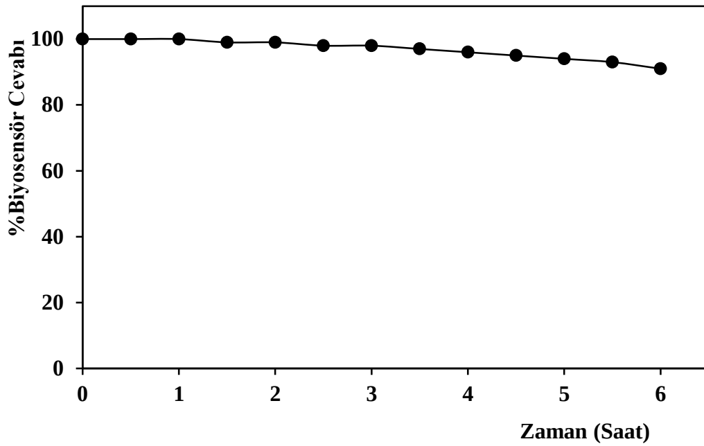
Şekil 4.148. PU-X-%1 polimeri ile hazırlanan biyosensörün operasyonel kararlılığı [0,5 U NR; 2 \mu L PU-X-%1; 0,25 mM NADPH; 100 mM, pH 7,5 fosfat tamponu; 25 \pm 2 °C; +0,87 V; DPV].
