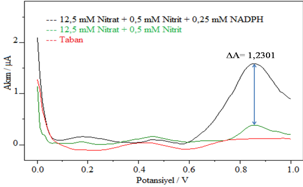
Şekil 4.145. PU-X-%1 polimeri ile hazırlanan biyosensörle 12,5 mM nitrat tayini için DPV eğrileri [0,5 U NR; 2 \mu\text{L} PU-X-%1; 100 mM, pH 7,5 fosfat tamponu; 25 \pm 2 °C].
