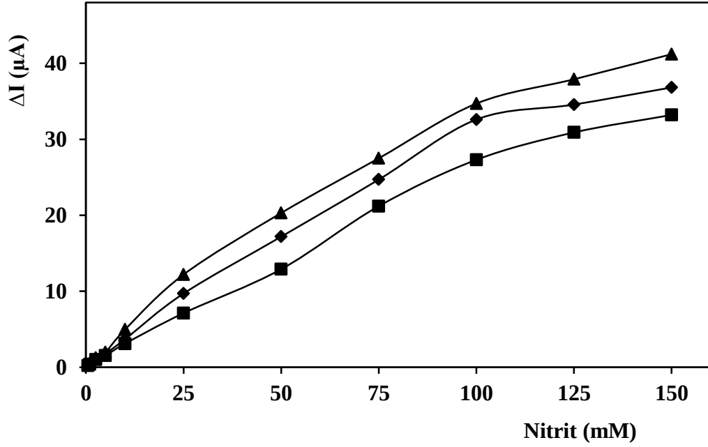
Şekil 4.91. Nitrit ölçümü için enzim miktarının PU-M-%1 polimeri ile hazırlanan biyosensör cevabına etkisi [2 \mu L PU-M-%1; 0,25 mM NADPH; 100 mM, pH 7,5 fosfat tamponu; 25 \pm 2 °C; +0,87 V; DPV; ▲ 0,25 U; ◆ 0,5 U; ■ 1 U].
