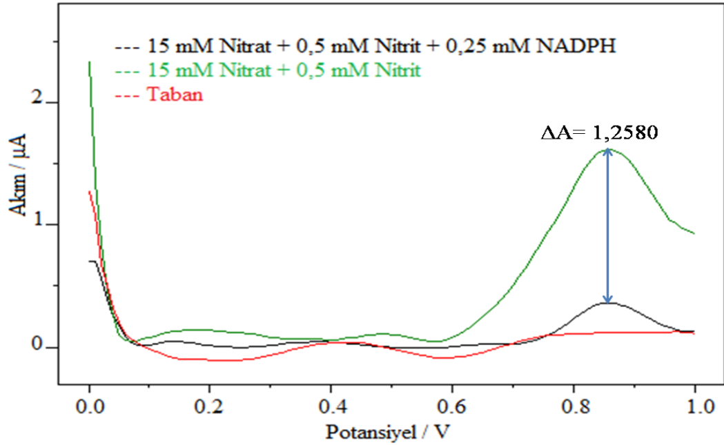
Şekil 4.146. PU-X-%1 polimeri ile hazırlanan biyosensörle 15 mM nitrat tayini için DPV eğrileri [0,5 U NR; 2 \mu\text{L} PU-X-%1; 100 mM, pH 7,5 fosfat tamponu; 25 \pm 2 °C].
