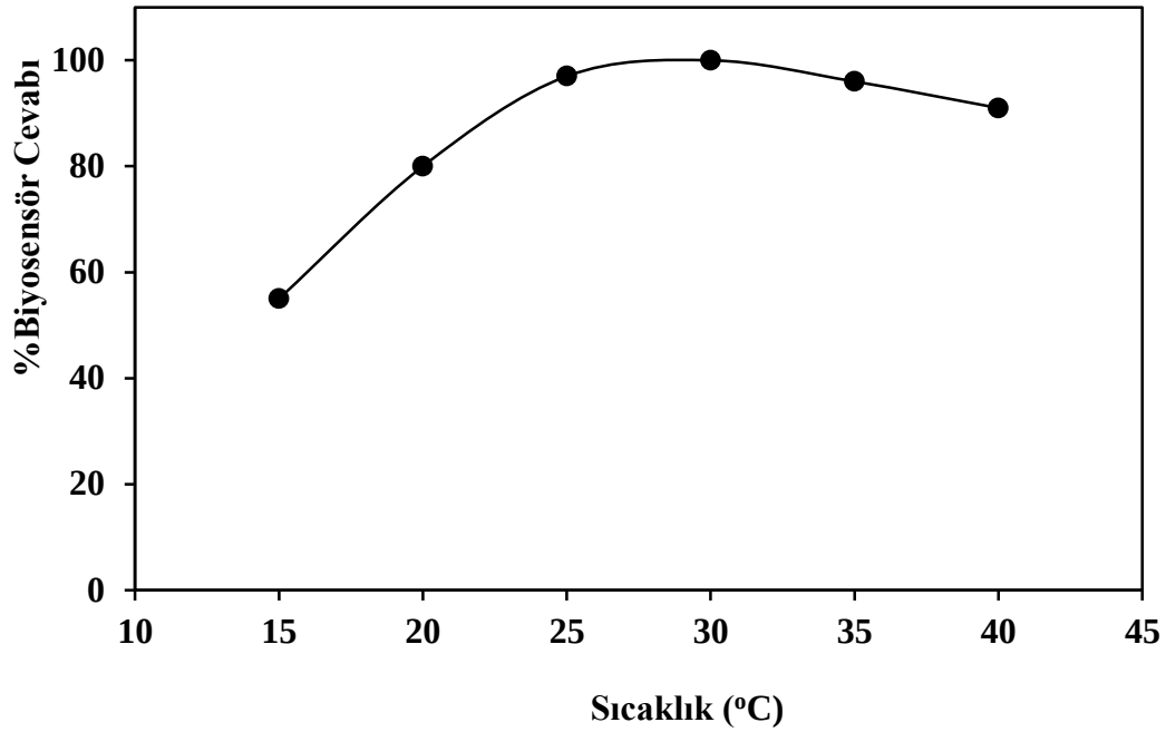
Şekil 4.95. PU-M-%1 polimeri ile hazırlanan biyosensörün optimum sıcaklık grafiği [0,5 U NR; 2 µL PU-M-%1; 0,25 mM NADPH; 100 mM, pH 7,5 fosfat tamponu; +0,87 V; DPV].
