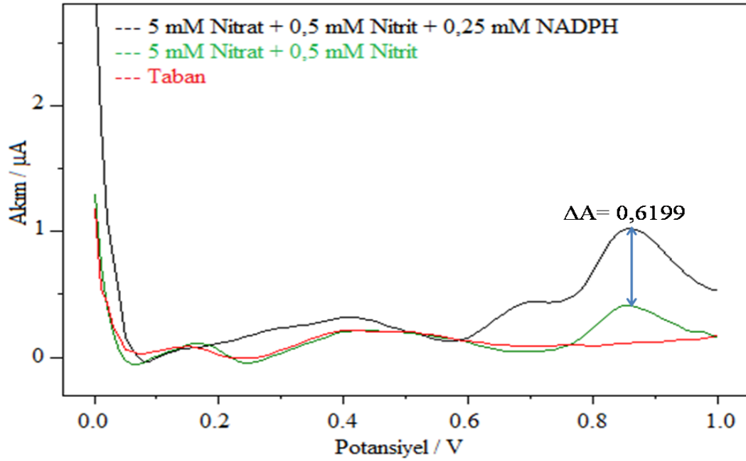
Şekil 4.102. PU-M-%1 polimeri ile hazırlanan biyosensörle 5 mM nitrat tayini için DPV eğrileri [0,5 U NR; 2 \mu L PU-M-%1; 100 mM, pH 7,5 fosfat tamponu; 25 \pm 2 °C].
