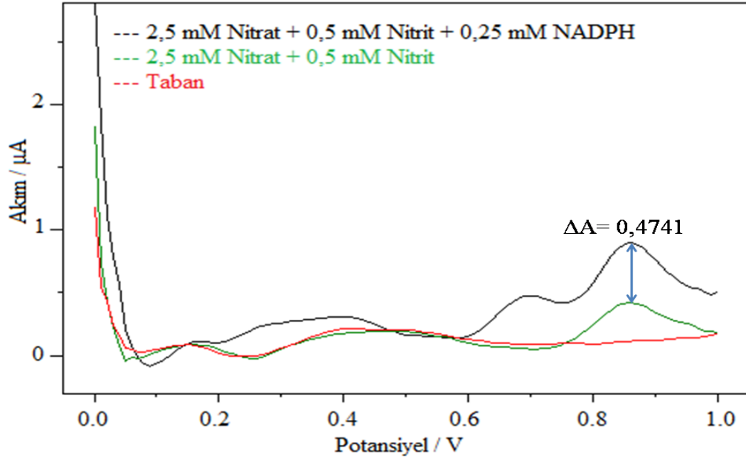
Şekil 4.101. PU-M-%1 polimeri ile hazırlanan biyosensörle 2,5 mM nitrat tayini için DPV eğrileri [0,5 U NR; 2 \mu L PU-M-%1; 100 mM, pH 7,5 fosfat tamponu; 25 \pm 2 °C].
