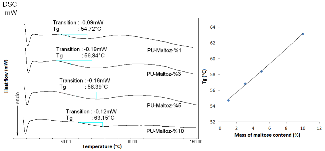
Şekil 4.28. Gliserol içermeyen maltoz temelli poliüretanlara ait DSC termogramları ve T_g değerleri.
