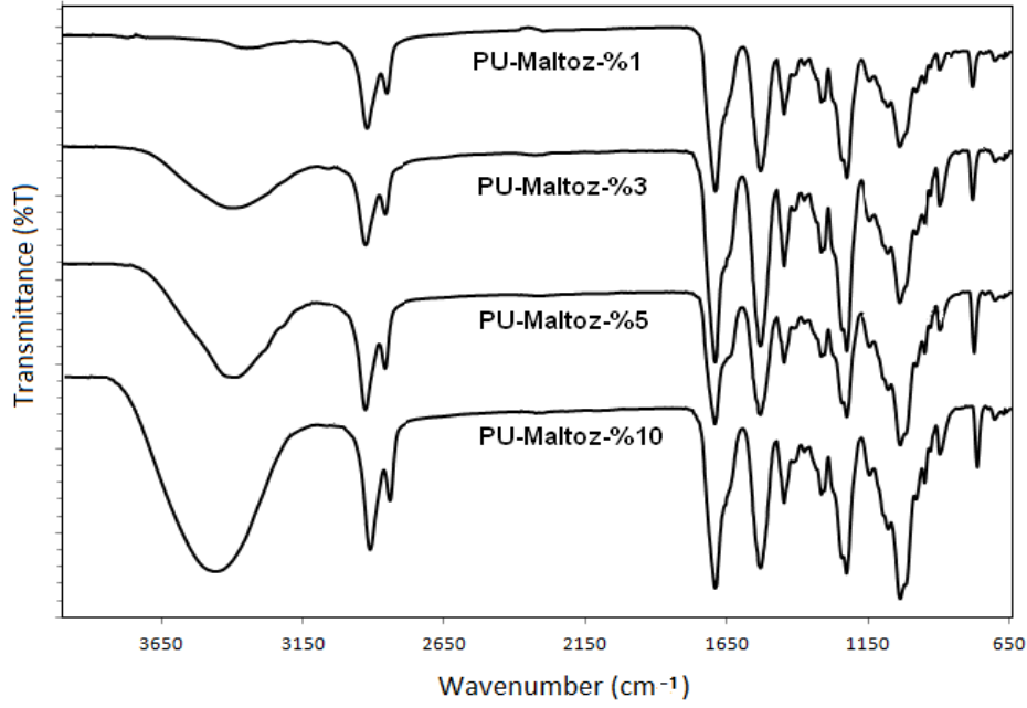
Şekil 4.25. Gliserol içermeyen maltos temelli poliüretanlara ait FTIR spektrumları.
