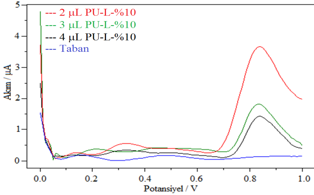
Şekil 4.54. Platin elektrodun PU-L-%10 polimeri ile kaplanması ve nitrit ölçümü [100 mM, pH 7,5 fosfat tamponu; 25 \pm 2 °C; DPV].
