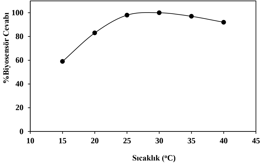
Şekil 4.115. PU-L-%1 polimeri ile hazırlanan biyosensörün optimum sıcaklık grafiği [0,5 U NR; 2 \mu L PU-L-%1; 0,25 mM NADPH; 100 mM, pH 7,5 fosfat tamponu; +0,87 V; DPV].
