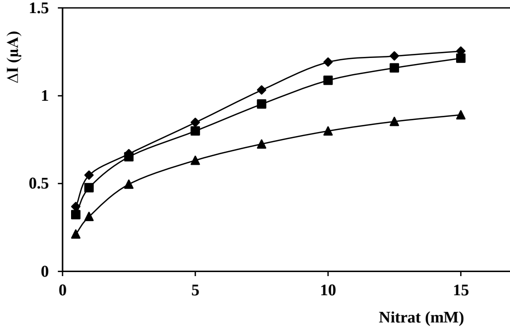
Şekil 4.152. Nitrat ölçümü için enzim miktarının PU-Maltoz-%1 polimeri ile hazırlanan biyosensör cevabına etkisi [2 µL PU-Maltoz-%1; 0,25 mM NADPH; 100 mM, pH 7,5 fosfat tamponu; 25±2 °C; +0,87 V; DPV; ▲ 0,25 U; ♦ 0,5 U; ■ 1 U].
