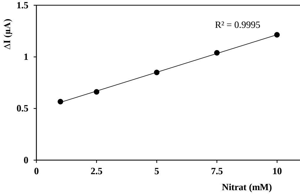
Şekil 4.147. PU-X-%1 polimeri ile hazırlanan biyosensörle nitrat tayinine yönelik doğrusal tayin aralığı [0,5 U NR; 2 \mu L PU-X-%1; 100 mM, pH 7,5 fosfat tamponu; 25 \pm 2 °C; 0,87 V; DPV].
