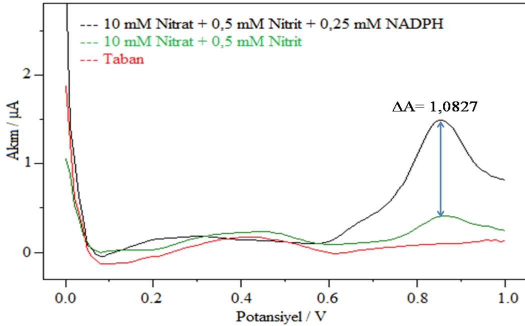
Şekil 4.84. PU-F-%1 polimeri ile hazırlanan biyosensörle 10 mM nitrat tayini için DPV eğrileri [0,5 U NR; 2 µL PU-F-%1; 100 mM, pH 7,5 fosfat tamponu; 25±2 °C].
