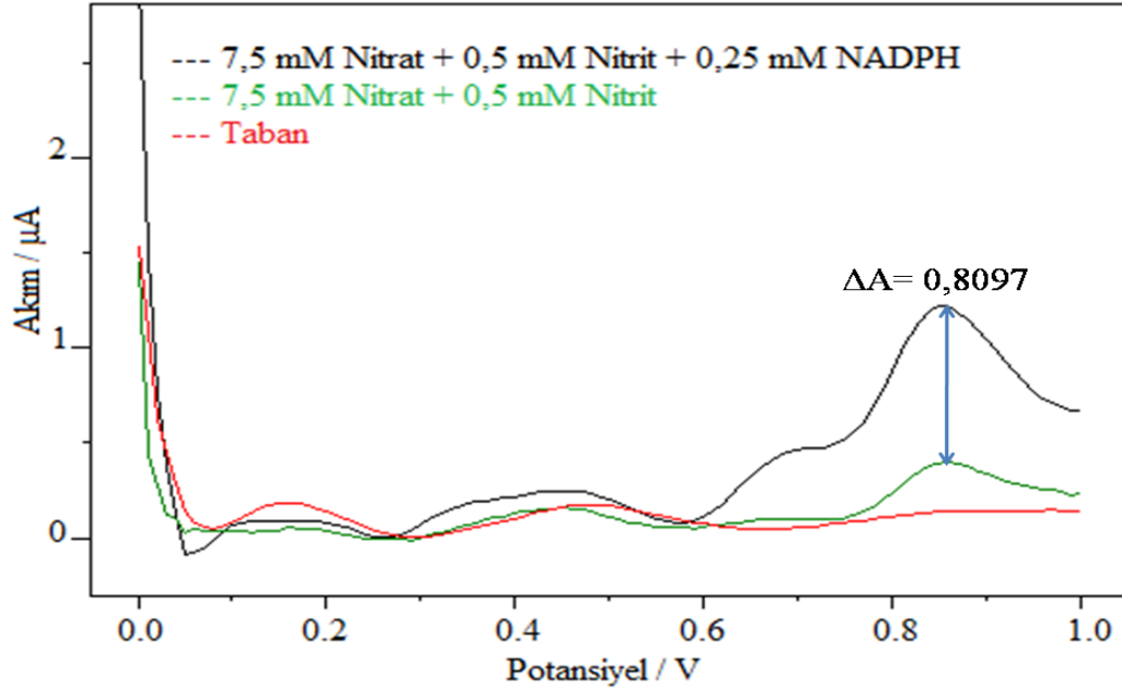
Şekil 4.123. PU-L-%1 polimeri ile hazırlanan biyosensörle 7,5 mM nitrat tayini için DPV eğrileri [0,5 U NR; 2 \mu\text{L} PU-L-%1; 100 mM, pH 7,5 fosfat tamponu; 25 \pm 2 °C].
