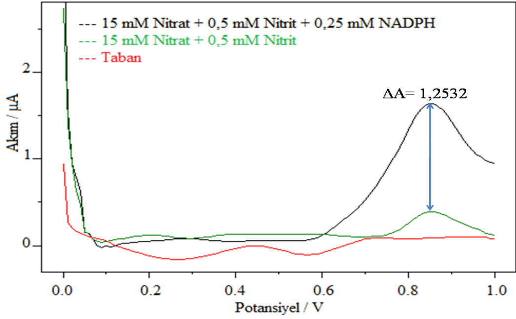
Şekil 4.166. PU-Maltoz-%1 polimeri ile hazırlanan biyosensörle 15 mM nitrat tayini için DPV eğrileri [0,5 U NR; 2 \mu L PU-Maltoz-%1; 100 mM, pH 7,5 fosfat tamponu; 25 \pm 2 ^{\circ} C].
