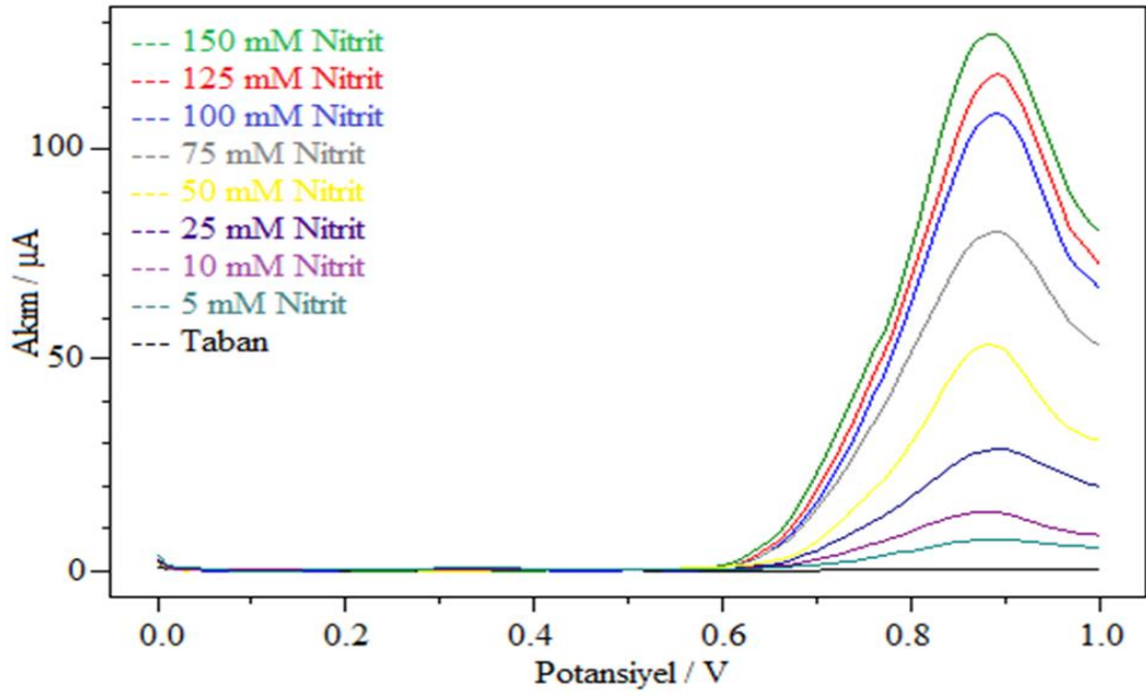
Şekil 4.37. Çıplak platin elektrotla 5 mM – 150 mM aralığındaki nitrit derişimleri için alınan DPV eğrileri [100 mM, pH 7,5 fosfat tamponu; 25 \pm 2 °C].
