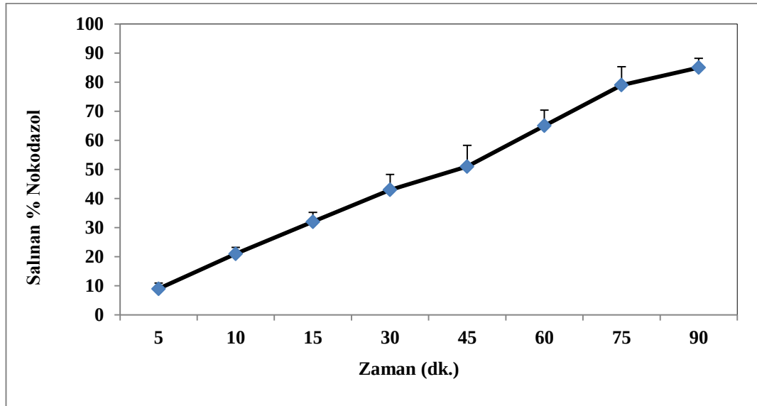
Şekil 3.16. Nokodazol'un zamana bağlı salım grafiği (pH6.8)
