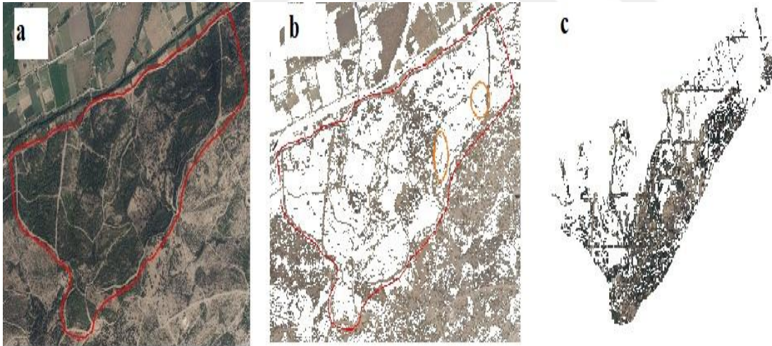
Şekil 4.10 a) İkinci çalışma alanı nokta bulutu, b) NDVI değerleri ile filtrenilmiş görünümü, c) CSF algoritması ile filtrenilmiş görünümü.
