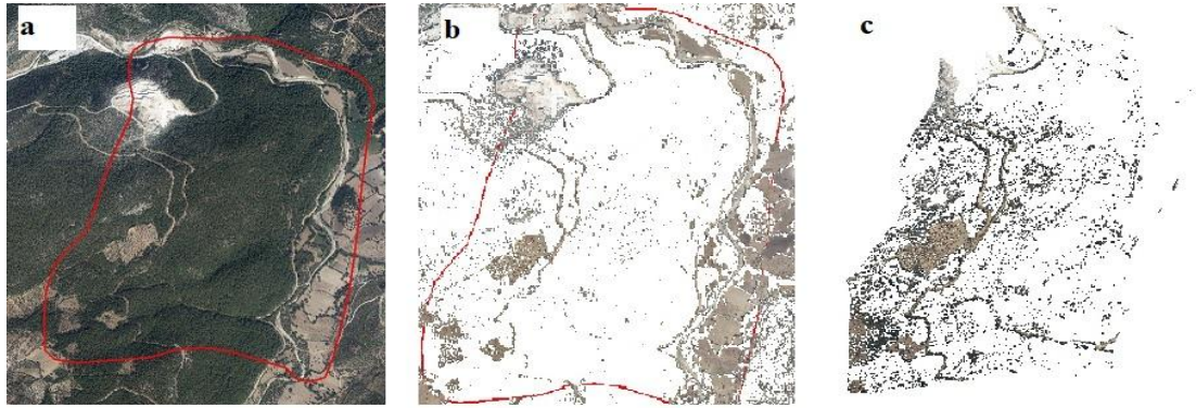
Şekil 4.11 a) Üçüncü çalışma alanı nokta bulutu, b) NDVI değerleri ile filtrelenmiş görünümü, c) CSF algoritması ile filtrelenmiş görünümü.
