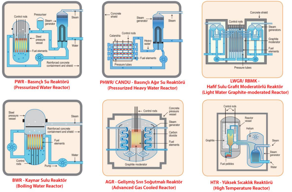
Şekil 2.8 Reaktör tasarımlarına ait çalışma şemaları.
