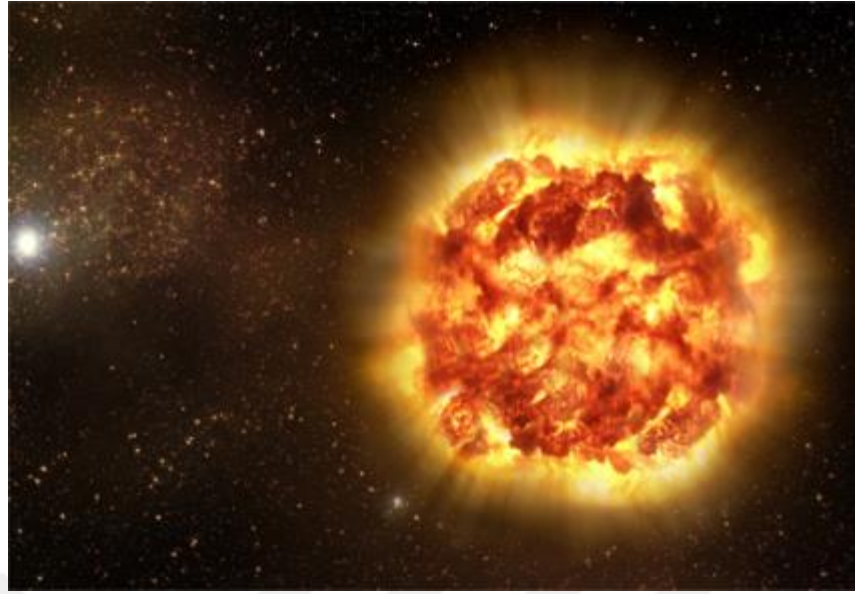
Şekil 2.2 Güneş patlaması.
