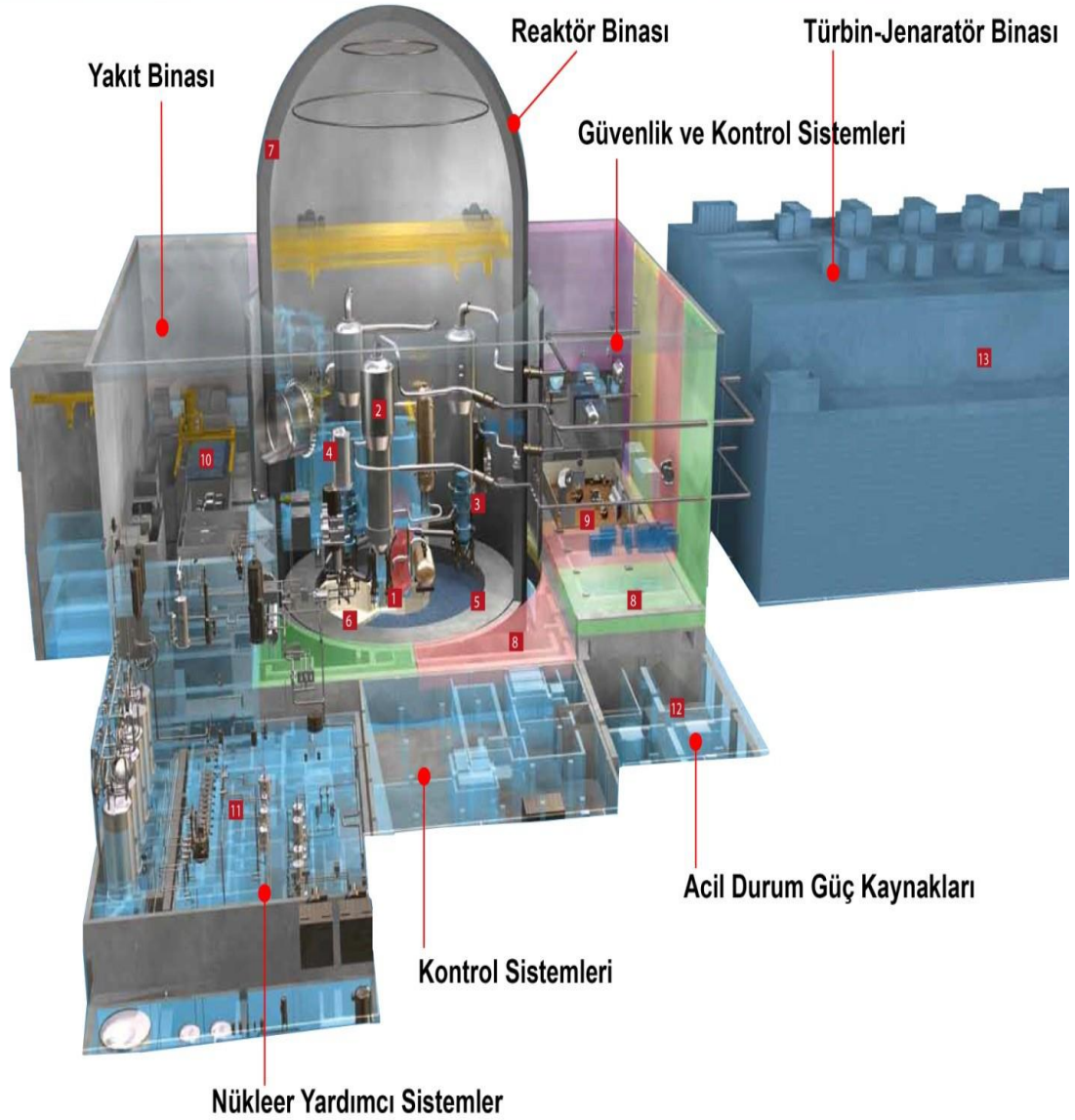
Şekil 2.10 ATMEA-1 tipi reaktörün şeması.
