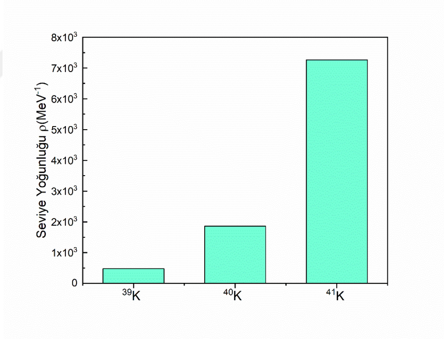
Şekil 15. Deforme K çekirdeklerinin nükleer seviye yoğunlukları
