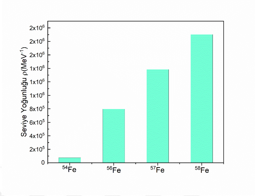
Şekil 9. Deforme Fe çekirdeklerinin nükleer seviye yoğunlukları
