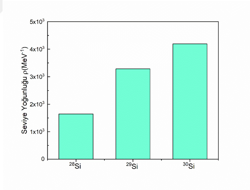
Şekil 14. Deforme Si çekirdeklerinin nükleer seviye yoğunlukları
