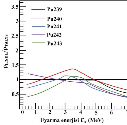
Şekil 3. Pu izotopu için seviye yoğunluğunun TALYS-1.6 ve JENDL-4.0 arasındaki oranı.
