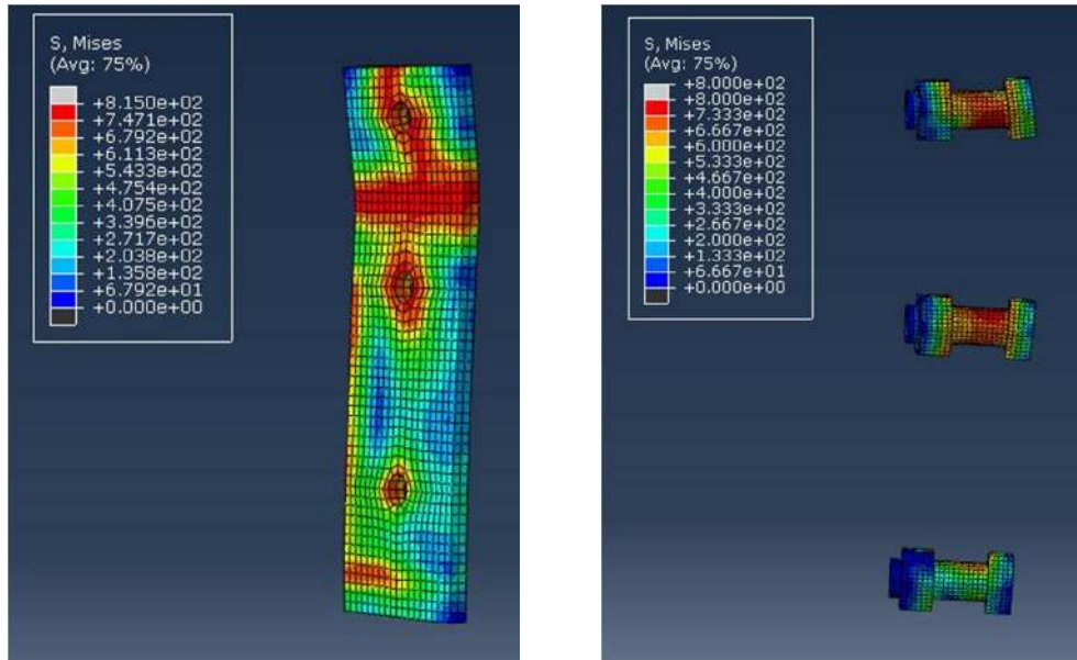
(a)End-Plate S690
