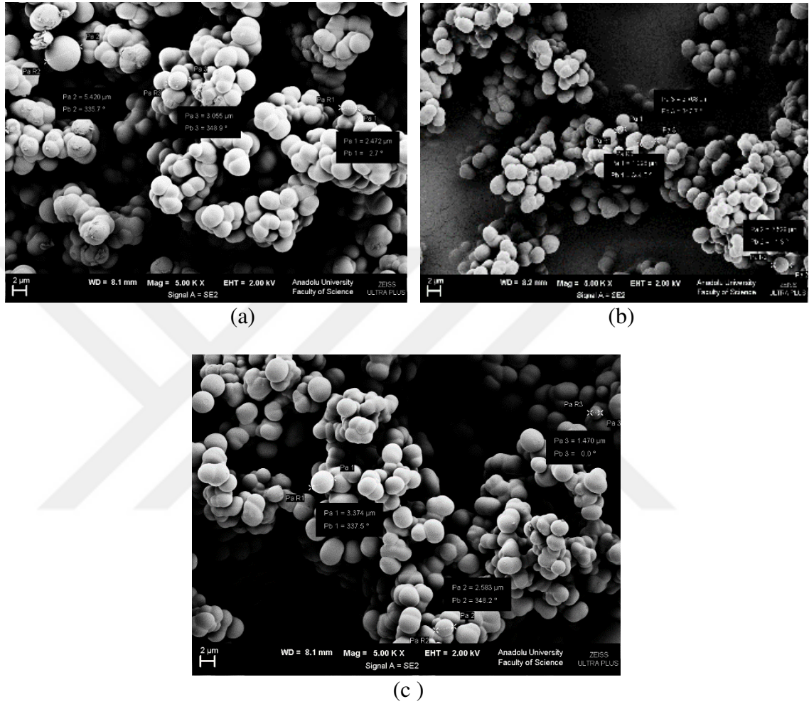
Şekil 5.13. ODNSD-tetramer ters oran denemesi sonucu elde edilen ürünlerin SEM görüntüleri: a) 2:1, b) 3:1, c) 4:1.
