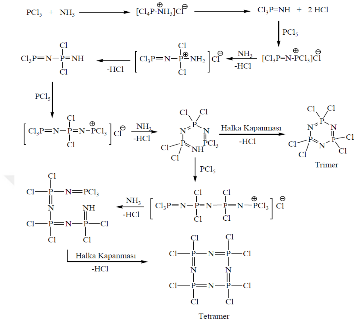
Şekil 2. 10. Halkalı fosfazenlerin sentez mekanizması.
