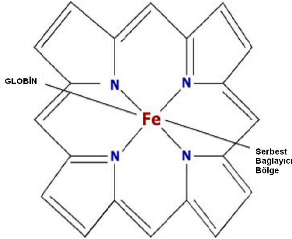
Şekil 13: Miyoglobin (52)
