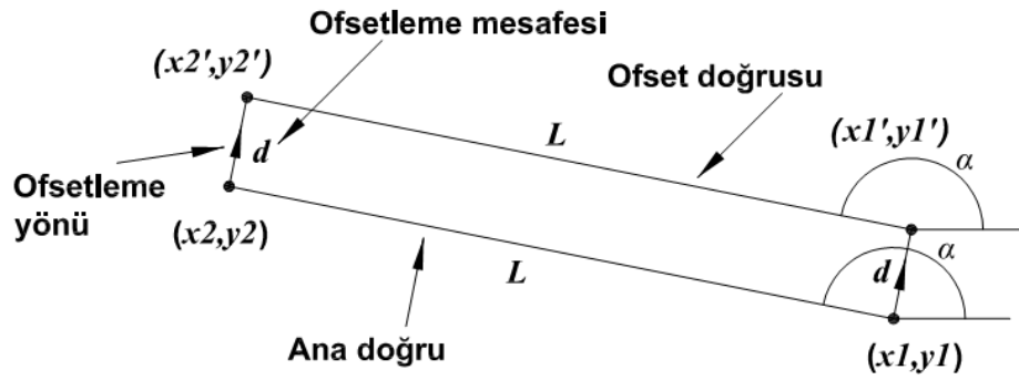
Şekil 4.8. Doğrunun ofsetlenmesi
