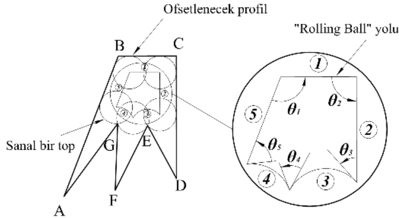
Şekil 2.1. "Rolling Ball" Yöntemi ile ofsetleme süreci [2]
