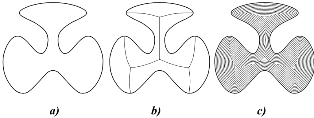
Şekil 2.3. ‘Voronoi’ eğrileri ile gerçekleştirilen Ofsetleme işlemi a) Ofsetlenecek profil b) ‘Voronoi’ eğrilerinin eklenmesi c) Profilin ofsetlenmesi [5]
