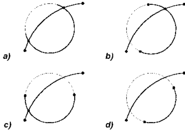
Şekil 4.21. İki yayın kesişim durumları
