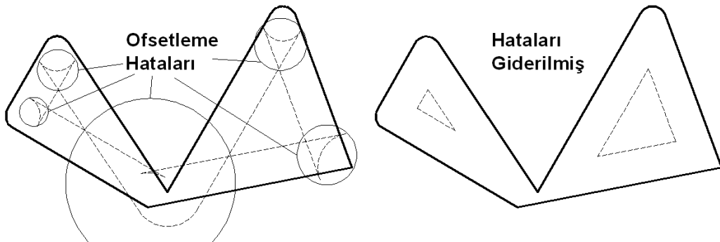
Şekil 4.13. Ofsetleme hataları
