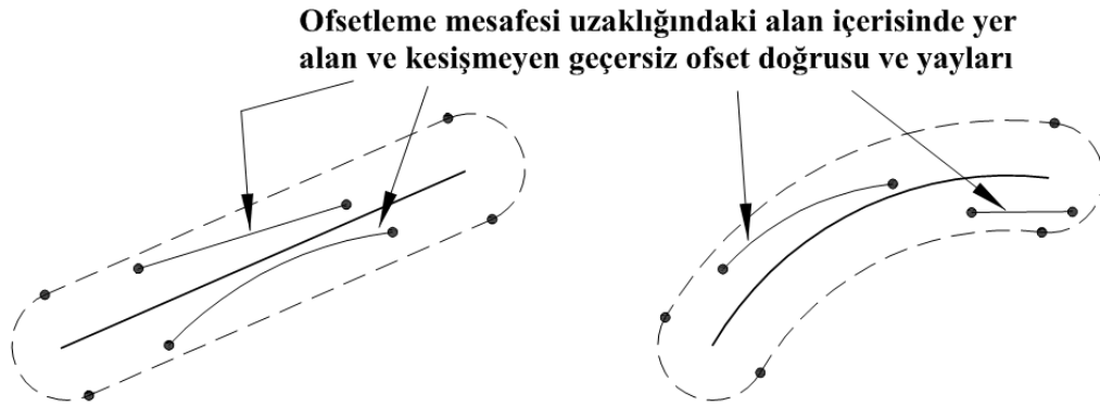
Şekil 4.28. Kesişmeyen ofset unsurları
