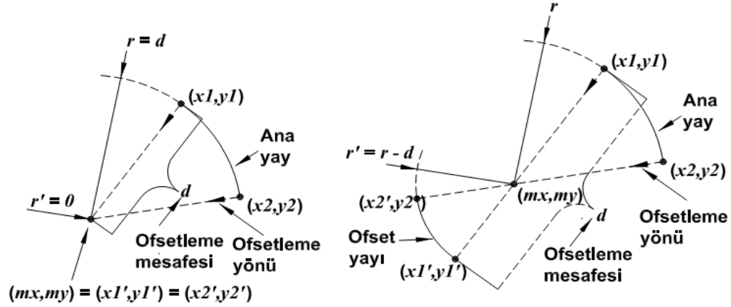
a) d = r iken yayın içe ofsetlenmesi
