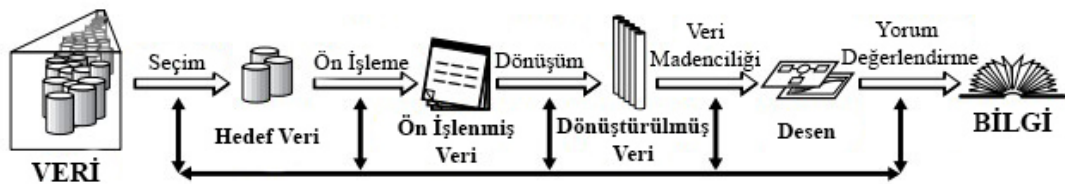
Şekil 1.1. KDD süreci [6]
