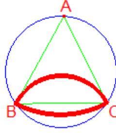
Şekil 4.9: Üçgenin İç Teğet Merkezinin Geometrik yeri
