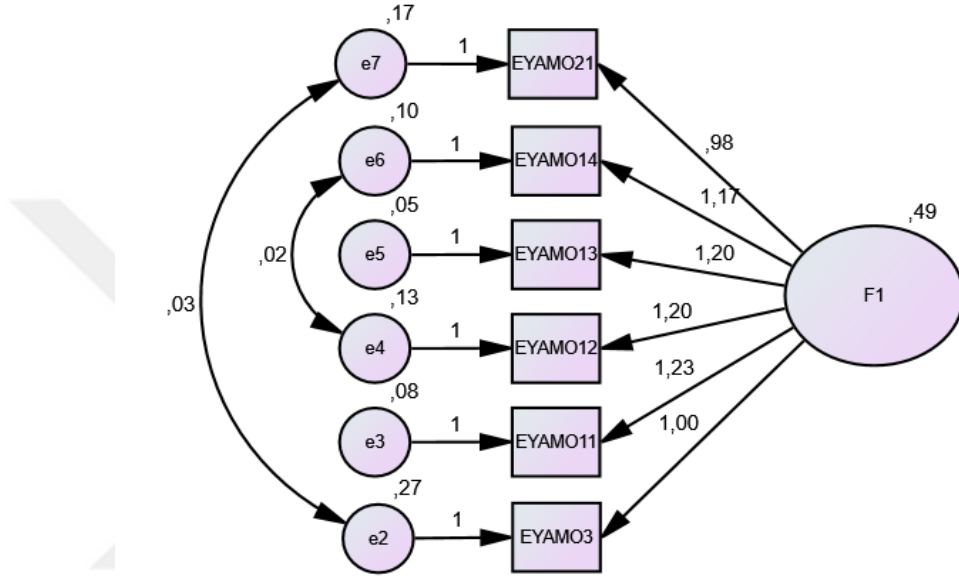
Şekil 7. Algısal Mobbing Ölçeği DFA Sonuçları
