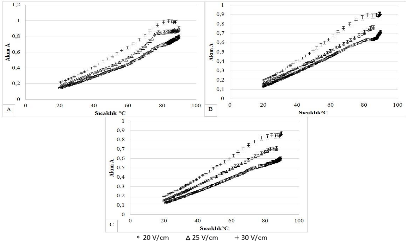
Şekil 4.2. Farklı işlem koşullarında akıma bağlı sıcaklık grafiği (A: 1:20, B: 1:1:40, C: 1:60)
