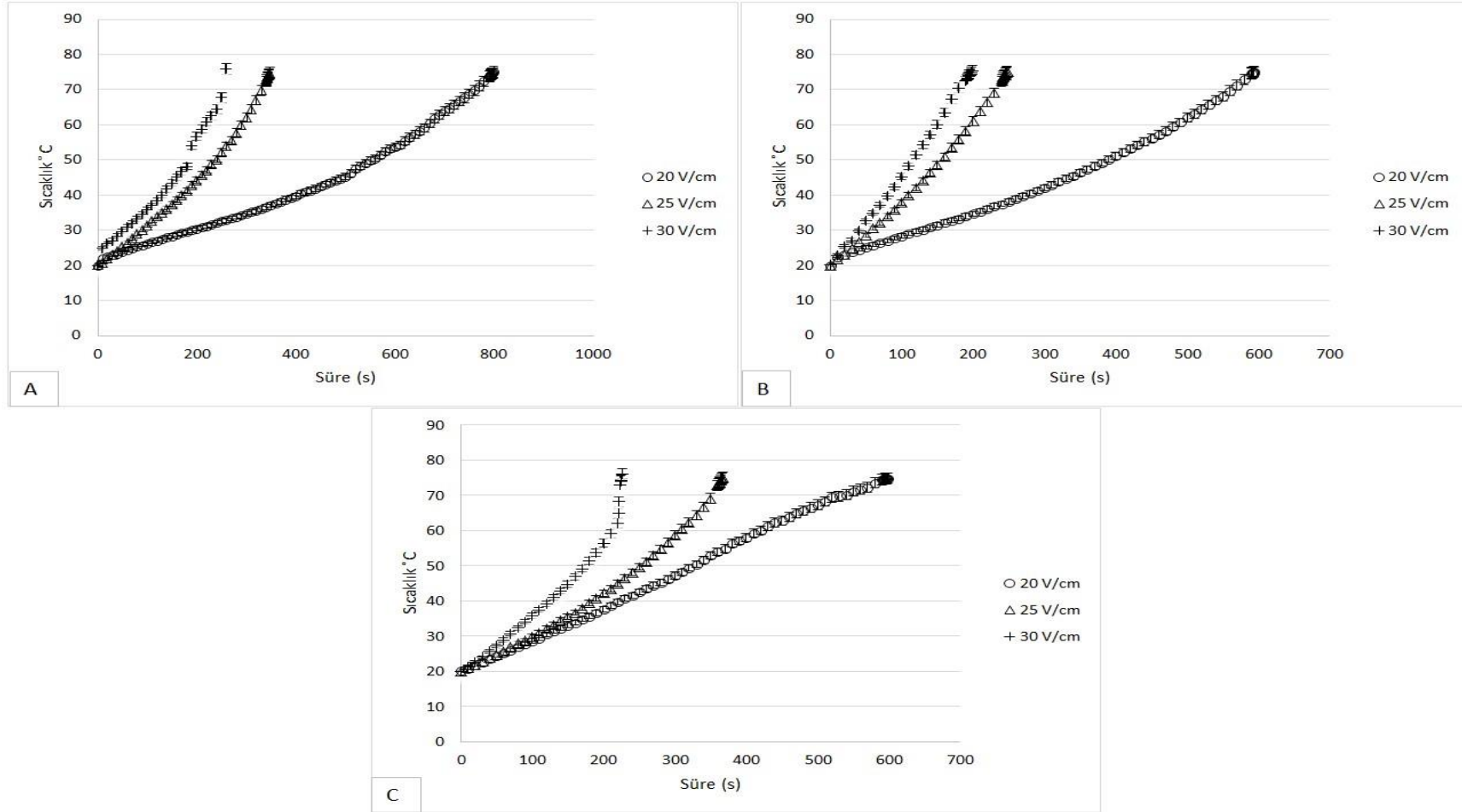
Ek Tablo 6A. Farklı işlem koşullarda ohmik ısıtma işleminde zamana bağlı sıcaklık grafiği (A: 1:20, B1:1:40, C: 1:60/ 75° C)
