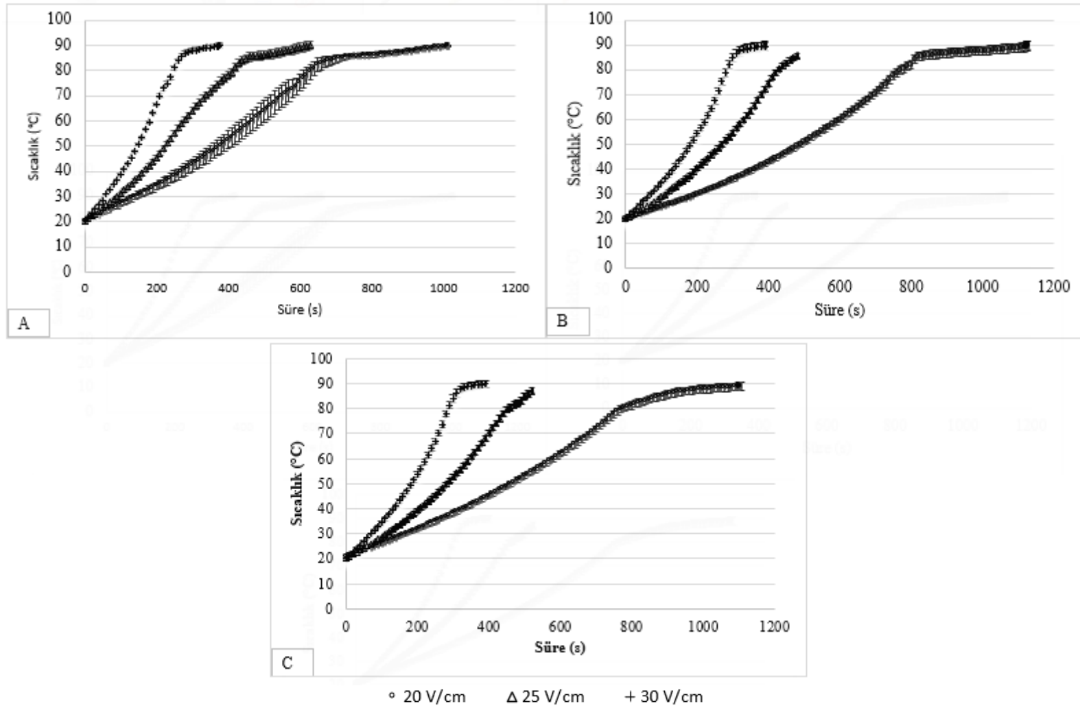
Şekil 4.1. Farklı işlem koşullarda ohmik ısıtma işleminde zamana bağlı sıcaklık grafiği (A: 1:20, B: 1:1:40, C: 1:60)
