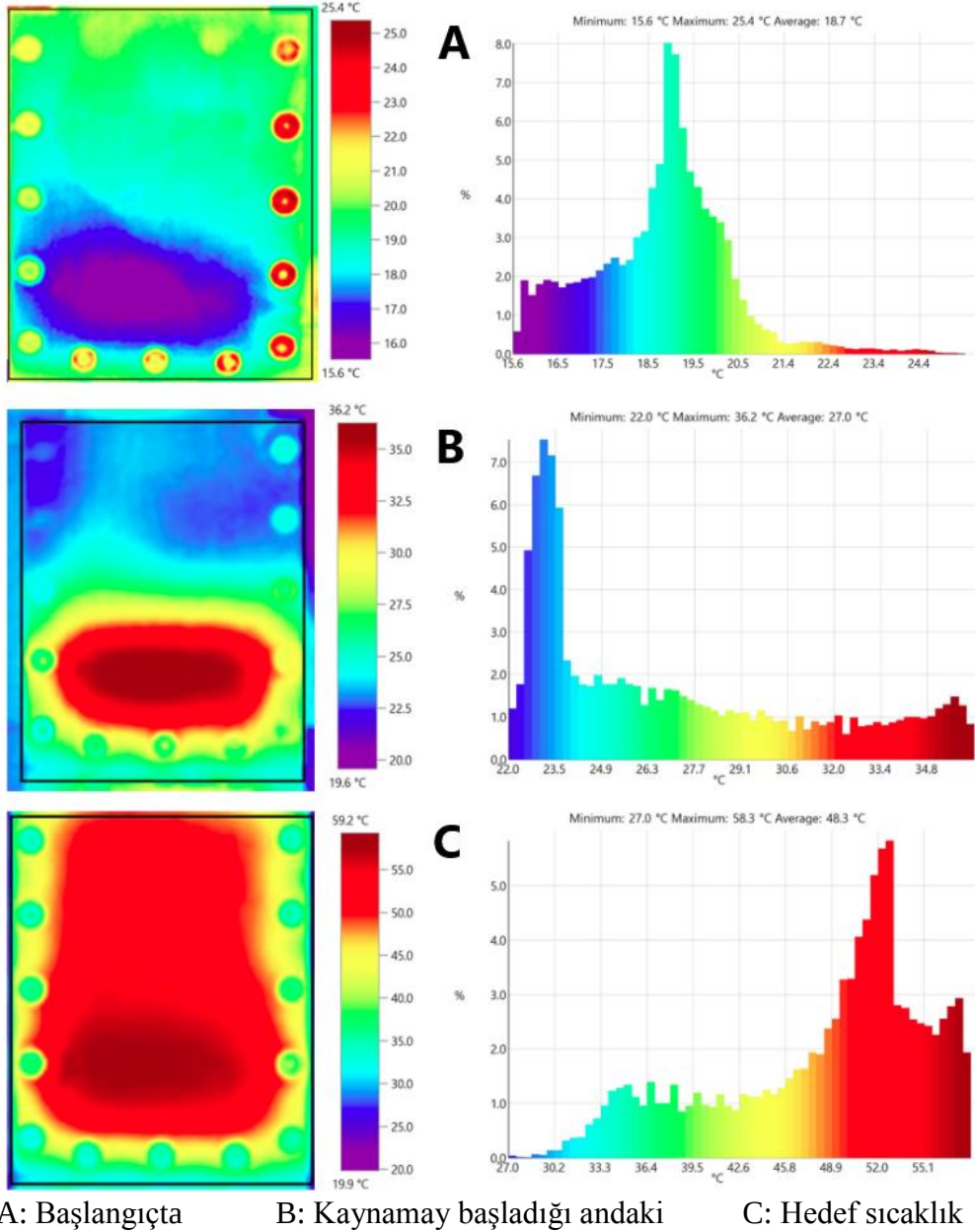
Şekil 4.4. Sisteme ait temassız sıcaklık ölçüm görüntüleri ve sıcaklık dağılımları
