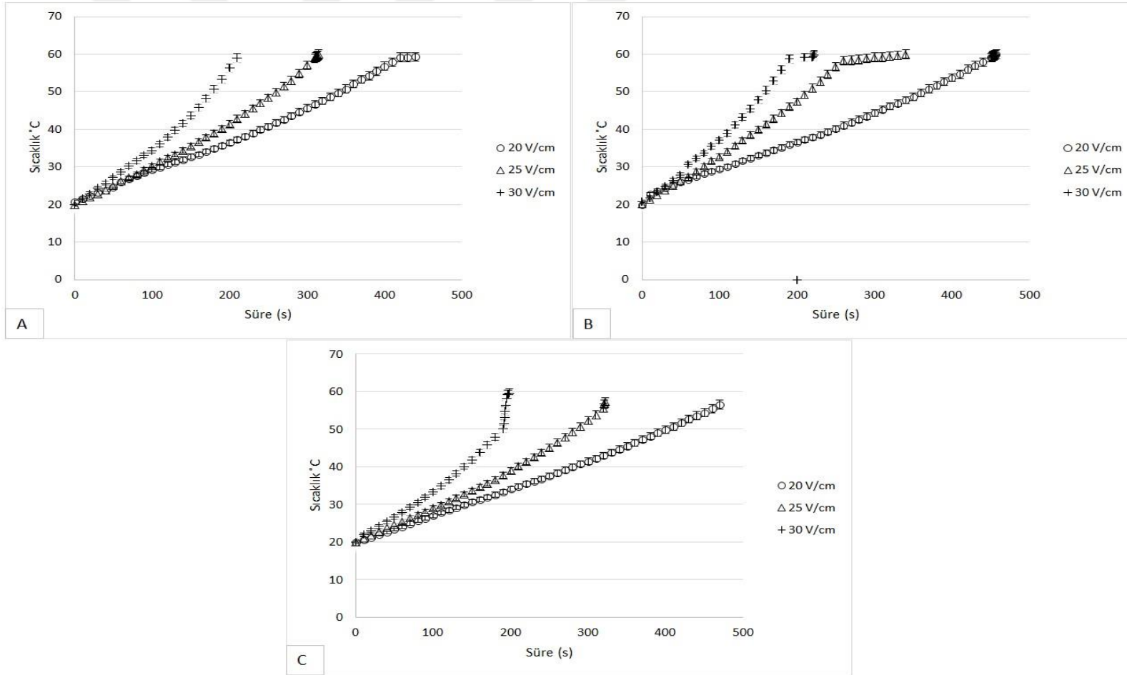
Ek Tablo 5A. Farklı işlem koşullarda ohmik ısıtma işleminde zamana bağlı sıcaklık grafiği (A: 1:20, B1:1:40, C: 1:60/ 60° C)
