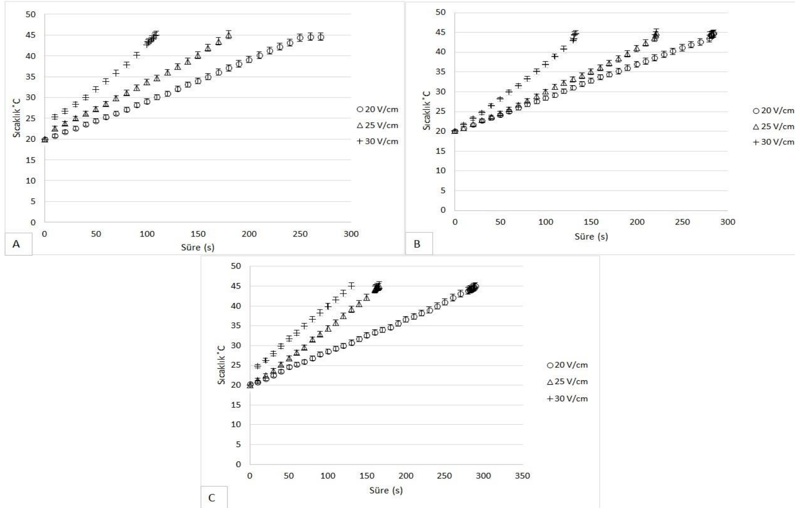
Ek Tablo 4A. Farklı işlem koşullarda ohmik ısıtma işleminde zamana bağlı sıcaklık grafiği (A: 1:20, B1:1:40, C: 1:60/ 45° C)
