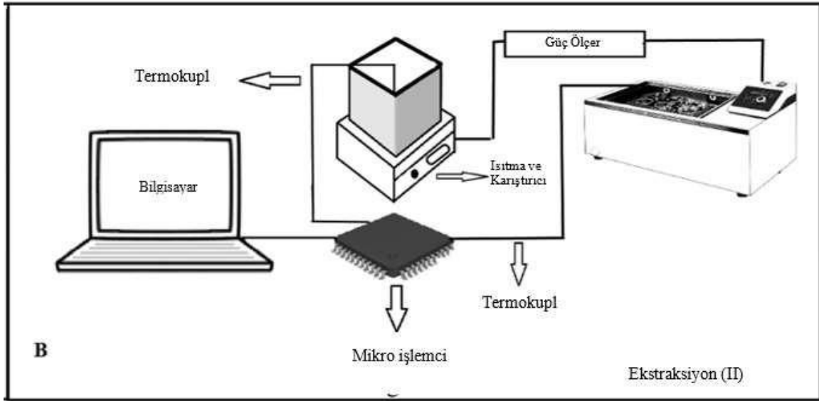
Şekil 3.1. Ohmik ısıtma destekli (A) ve geleneksel ekstraksiyon (B) işlemine ait şematik gösterimi
