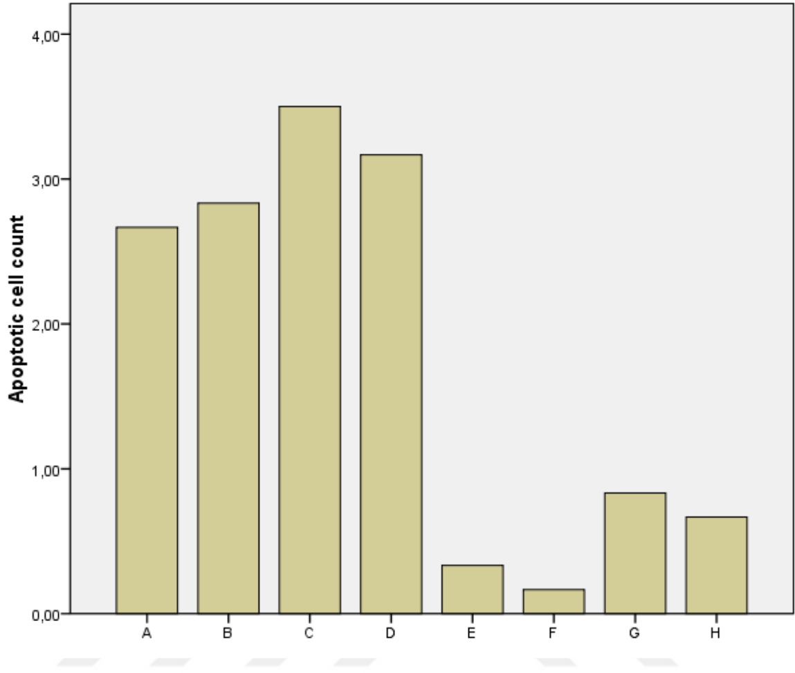
Şekil 4.4.1. : Grup-A-H’de apoptotik hücrelerin kantitatif analizi
