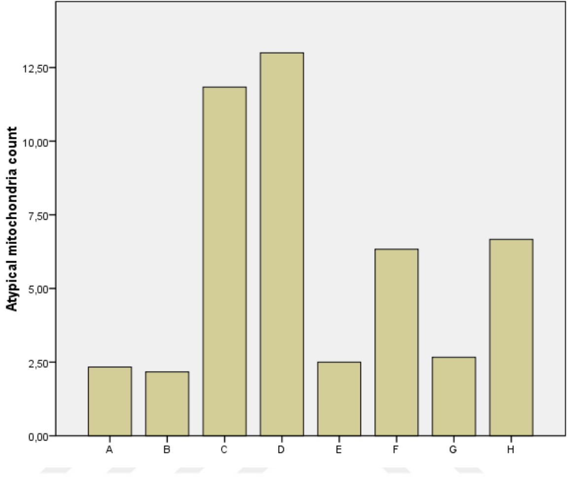
Şekil 4.3.2. : Grup-A-H’de elektron mikroskopi ile atipik mitokondrilerin kantitatif analizi
