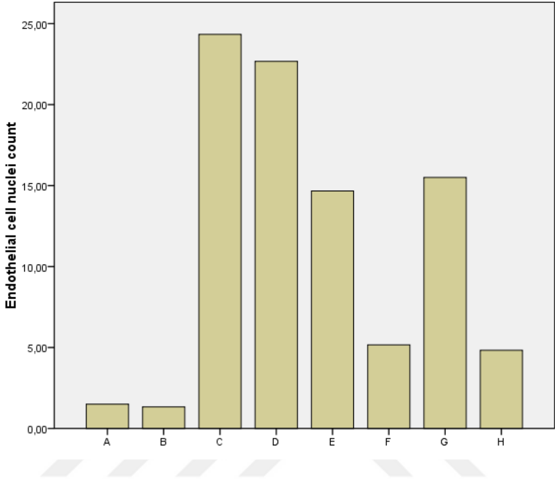
Şekil 4.1.2. : Grup-A-H’de ışık mikroskopi ile neovaskülarizasyonun kantitatif analizi
