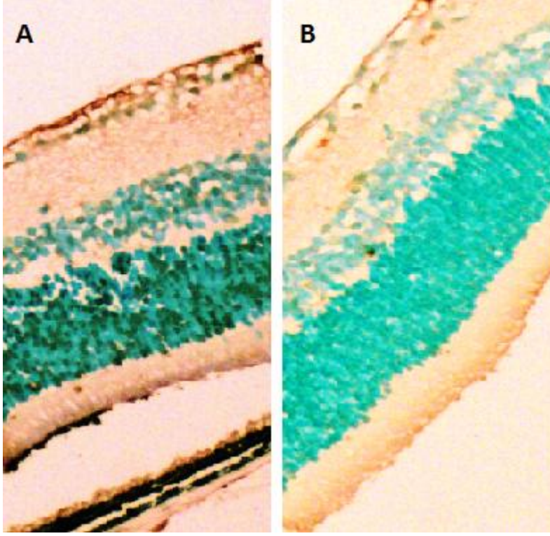
Şekil 4.4.2. : TUNEL tekniği ile apoptotik hücrelerin analizi
