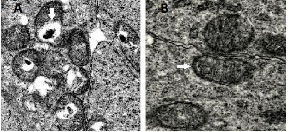
Şekil 4.3.1. : Elektron mikroskopi kesitleri
