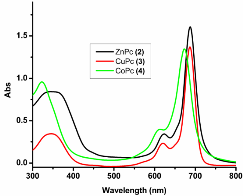
Şekil 4.3. Sentezlenen (2), (3) ve (4) ftalosiyeninlerinin UV-Vis spektrumu.
