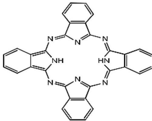
Şekil 2.6. Metalsiz ftalosiyanin Metalsiz ftalosiyanin.
