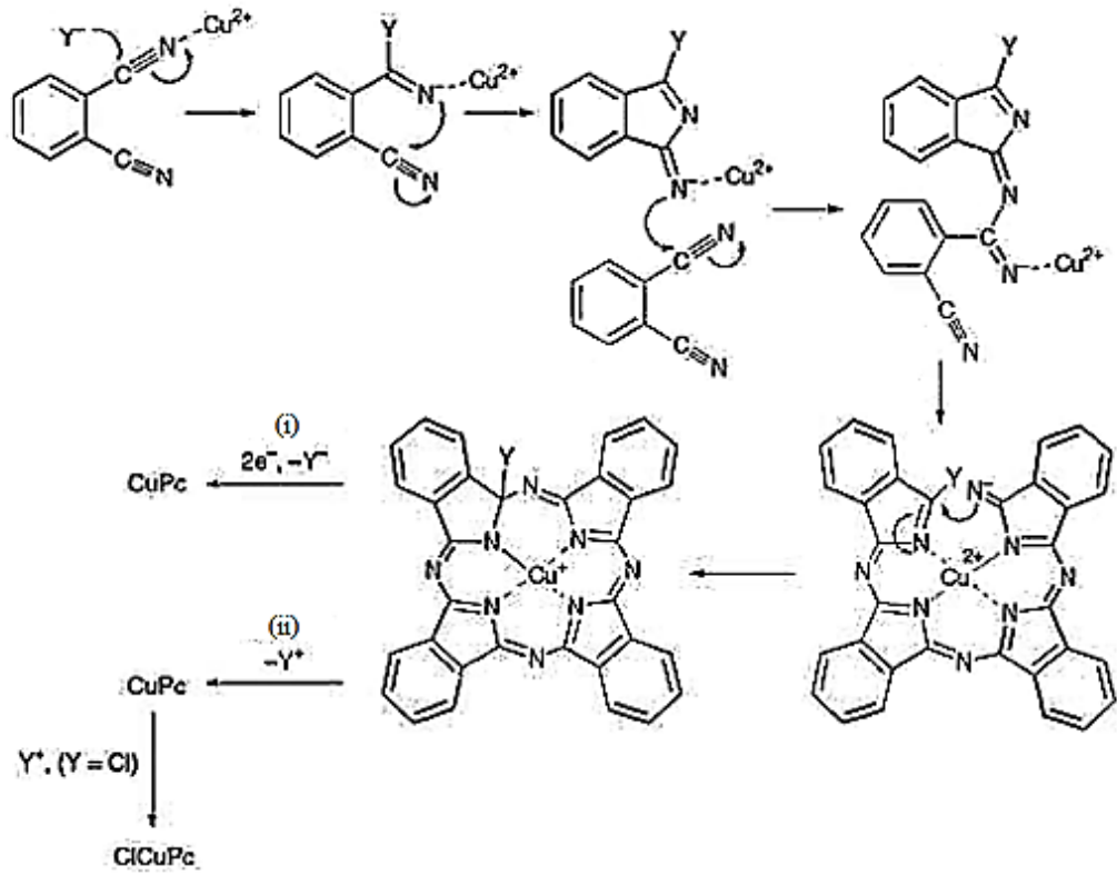
Şekil 2.18. Metalli ftalosiyenin oluşma mekanizması.
