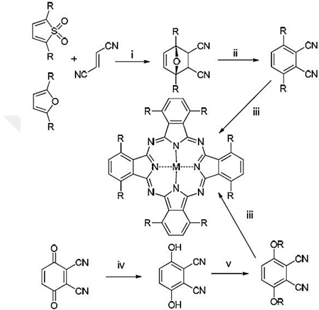
Şekil 2.21. Nonperiferal okta-substitue ftalosiyanın sentezi.
