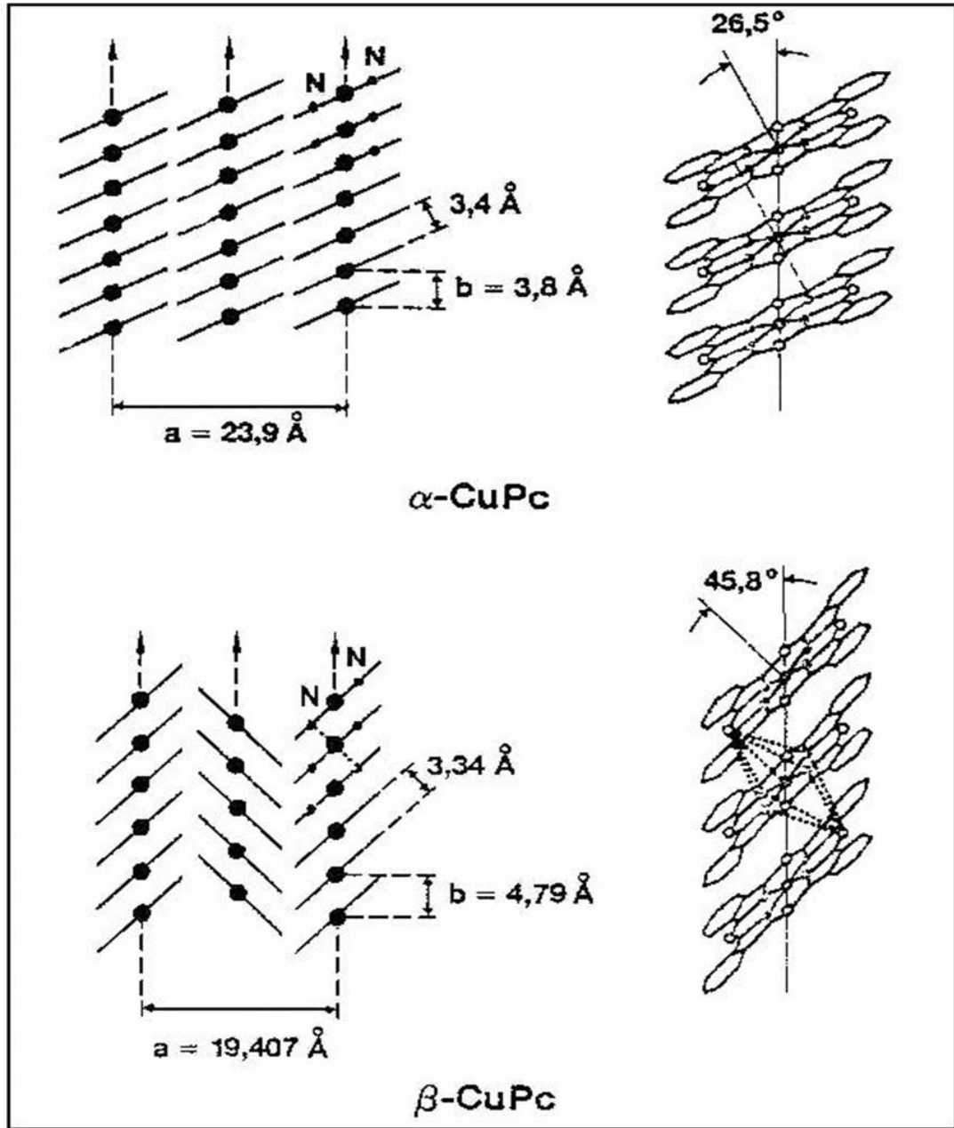
Şekil 2.13. Metalli ftalosiyeninlerde kristal yapıların şematik gösterimi.
