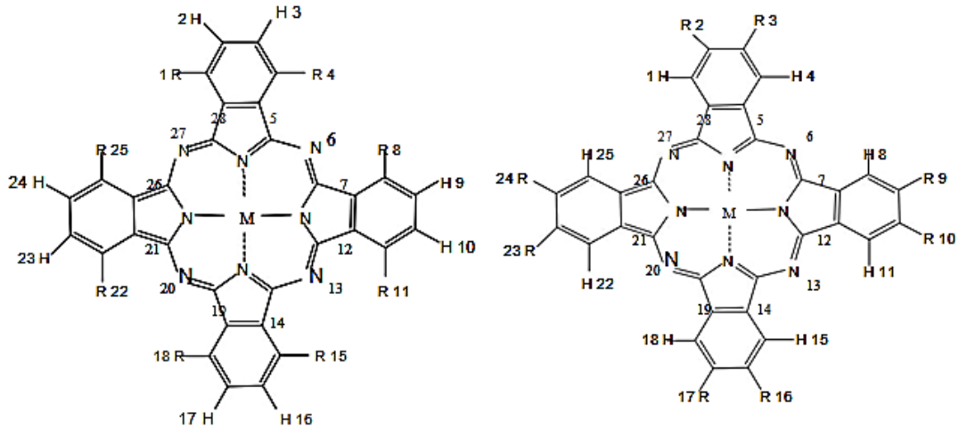
Şekil 2.11. 1,4-süstitüe Ftalosiyanin; 2,3- süstitüe Ftalosiyanin.
