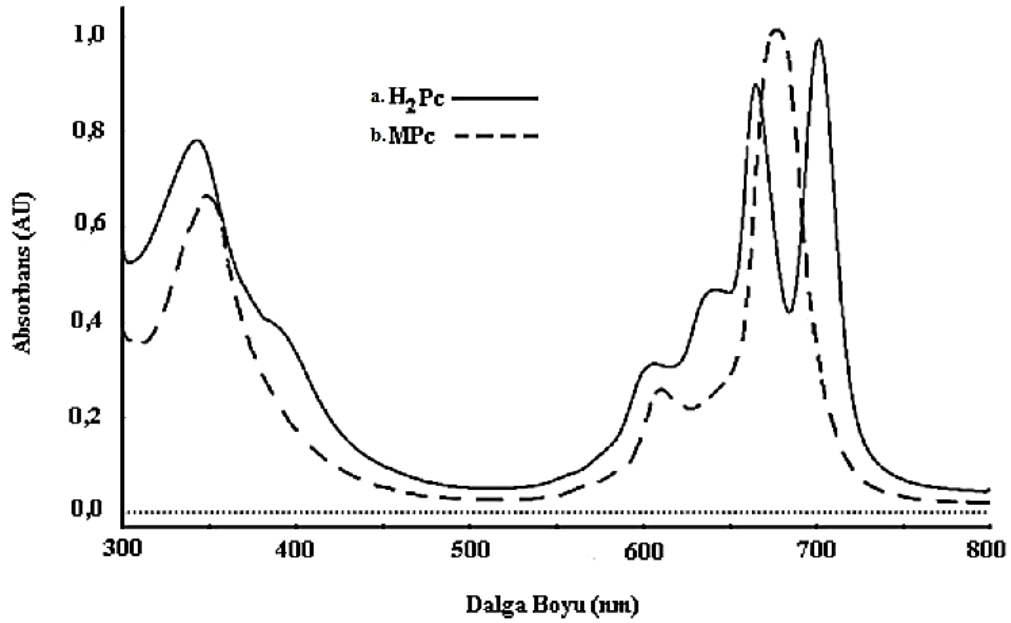
Şekil 2.24. a. Metalli ftalosiyanin UV-vis b. Metalsiz ftalosiyanin UV-vis.
