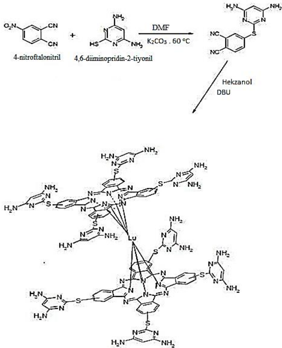
Şekil 2.23. Sandviç ftalosiyenin sentezi.
