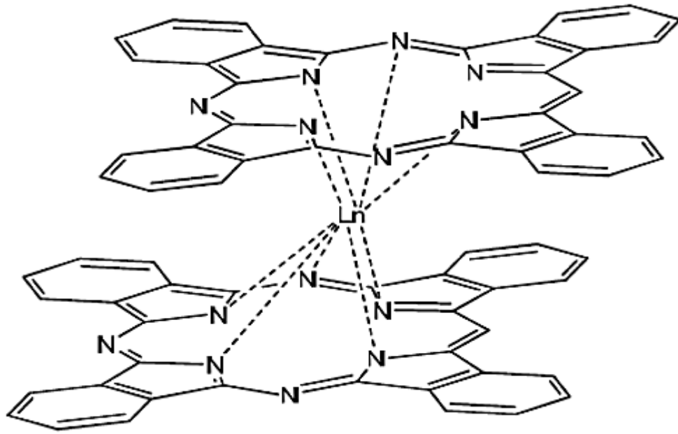
Şekil 2.22. Sandviç ftalosiyenin örneği.
