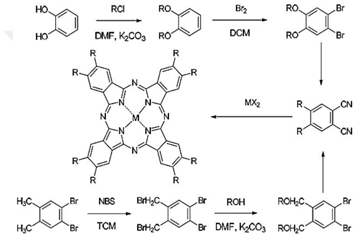
Şekil 2.20. Oktasüstitüe ftalosiyenin sentezi.
