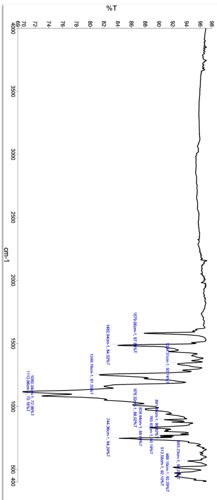
EK 4: (2) Maddesine ait IR spektrumu
