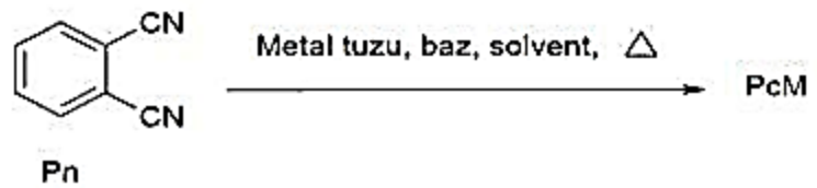
Şekil 2.14. Ftalosiyanın genel elde edilme yolları [47].
