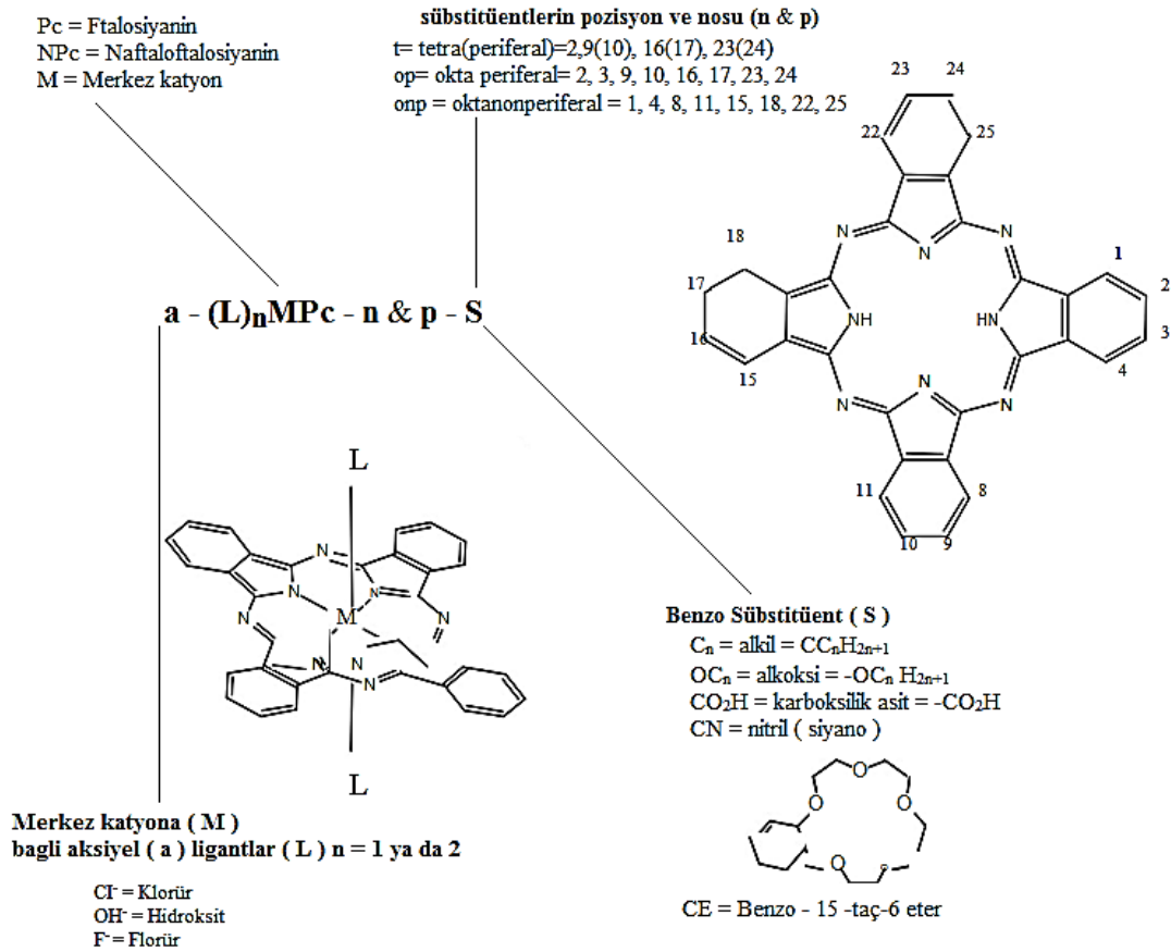
Şekil 2.12. Ftalosiyaninlerin adlandırılması.
