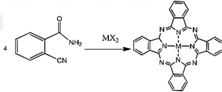
Şekil 2.1. Ftalosiyanin sentez reaksiyonu.
