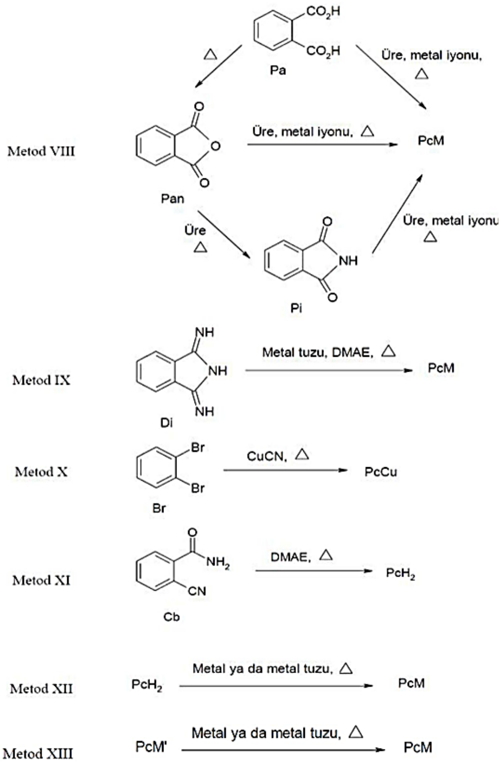
Şekil 2.15. Ftalosiyeninlerin genel elde edilme yolları (Devamı).
