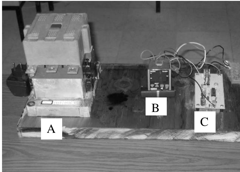
Őekil 4.2. Numunelerin a ma-kapama deneylerinin yapıldıđı deney d zeneđi
