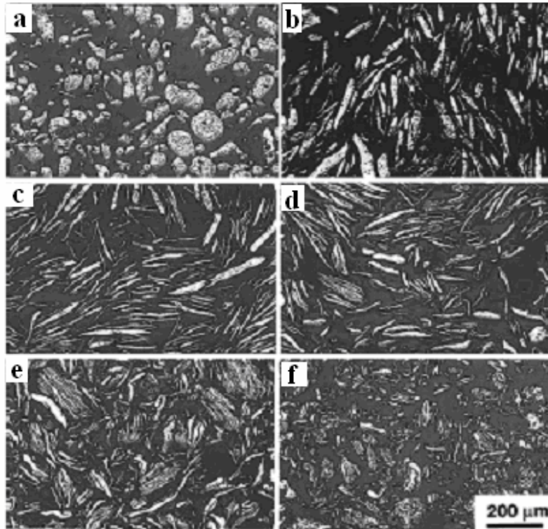
Şekil 2.3. 6061 Alüminyum alaşımında grafit dispersiyonu sağlamak için uygulanan mekanik alaşımla işlemi boyunca toz morfolojisi değişimi (a) Alaşımlamadan önce, (b) 20 saat, (c) 30 saat, (d) 40 saat, (e) 60 saat, (f) 70 saat [12].
