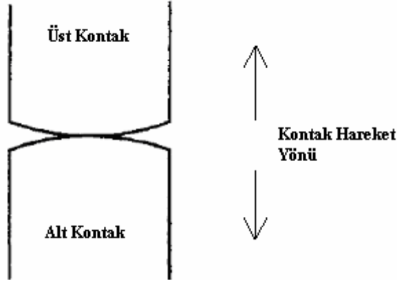
Şekil 3.4. Kontak Açma esnasında meydana gelen akım yoğunluğu [17]
