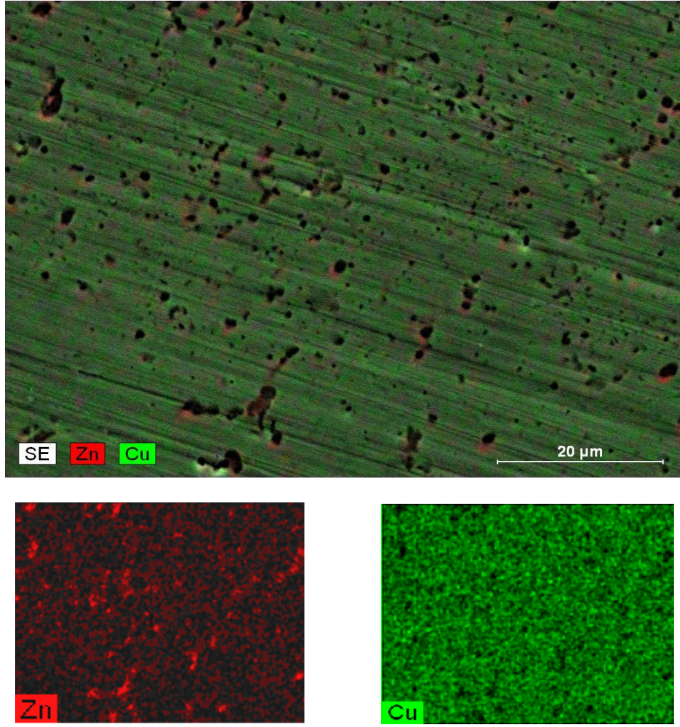
Şekil 5.6. % 4 ZnO ilaveli 5 saat mekanik alaşımlanmış numunenin element dağılım haritası
