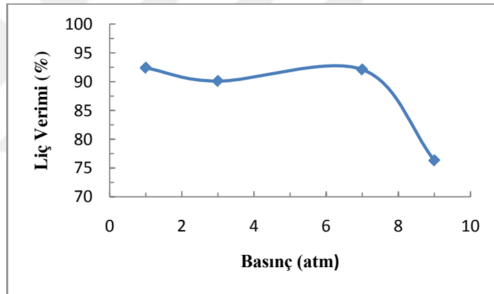
Şekil 4.25. Basıncılı Ortamda H_2O_2 + O_2 Liç Verimi Üzerine Etkisi
