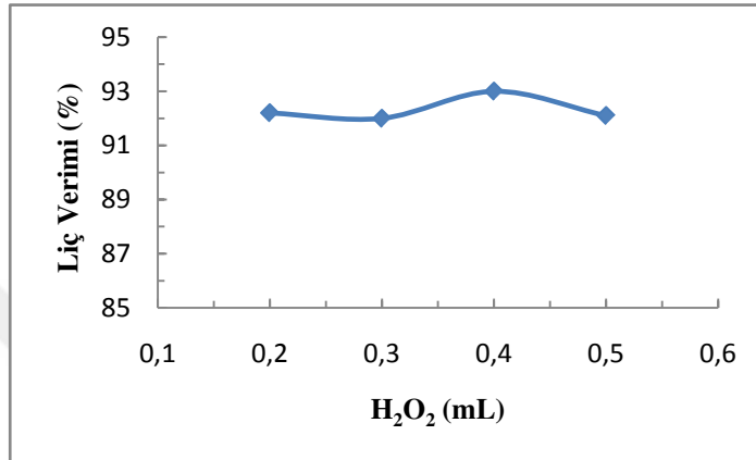
Şekil 4.26. \text{Ca}(\text{OH})_2 'in \text{H}_2\text{O}_2 Ortamında Liç Verimi Üzerine Etkisi
