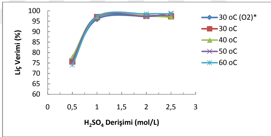
Şekil 4.9. Bakırın Liç Verimi Üzerine \text{Ca}(\text{OH})_2 'in Etkisi
