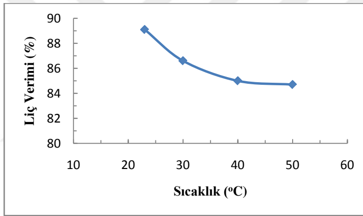
Şekil 4.21. \text{HNO}_3 'in Sıcaklığa Bağlı Olarak Liç Verimi Üzerine Etkisi
