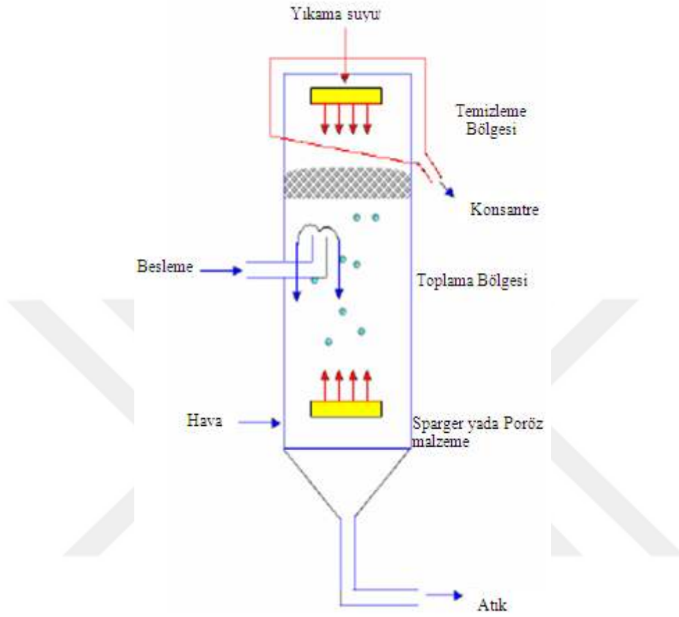
Şekil 1.11. Klasik Kolon Flotasyonu
