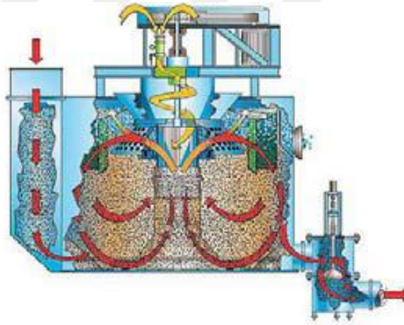
Şekil 1.10. Mekanik Hücre Flotasyonu
