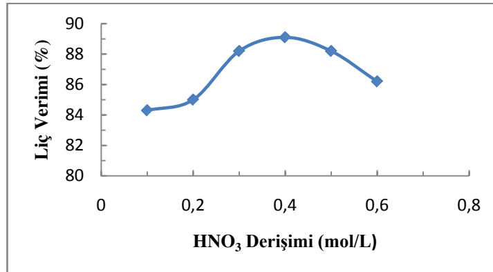
Şekil 4.20. Bakırın Liç Verimi Üzerine Yükseltgen \text{HNO}_3 'in Etkisi
