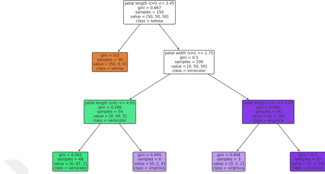
Şekil 3.3. Karar Ağacı Yapısının Görselleştirilmesi
