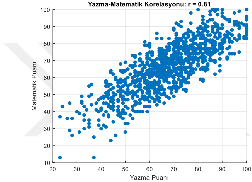
Şekil 4.2. Yazma ve Matematik Skorları Arasındaki İlişki
