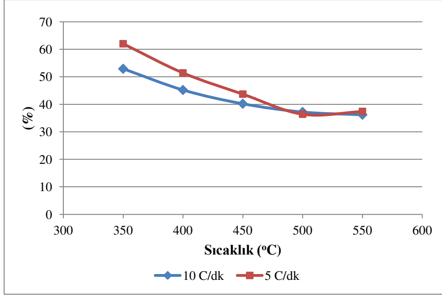
Şekil 4.10. Farklı ısıtma hızlarında otomobil lastiđinden elde edilen karbon siyahı miktarının değışimi
