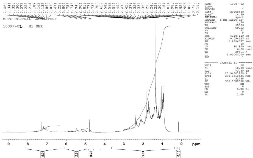
Resim 4.5. Sabit yatak piroliz deneyi ile otomobil lastiğinden elde edilen piroliz yağının 0 - 9 ppm arası ^1\text{H} NMR spektroskopisi
