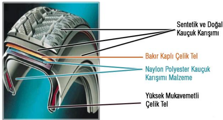
Resim 2.1. Lastiğin yapısı
