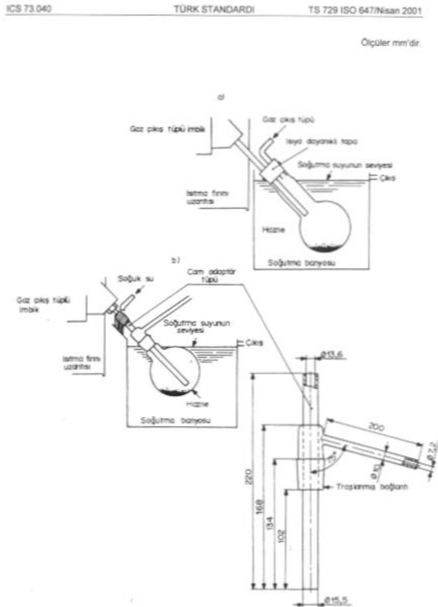
ŞEKİL 2 - Soğutma Banyosunda Haznenin Düzenlenmesi
