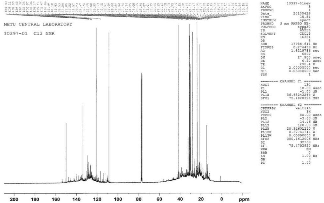
Resim 4.6. Sabit yatak piroliz deneyi ile kamyon lastiğinden elde edilen piroliz yağının ^{13}\text{C} NMR spektroskopisi
