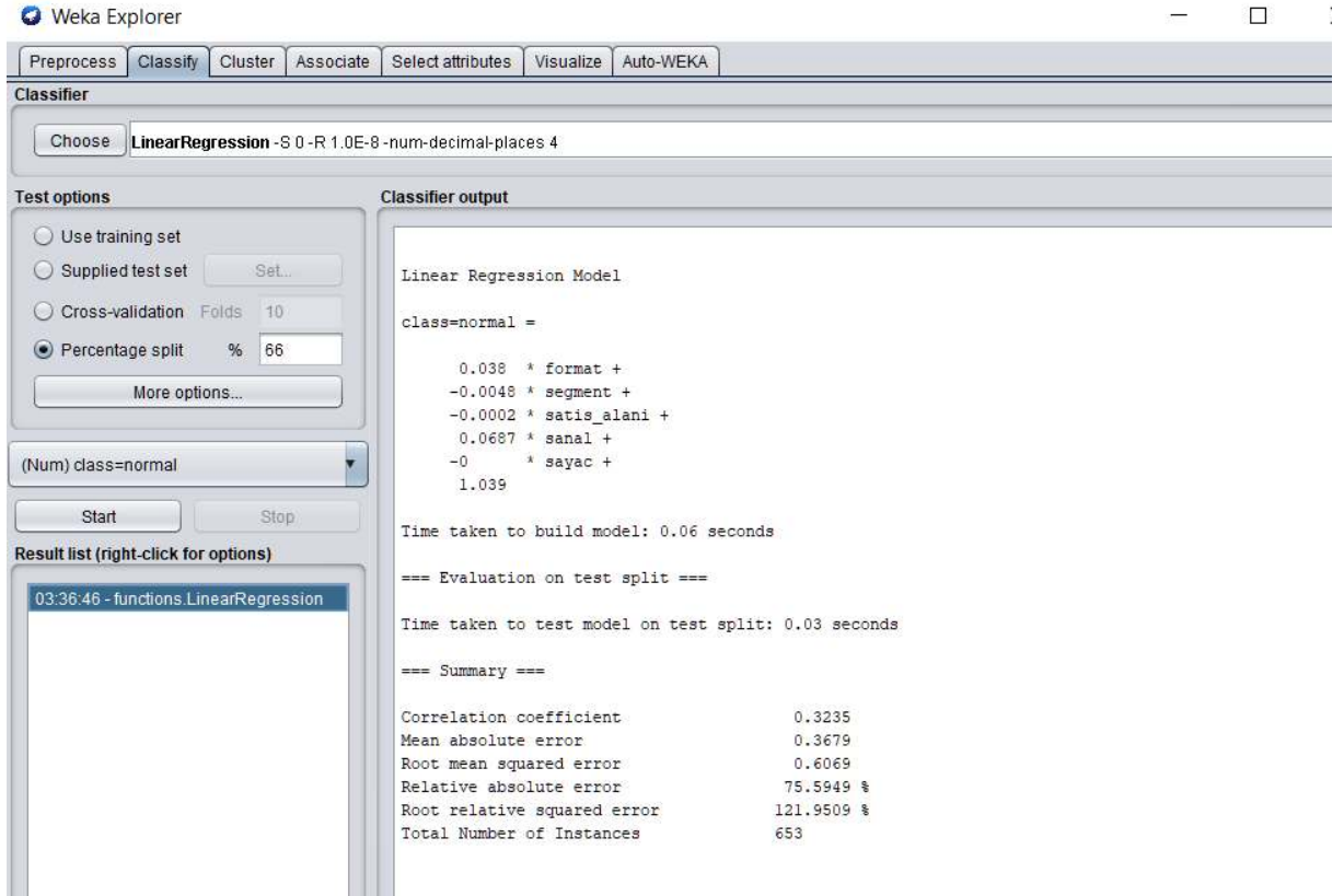
Şekil 23 Lineer Regresyon Çıktısı
