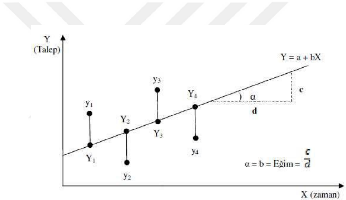
Şekil 3 Regresyon Doğrusu
