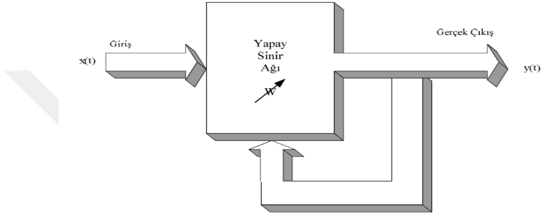
Şekil 19 Gözetimsiz Öğrenme
