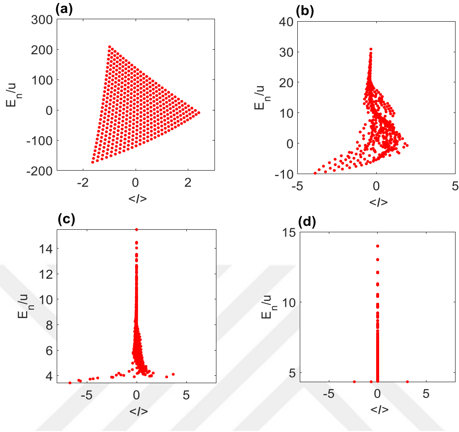
Şekil 4.3: Akımın özdeğerler ile değişimi. N = 30 , \Phi = 0,8\pi , \varepsilon = 1 , J = 0,5 ve (a) u = 0,2 (b) u=2 (c) u=20 (d) u=20000 . Parçacıklar arası etkileşim arttıkça akım sıfıra gitmektedir.
