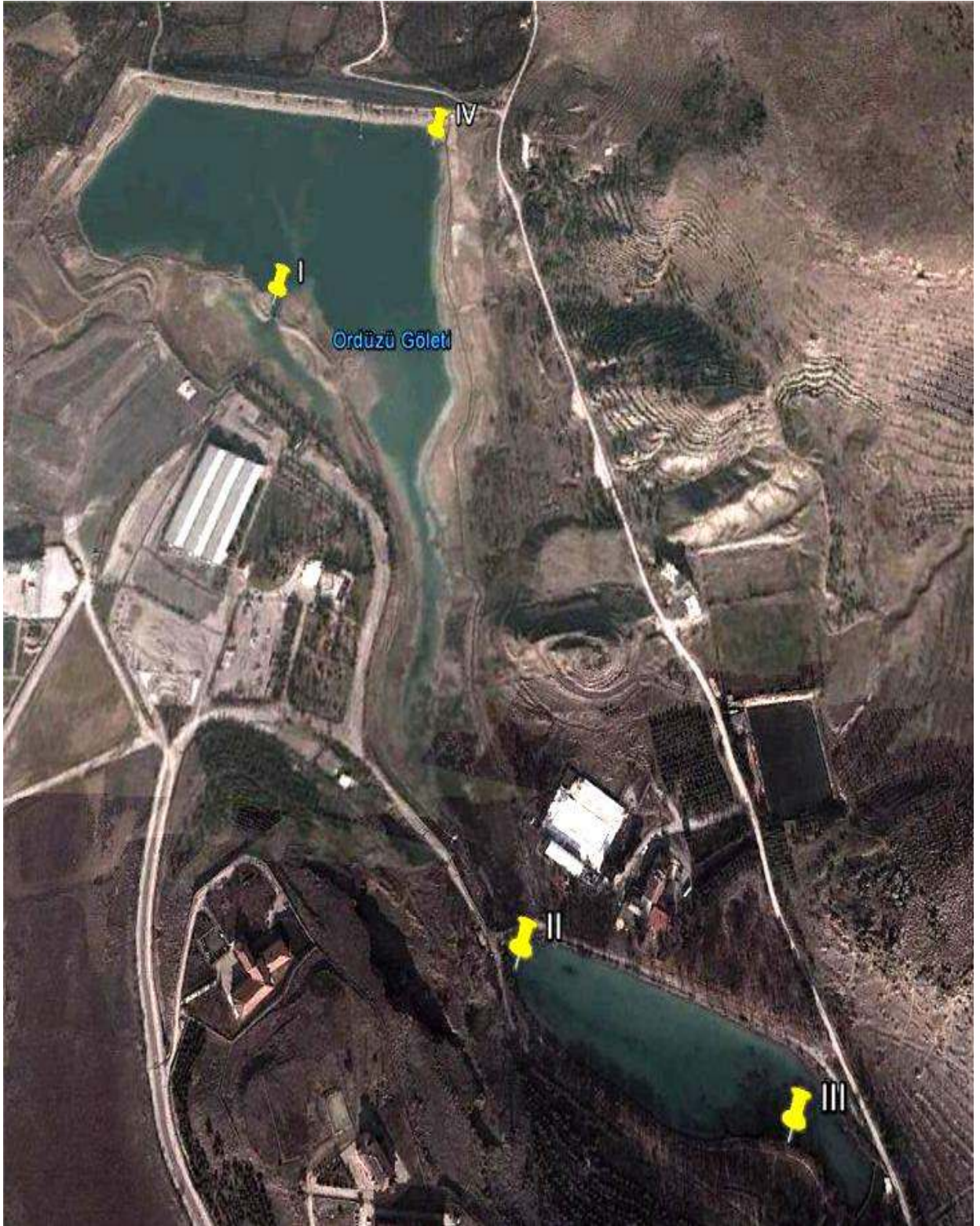
Şekil 2.1. Orduzu Gölü ve Örnekleme İstasyonları
