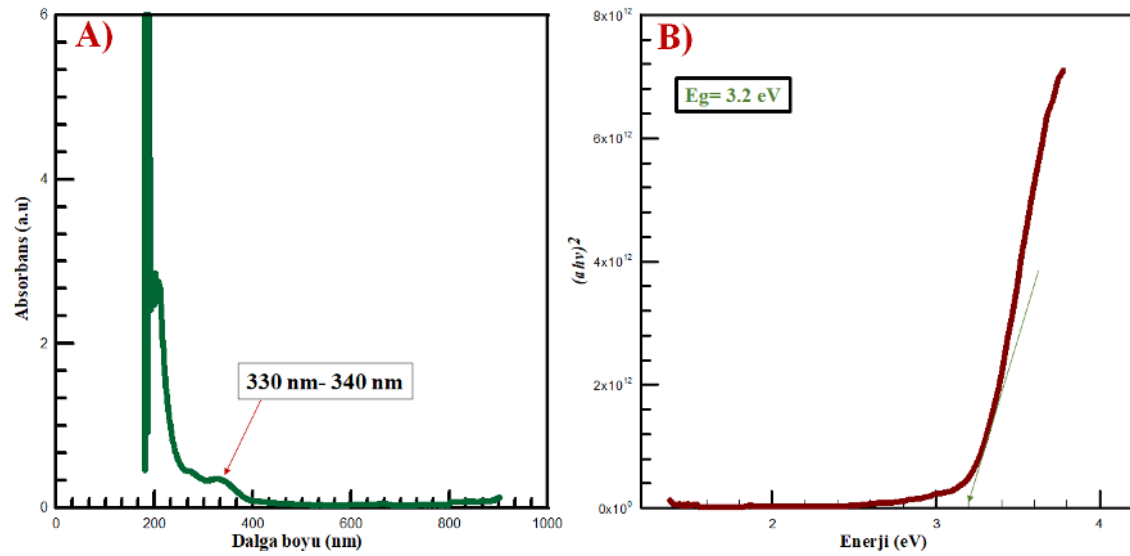
Şekil 4.2. Stachys lavandulifolia bitkisinin a) UV-görünür bölge spektrumu, b) yasak enerji bant aralığı
