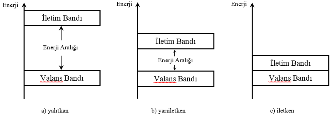
Şekil 2. 2. a) Yalıtkan, b) Yarıiletken, c) İletken enerji diyagramı
