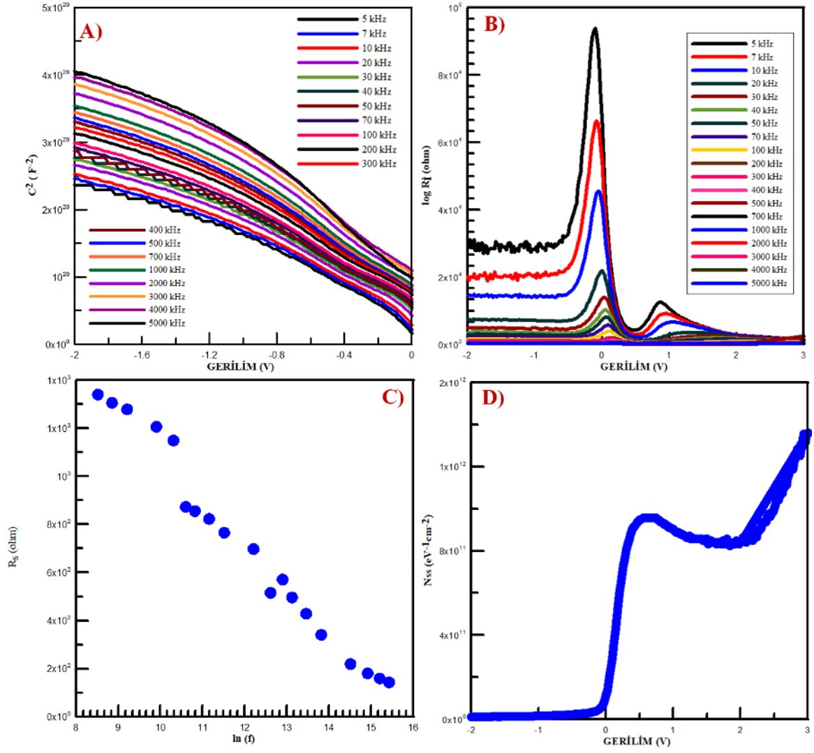
Şekil 4.5 Stachys lavandulifolia arayüzeyli doğrultucu yapısının (-2,+3) volt ve (5-5000) kHz frekans aralığında elde edilen (A) C^2 -V grafiği, (B) düşük- yüksek frekans R_i -V grafiği, (C) R_s -ln(f) grafiği, (d) 5 kHz'de N_{ss} -V grafiği
