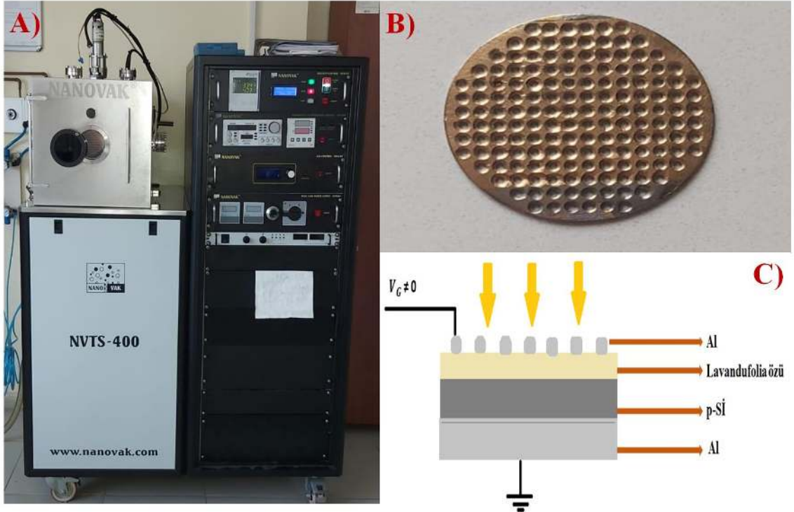
Şekil 3.3. a-) Termal buharlaştırma cihazı (nanovak NVTS-400), b-) 1mm nokta kontak maske, c-) Lavandufolia arayüzeyli diyot şeması
