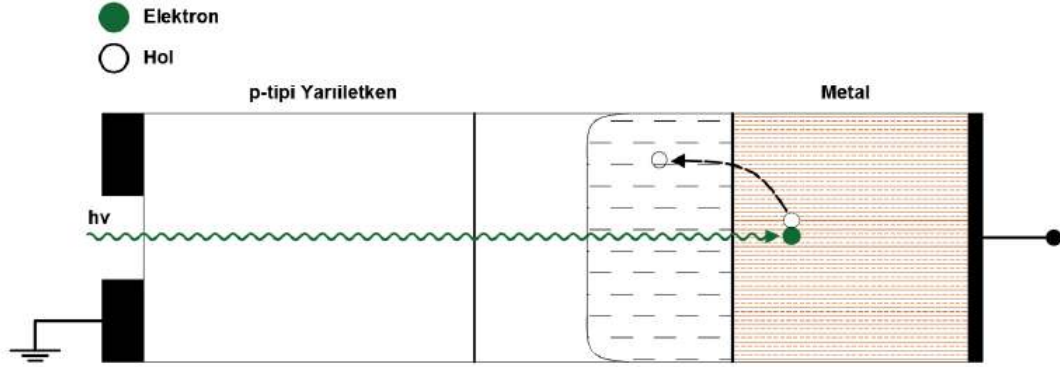
Şekil 2.6. Schottky fotodiyot yapısı
