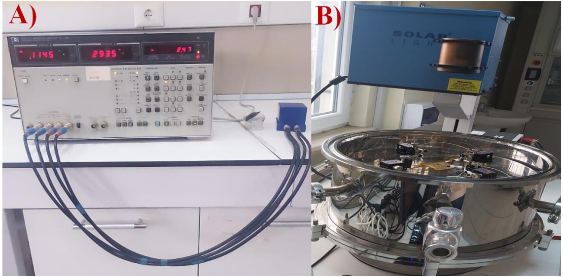
Şekil 3.6. (a) Frekansa bağlı C-V analiz cihazı 4192A model YHP (b) Akım-Gerilim analiz solar simülatörü
