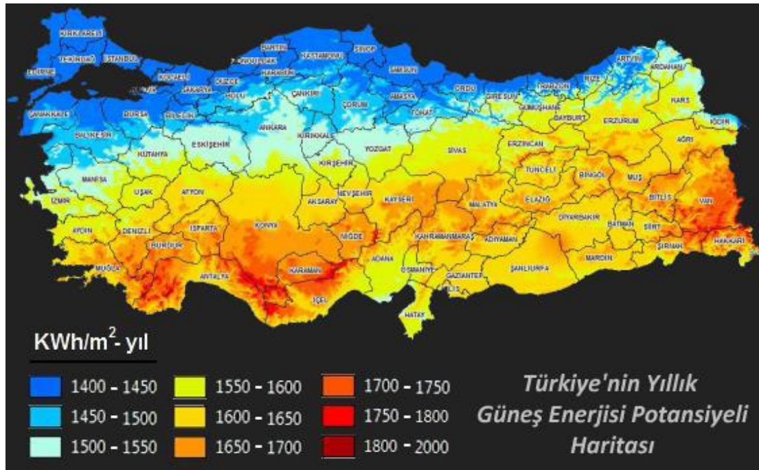
Şekil 2.1. Türkiye'nin yıllık güneş enerjisi potansiyeli haritası
