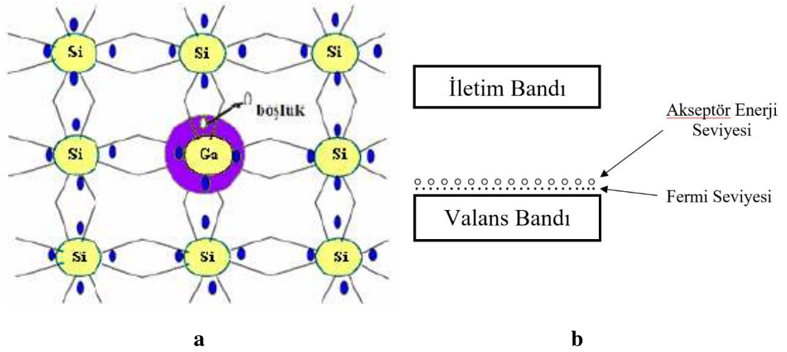
Şekil 2.4. a) Ga katkılı silisyum kristali, b) p-tipi yarıiletkenlerin band yapısı
