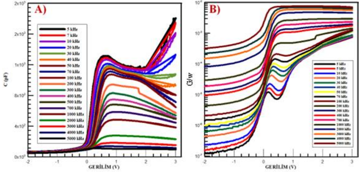
Şekil 4.4. Stachys lavandulifolia arayüzeyli doğrultucu yapısının (-2,+3) volt ve (5-5000) kHz frekans aralığında elde edilen (A) düşük-yüksek C-V grafikleri, (B) düşük-yüksek G/w-V grafikleri
