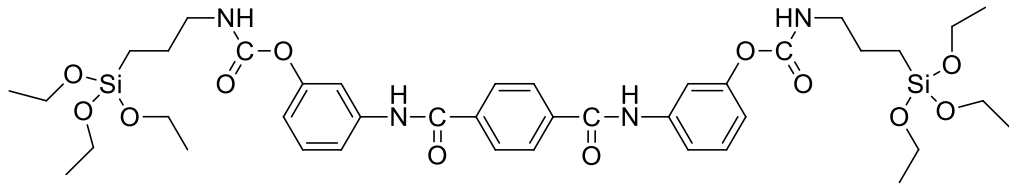
Şekil 3 : Alkoksisilan modifiye makromonomer.
