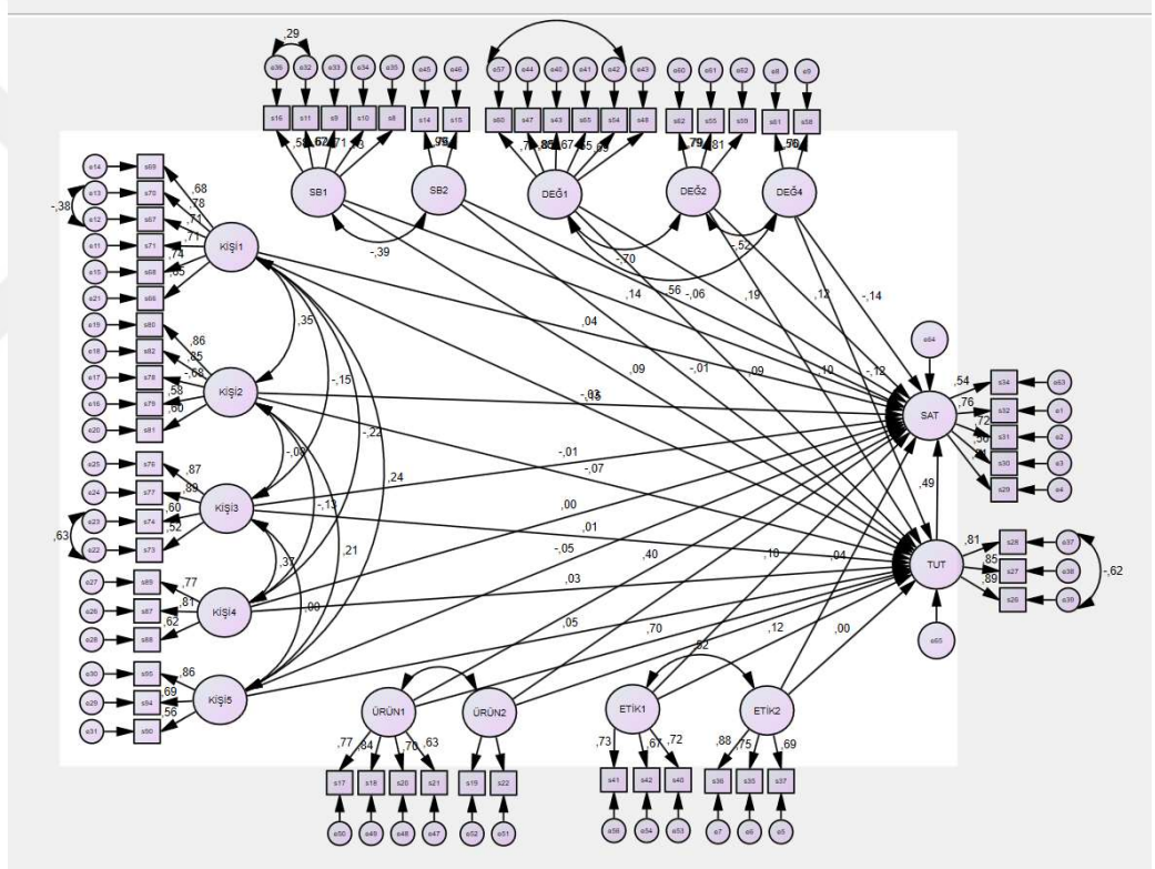
Şekil 13: Yapısal Eşitlik Araştırma Modeli (Revize Model)
