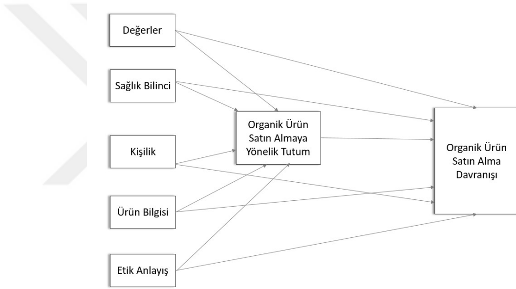
Şekil 4: Araştırma Modeli
