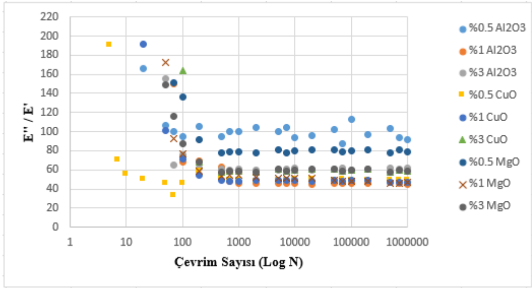
Şekil 4.24. KM-3 katman yapısında %0.5-%1-%3 ( \text{Al}_2\text{O}_3 , CuO ve MgO) nanopartikül takviyeli kompozit malzemelerin E''/E' – Çevrim Sayısı (Log N) karşılaştırmalı grafiği
