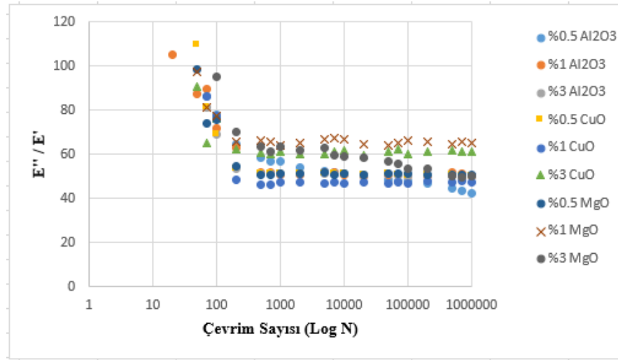
Şekil 4.22. KM-1 katman yapısında %0.5-%1-%3 ( \text{Al}_2\text{O}_3 , CuO ve MgO) nanopartikül takviyeli kompozit malzemelerin E''/E' – Çevrim Sayısı (Log N) karşılaştırmalı grafiği
