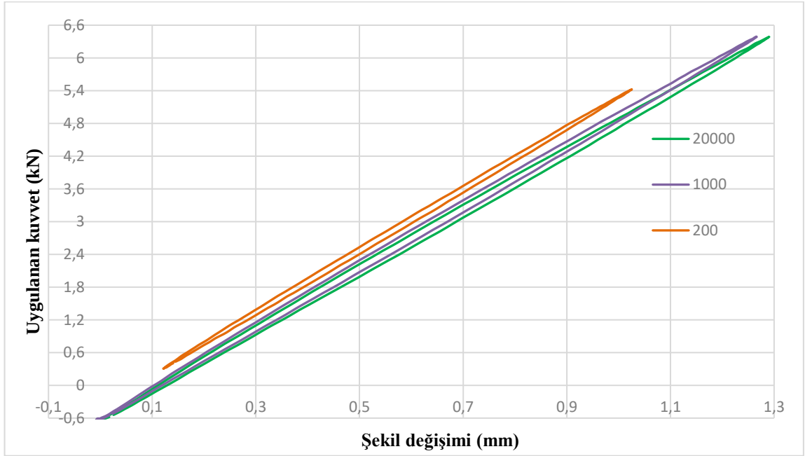
Şekil 4.42. KM-2 katman yapısında %1 MgO nanopartikül takviyeli kompozit malzemelerin farklı çevrim sayılarında karşılaştırmalı histerezis eğrileri
