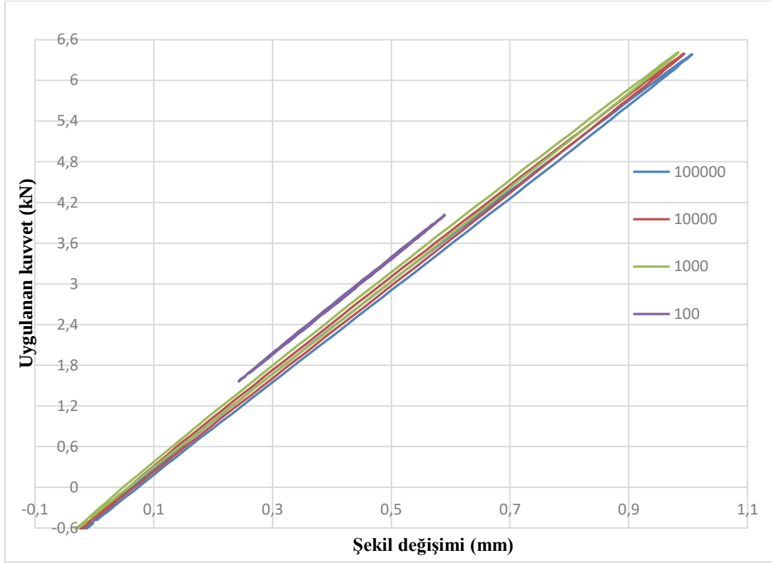
Şekil 4.50. KM-3 katman yapısında %1 \text{Al}_2\text{O}_3 nanopartikül takviyeli kompozit malzemelerin farklı çevrim sayılarında karşılaştırmalı histerezis eğrileri
