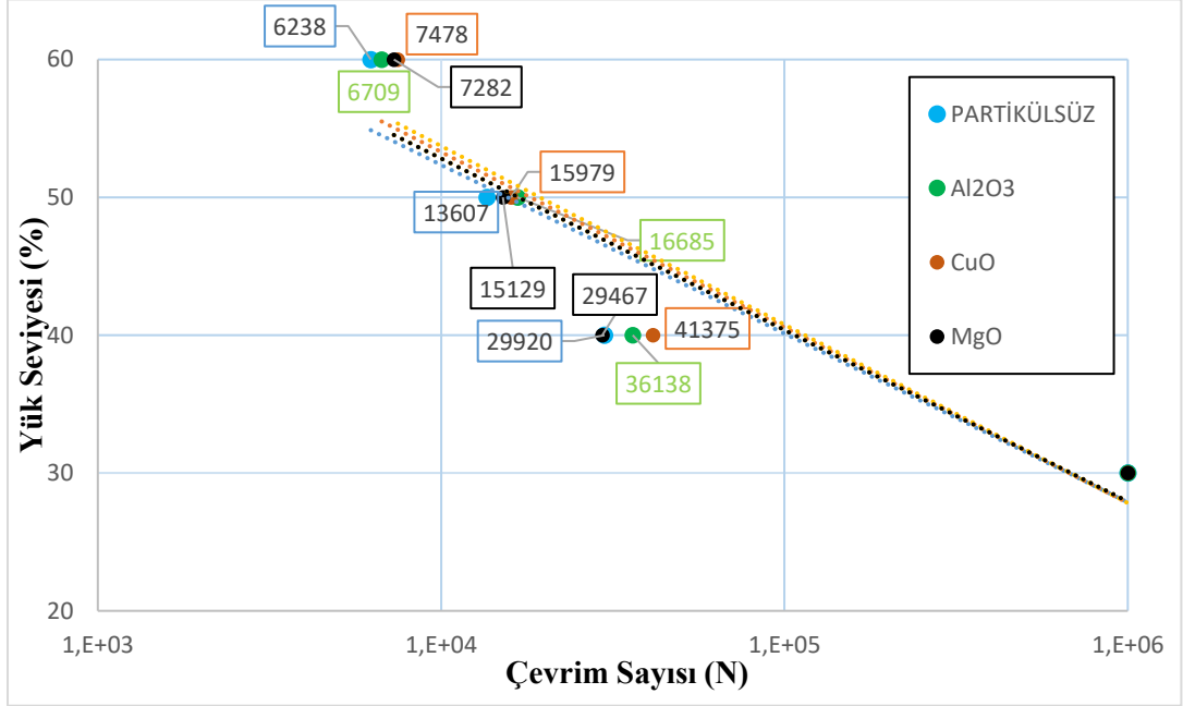
Şekil 4.10. KM-4 katman yapısında takviyesiz ve %3 Al 2 O 3 , CuO ve MgO nanopartikül takviyeli kompozit malzemelerin Yük Seviyesi (%) – Çevrim Sayısı (N) karşılaştırmalı grafiği
