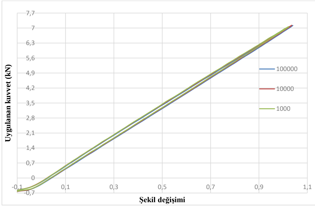
Şekil 4.48. KM-3 katman yapısında %0.5 Al 2 O 3 nanopartikül takviyeli kompozit malzemelerin farklı çevrim sayılarında karşılaştırmalı histerezis eğrileri
