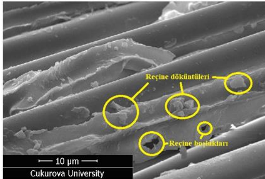
Şekil 4.58. \text{Al}_2\text{O}_3 nanopartikül takviyeli kompozit malzemelerde fiber yüzeyleri hasar mekanizmaları
