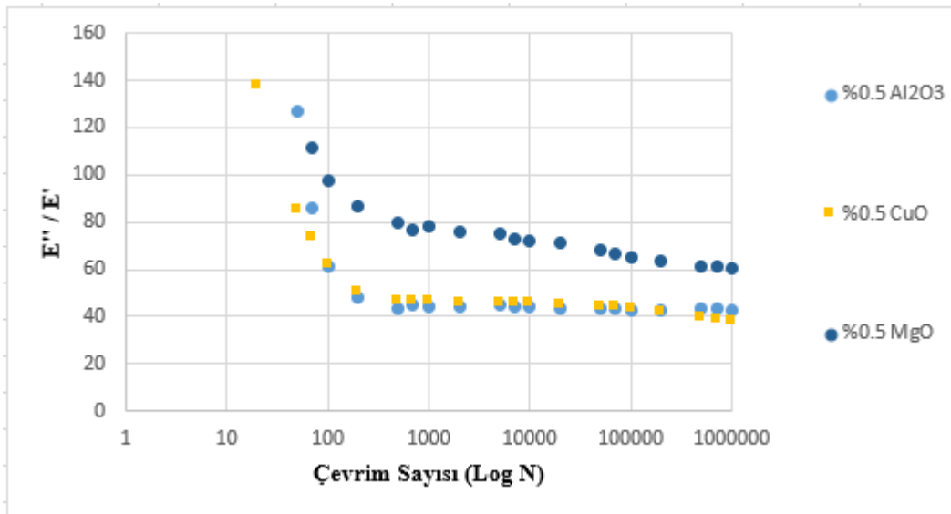
Şekil 4.32. KM-4 katman yapısında %0.5 \text{Al}_2\text{O}_3 , CuO ve MgO nanopartikül takviyeli kompozit malzemelerin E''/E' – Çevrim Sayısı (Log N) karşılaştırmalı grafiği
