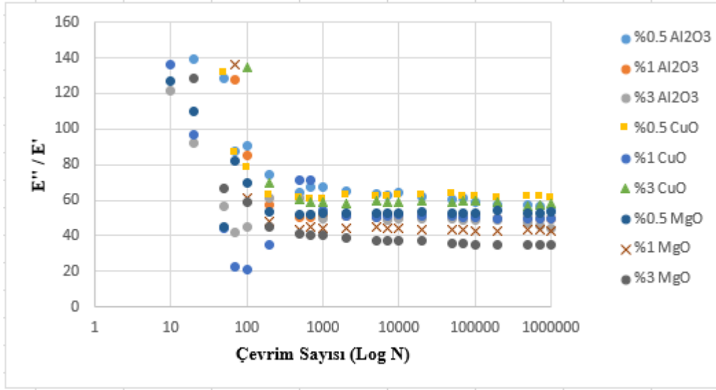
Şekil 4.26. KM-5 katman yapısında %0.5-%1-%3 ( \text{Al}_2\text{O}_3 , CuO ve MgO) nanopartikül takviyeli kompozit malzemelerin E''/E' – Çevrim Sayısı (Log N) karşılaştırmalı grafiği
