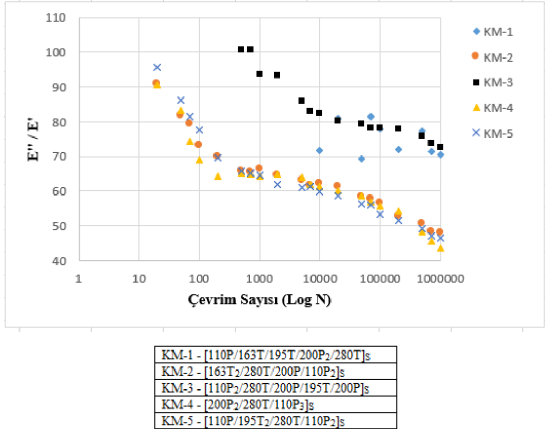
Şekil 4.12. Farklı katman yapılarında nanopartikül takviyesiz kompozit malzemelerin E''/E' – Çevrim Sayısı (Log N) karşılaştırmalı grafiği
