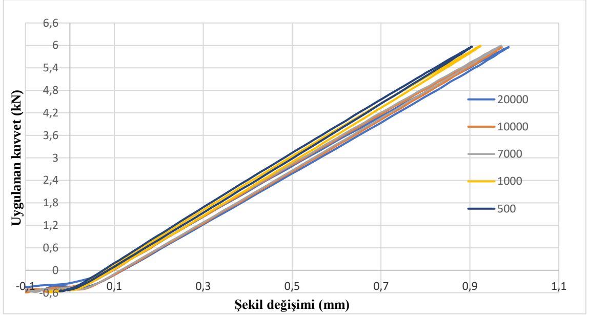
Şekil 4.35. KM-5 katman yapısında nanopartikül takviyesiz kompozit malzemelerin farklı çevrim sayılarında karşılaştırmalı histerezis eğrileri
