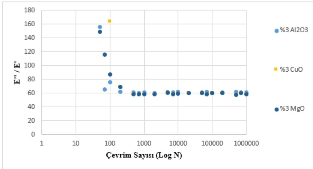
Şekil 4.31. KM-3 katman yapısında %3 \text{Al}_2\text{O}_3 , CuO ve MgO nanopartikül takviyeli kompozit malzemelerin E''/E' – Çevrim Sayısı (Log N) karşılaştırmalı grafiği
