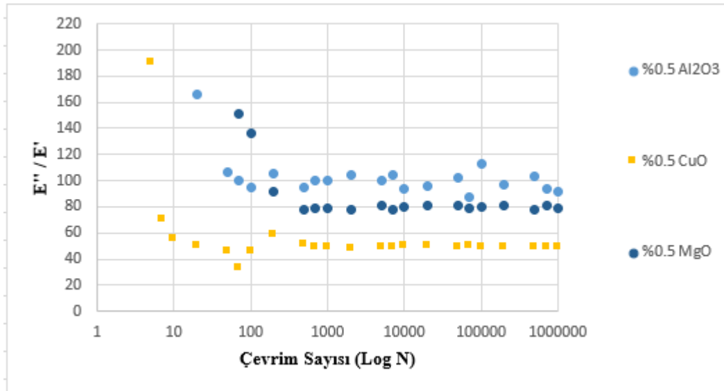
Şekil 4.29. KM-3 katman yapısında %0.5 \text{Al}_2\text{O}_3 , CuO ve MgO nanopartikül takviyeli kompozit malzemelerin E''/E' – Çevrim Sayısı (Log N) karşılaştırmalı grafiği
