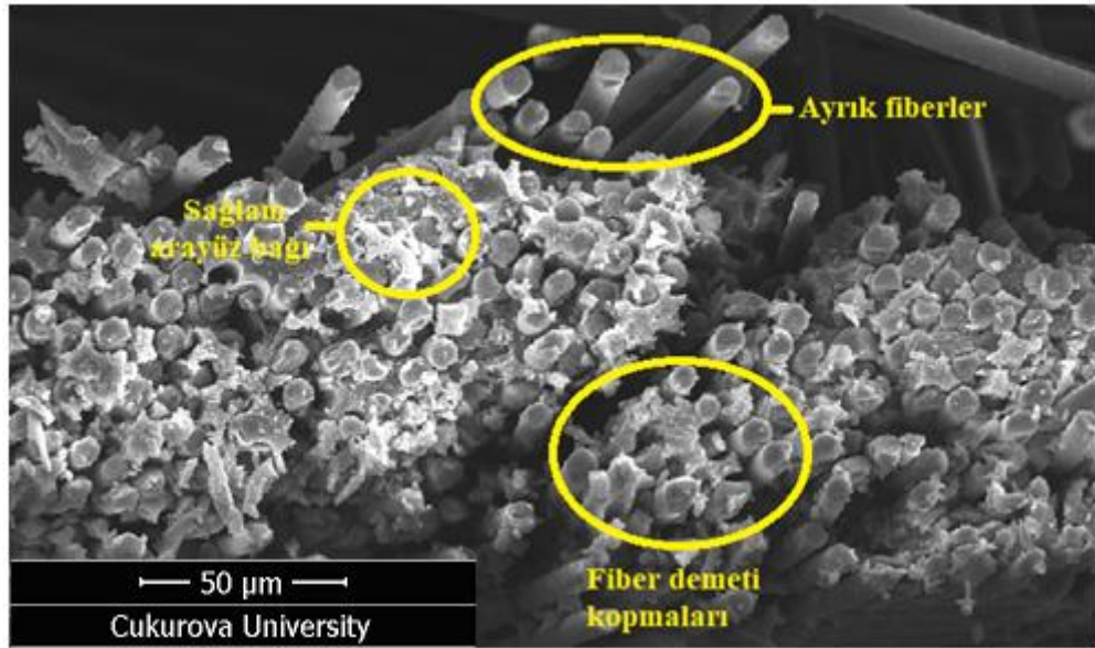
Şekil 4.64. CuO nanopartikül takviyeli kompozit malzemelerde fiber hasar mekanizmaları
