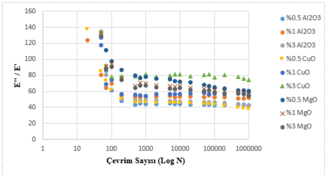
Şekil 4.25. KM-4 katman yapısında %0.5-%1-%3 ( \text{Al}_2\text{O}_3 , CuO ve MgO) nanopartikül takviyeli kompozit malzemelerin E''/E' – Çevrim Sayısı (Log N) karşılaştırmalı grafiği
