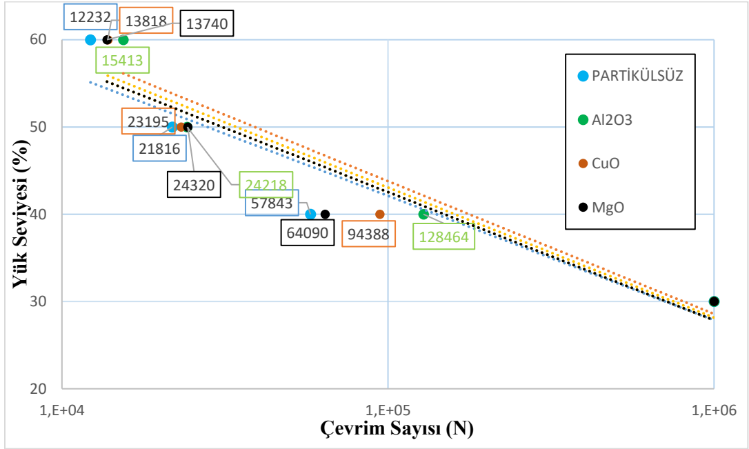
Şekil 4.9. KM-3 katman yapısında takviyesiz ve %1 \text{Al}_2\text{O}_3 , CuO ve MgO nanopartikül takviyeli kompozit malzemelerin Yük Seviyesi (%) – Çevrim Sayısı (N) karşılaştırmalı grafiği
