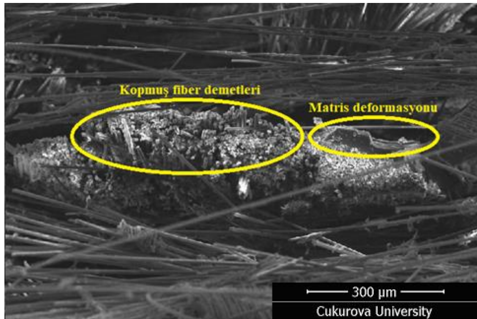
Şekil 4.60. \text{Al}_2\text{O}_3 nanopartikül takviyeli kompozit malzemelerde fiber demetlerinin matris hasar mekanizmasına etkisi
