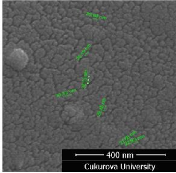
Şekil 4.57. SEM analizi ile elde edilen \text{Al}_2\text{O}_3 nanopartikül boyutları
