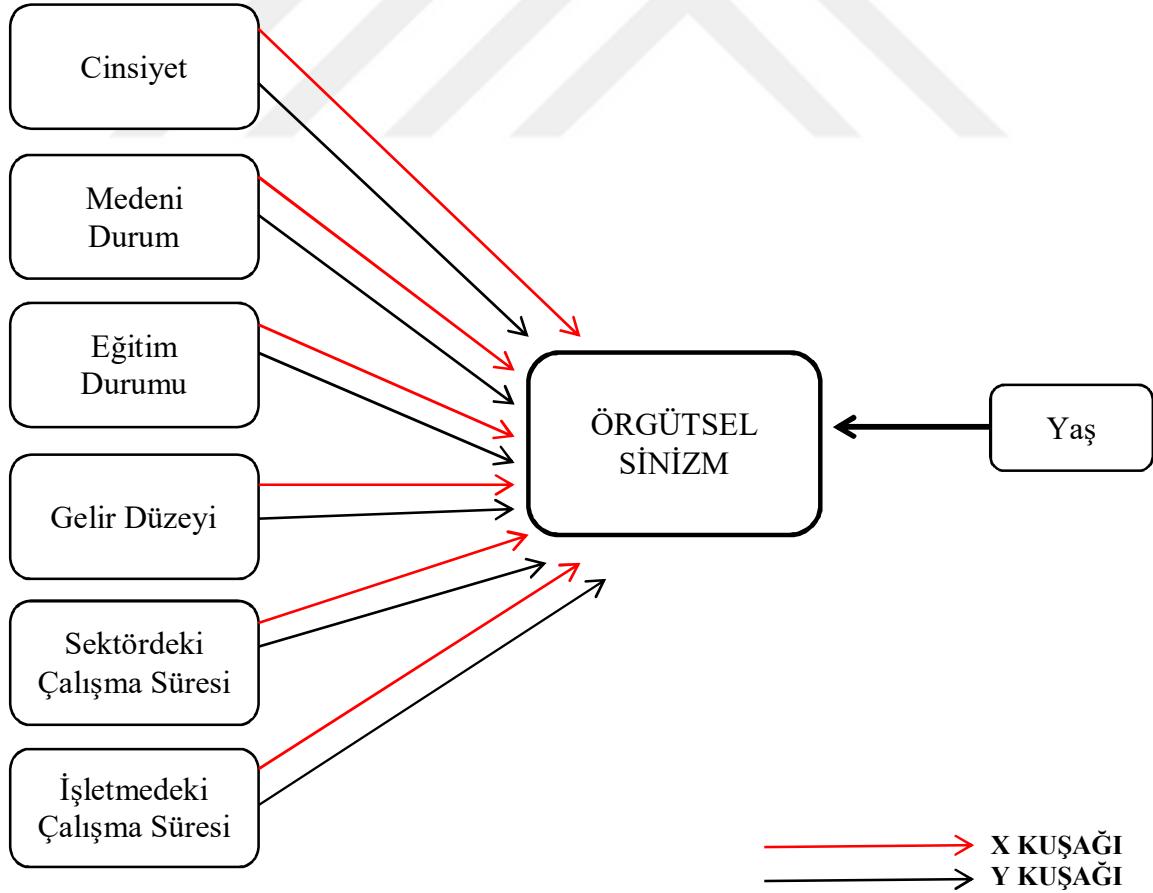
Şekil 3.3 Araştırmanın Modeli
